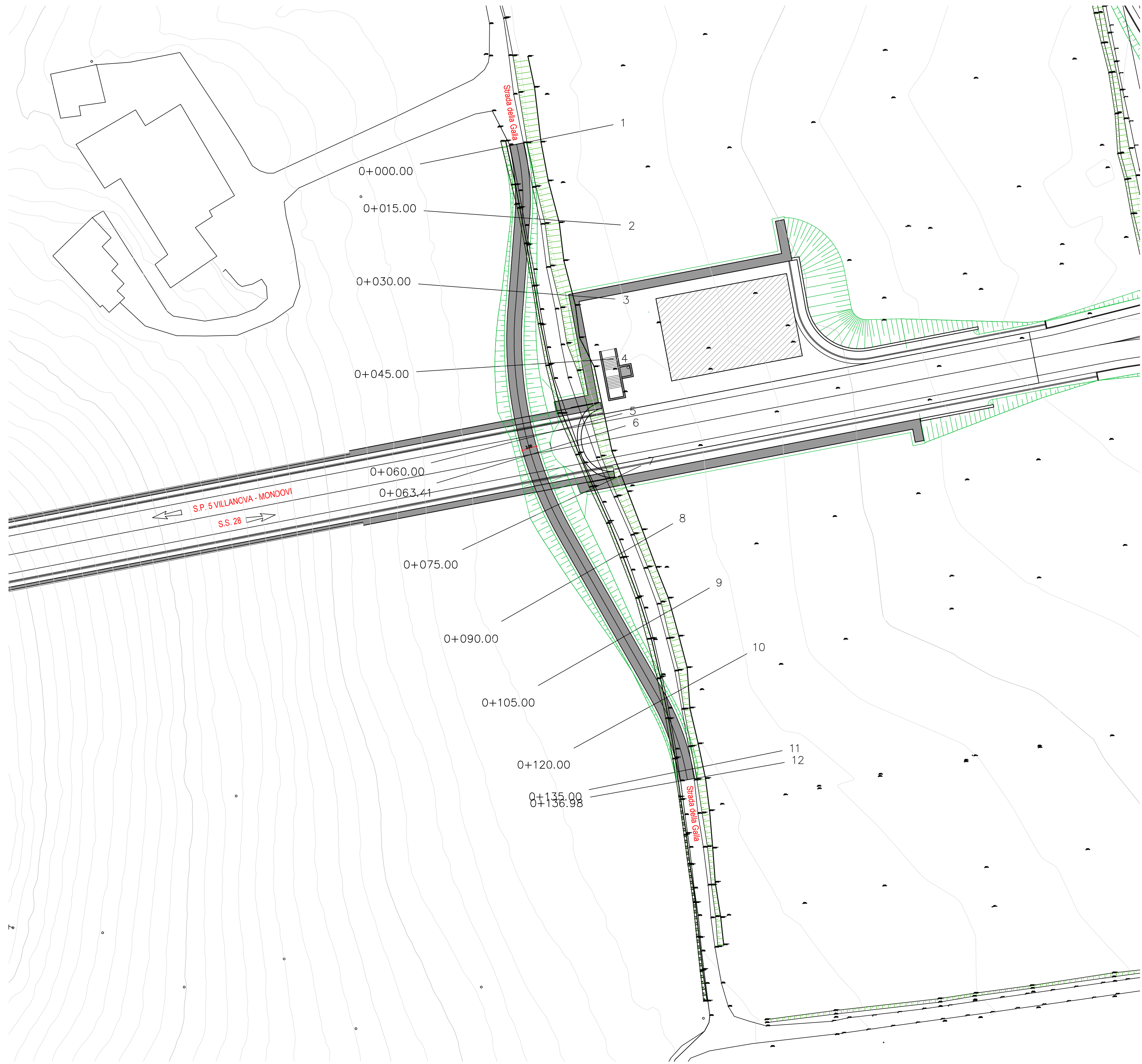
Planimetria di tracciamento Scala 1:500
