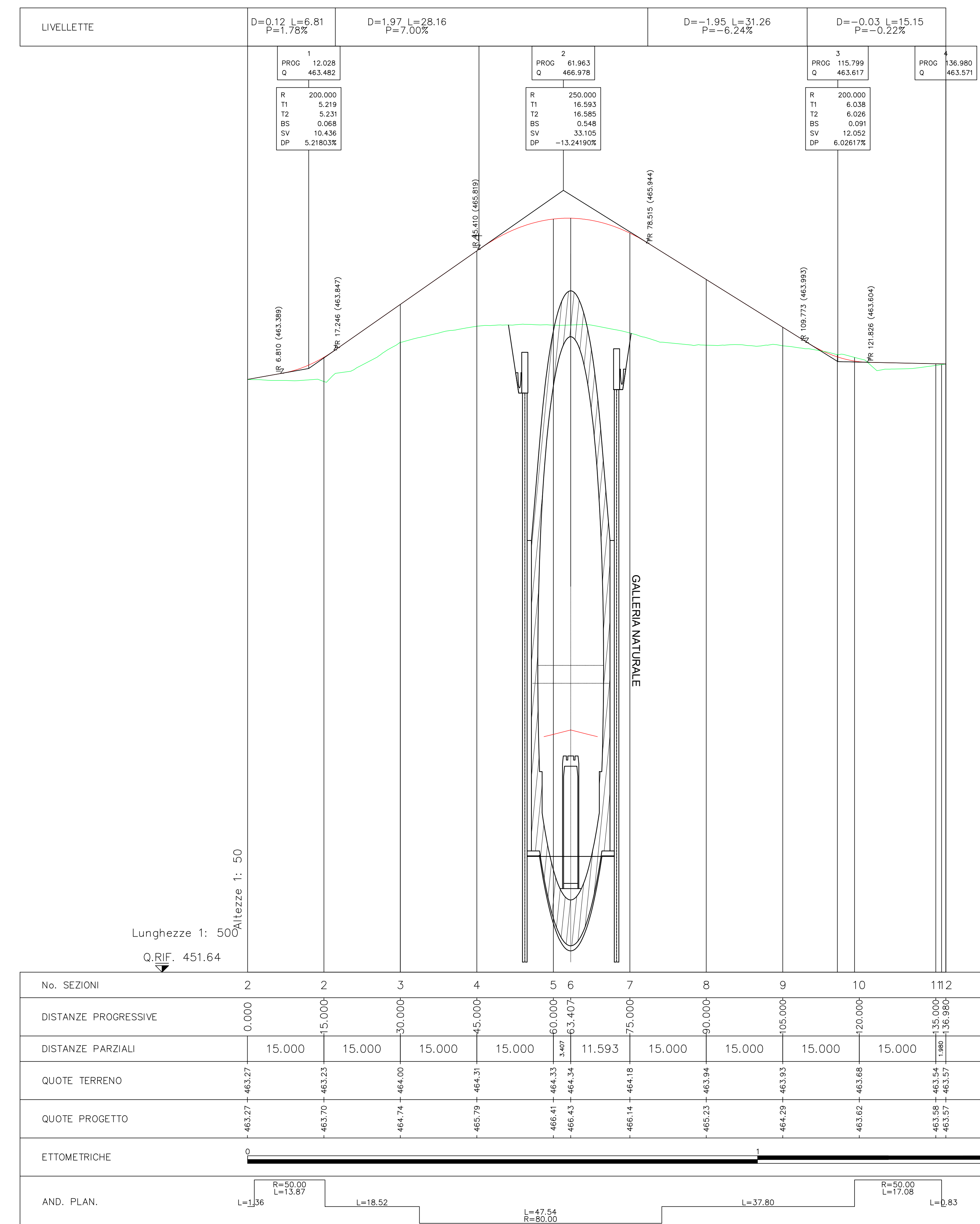
Profilo di progetto Scala 1:500 / 1:50
