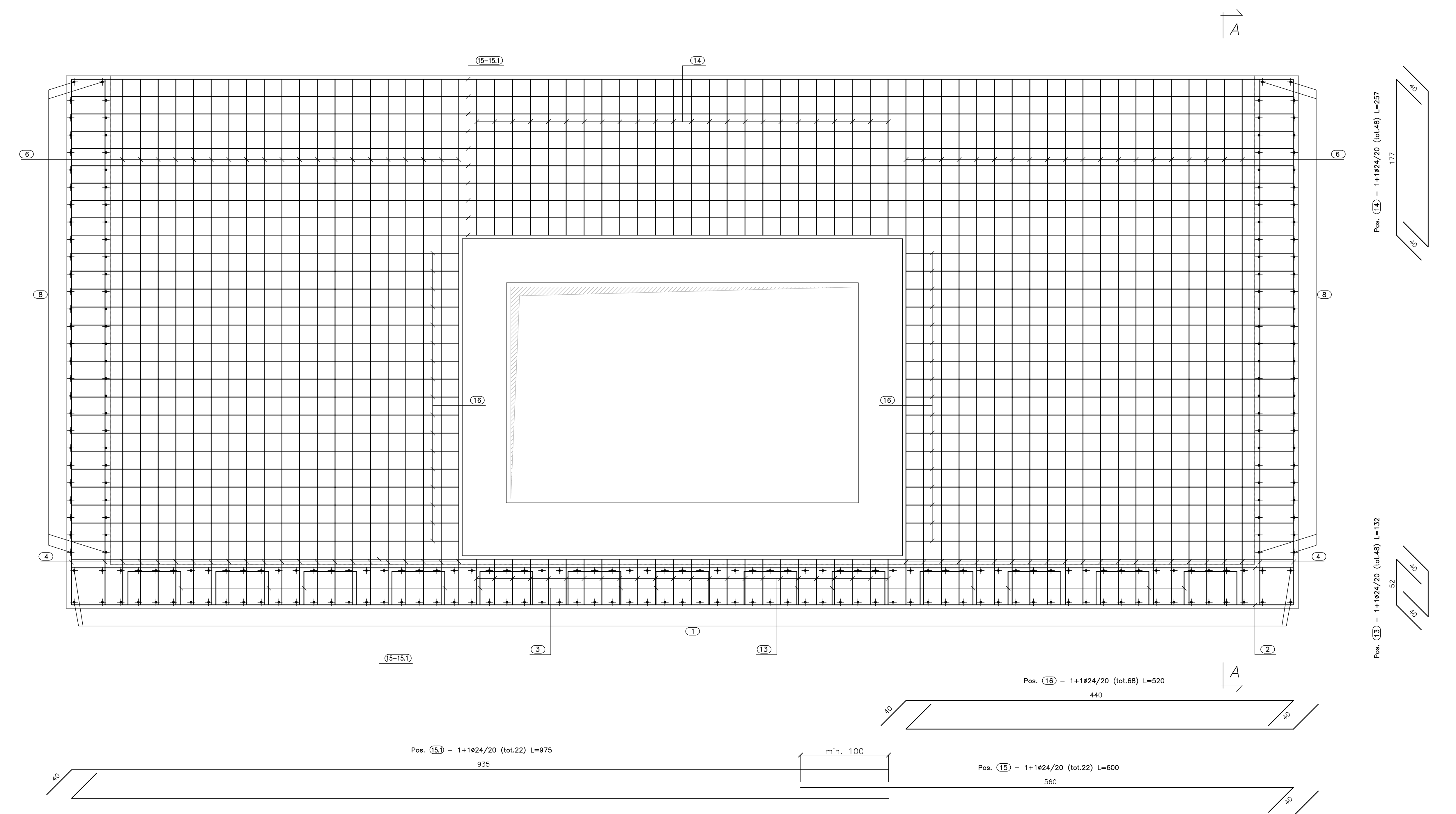
VISTA. C-C (SCALA 1:25)
