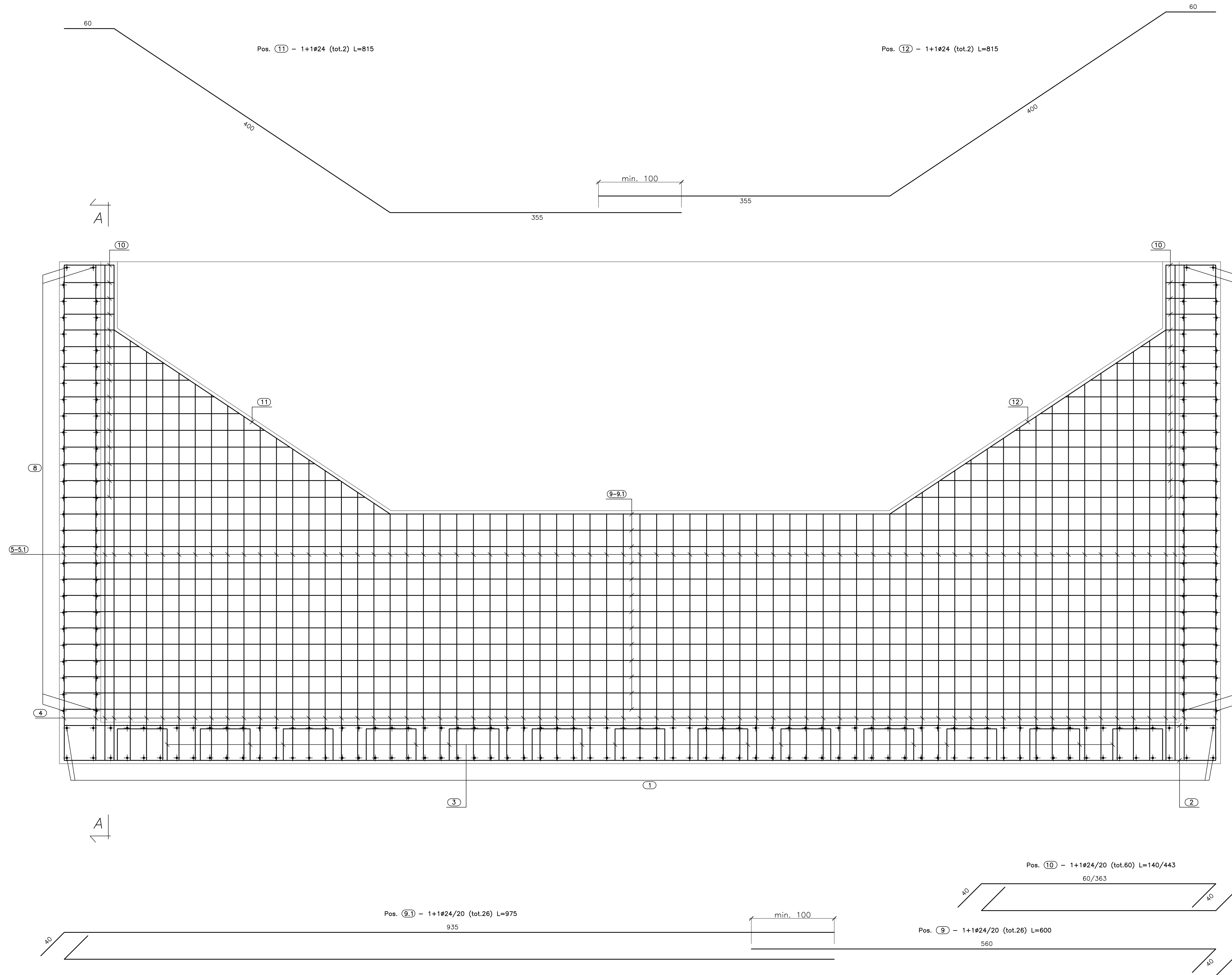
VISTA. B-B (SCALA 1:25)
