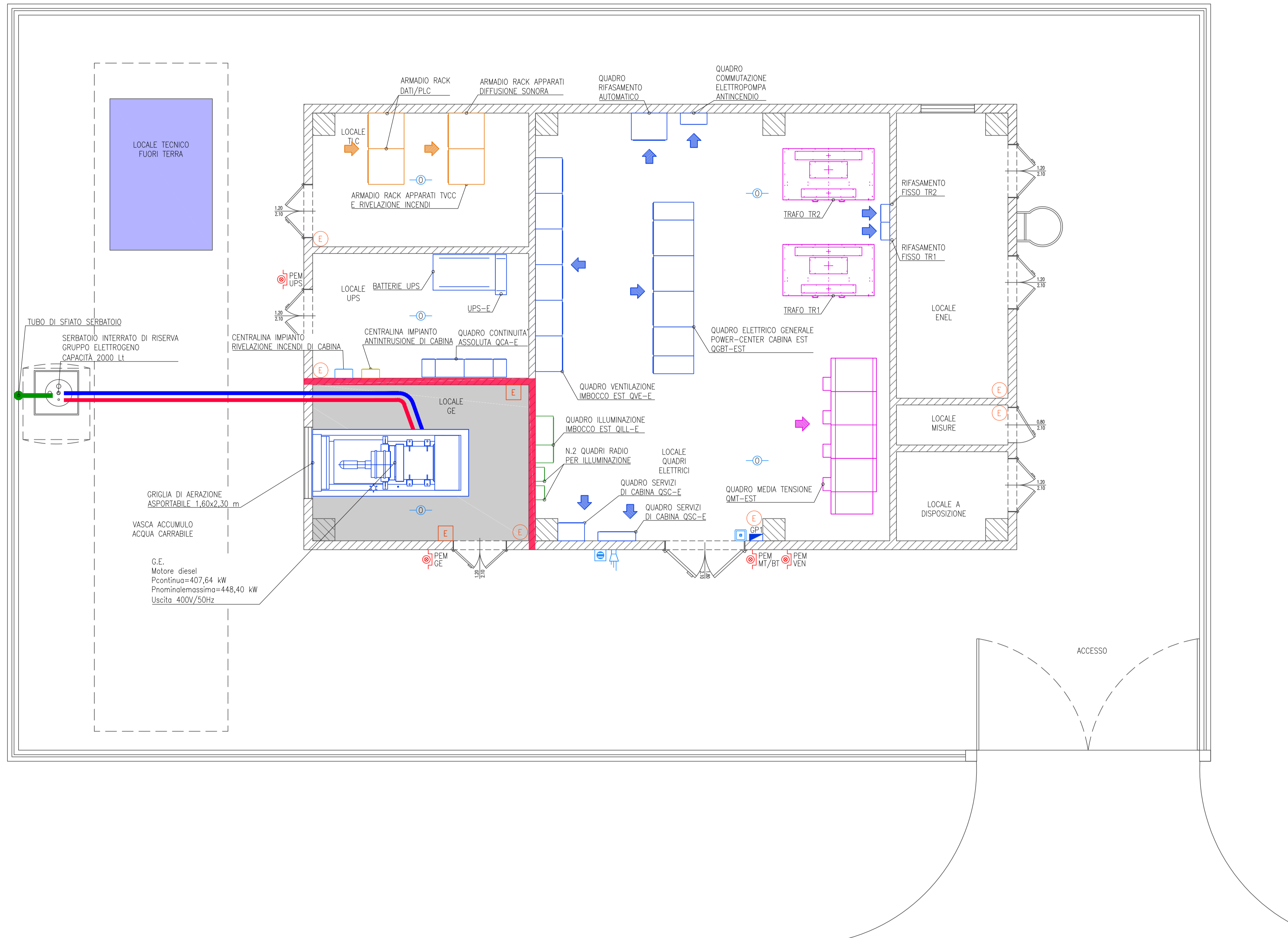
Cabina elettrica Est Pianta con ubicazione attrezzature antincendio Scala 1:50
