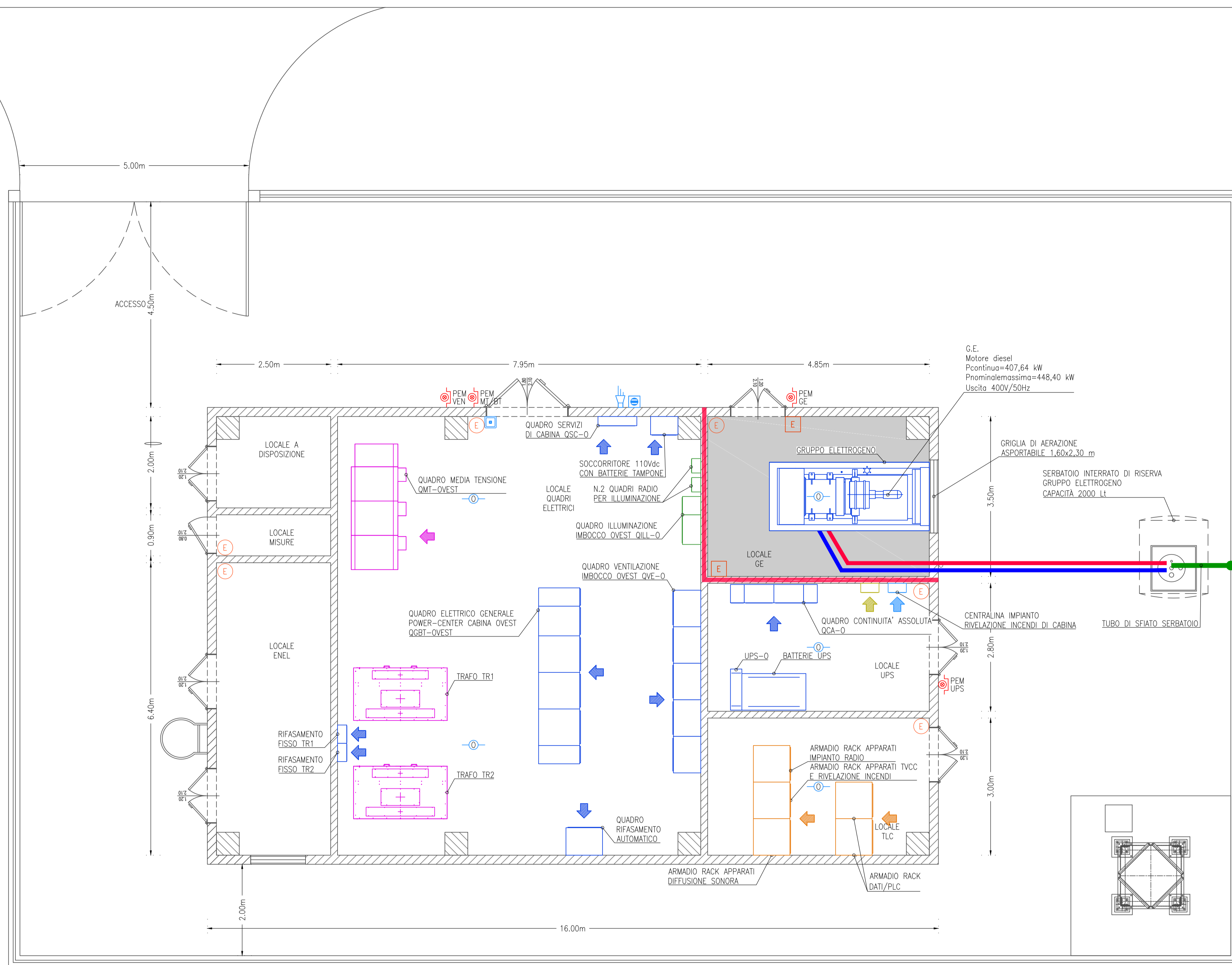
Cabina elettrica Ovest Pianta con ubicazione attrezzature antincendio Scala 1:50
