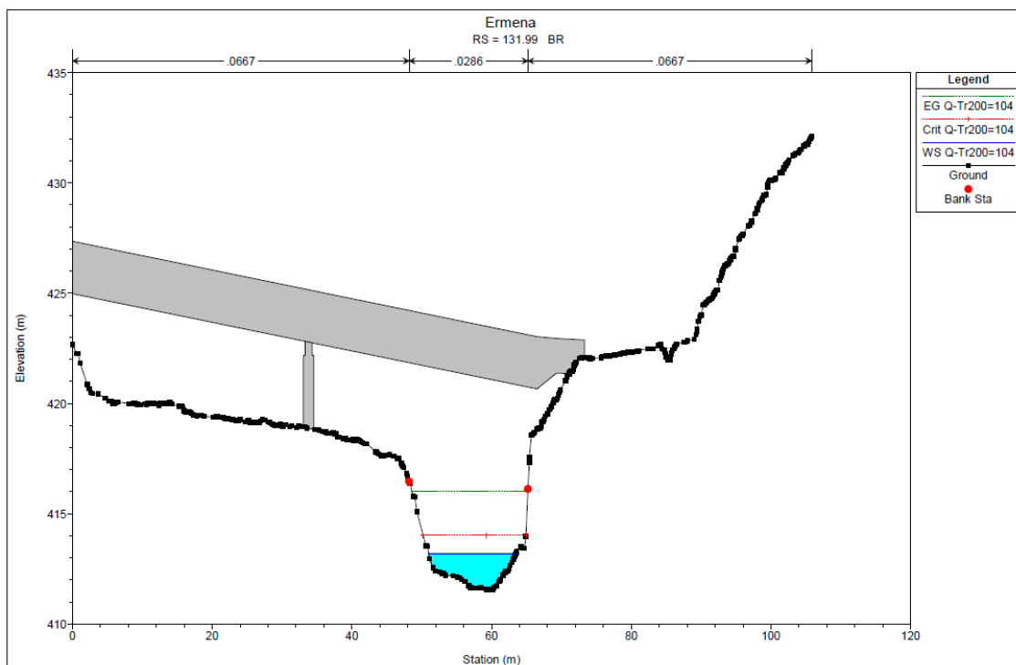
Figura 3.11 Livello idrico nella sezione del viadotto pari a 413,36 m slm con Q_{Tr200} . (dalla relazione idraulica di progetto)
