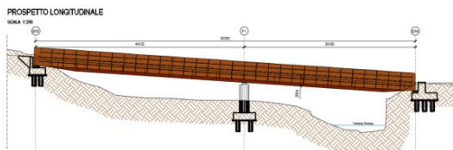
Figura 3.8 Sezione longitudinale ponte sull' Ermèna (Estratto dalla tavola di progetto P00VI02STRPF01_A)
