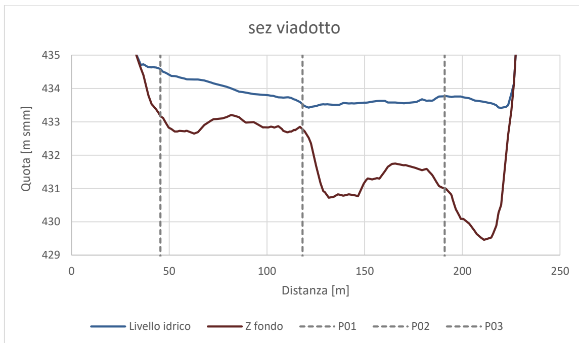
Figura 3.9: Livello idrico nella sezione del viadotto pari a 434,42 m slm con Q_{Tr200}=831 \text{ m}^3/\text{s} .
