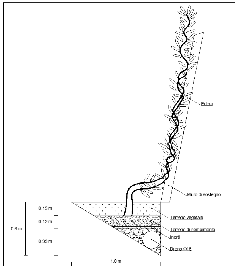
Figura 4-2 Dettaglio della posa in opera del rampicante
