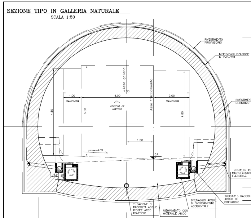
Figura 2-2 Sezione tipo galleria nuova realizzazione
