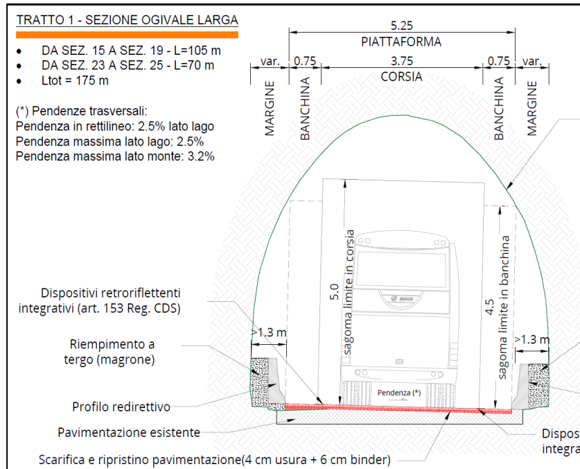
Figura 2-3 Sezione tipo adeguamento galleria esistenti
