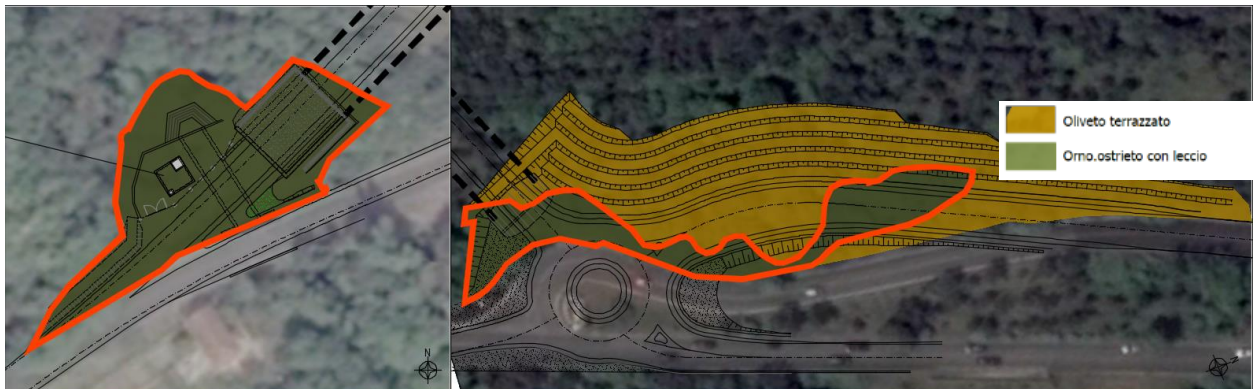
Figura 4-10 Rappresentazione aree taglio boschi
