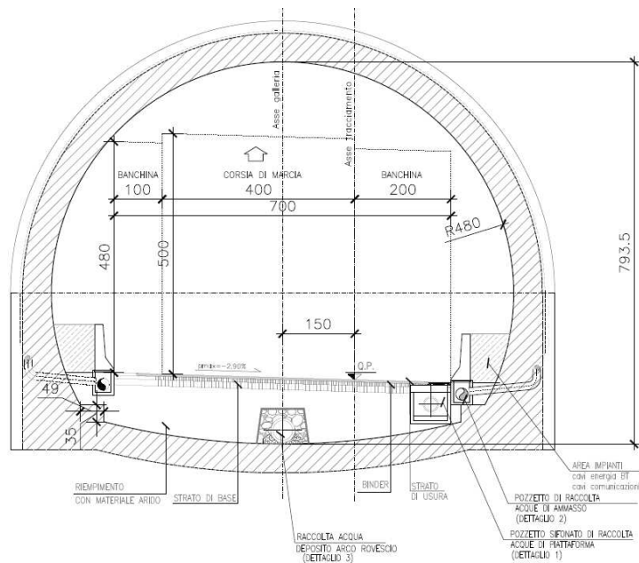
Figura 4: sezione tipo della galleria a senso unico in direzione Brescia
