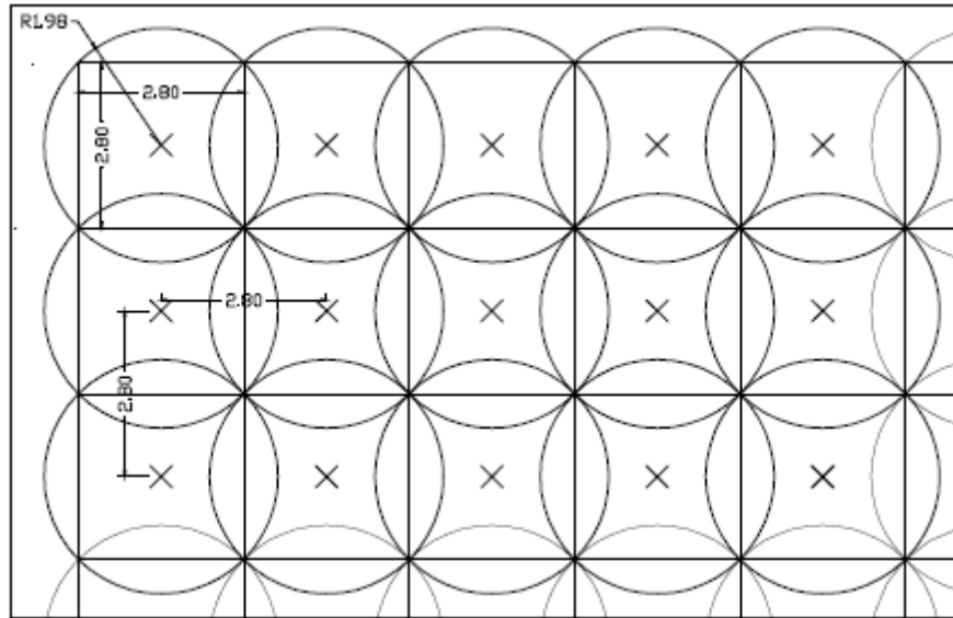
Maglia di perforazione tipo per Bonifica bellica.
