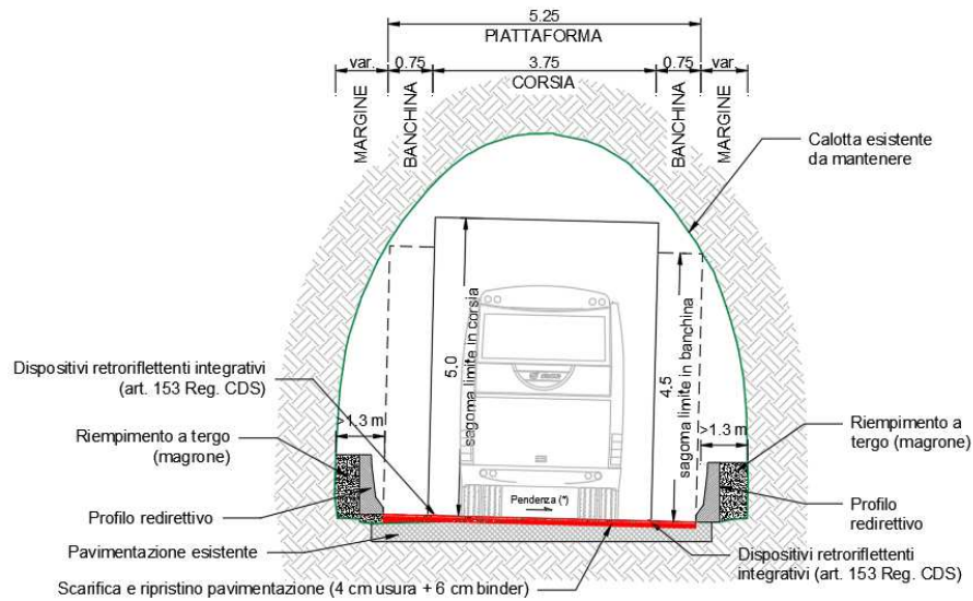
Figura 2: sezione ogivale larga nella galleria D'Acli
