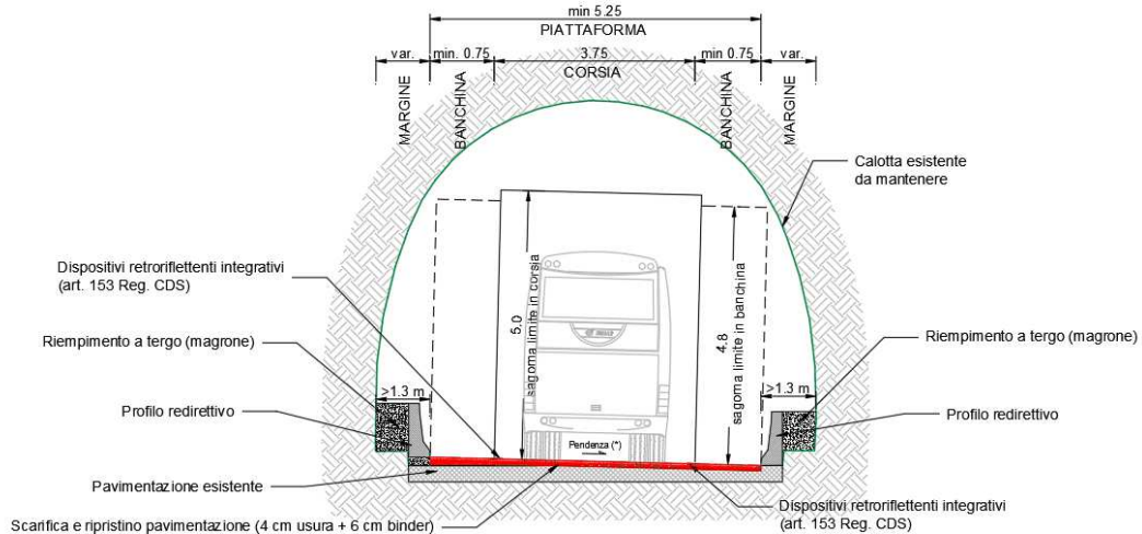
Figura 3: sezione tipo larga nella galleria Dei Ciclopi
