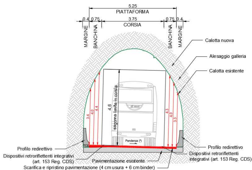
Figura 1: sezione ogivale stretta
