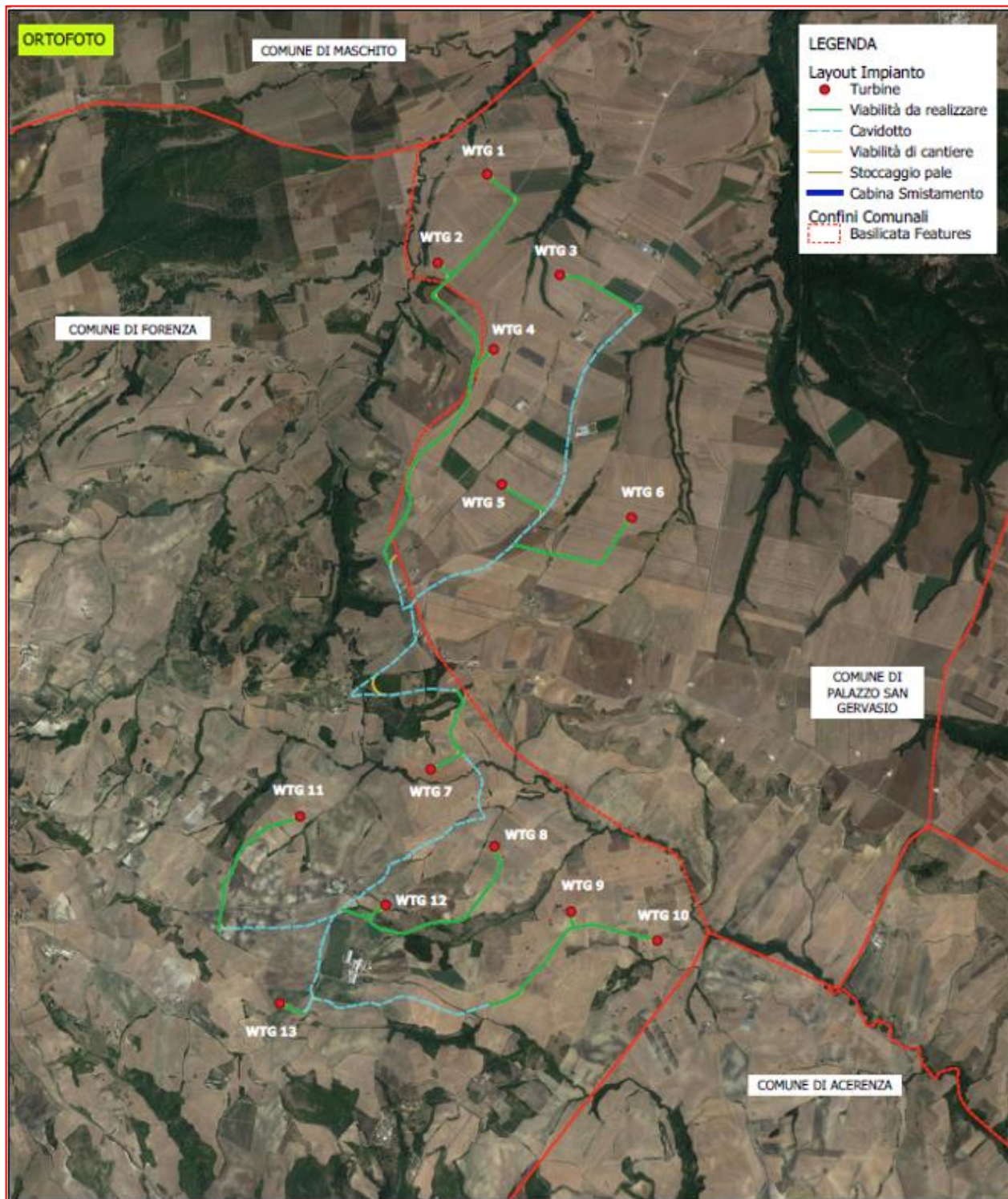
Figura 2-3: Area di intervento: dettaglio layout di progetto su ortofoto
