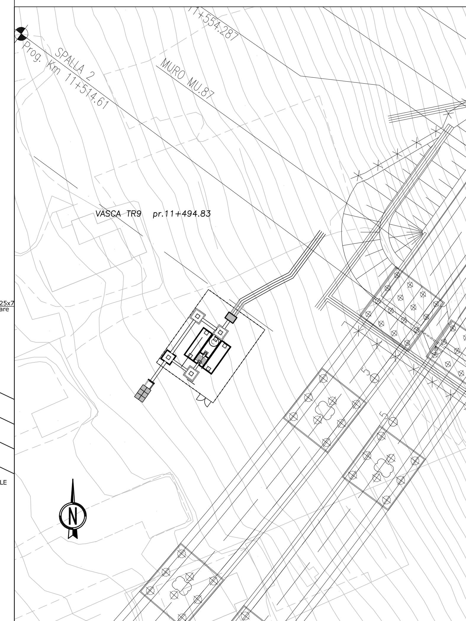
INQUADRAMENTO (SCALA 1:500)
