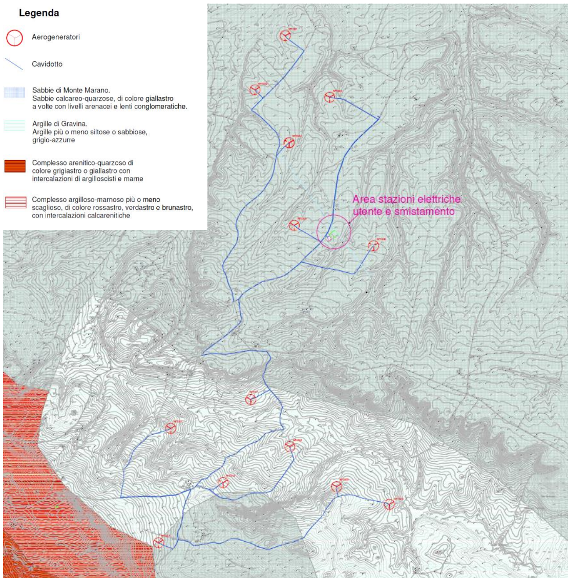
Figura f-1: Stralcio Carta Geologica
