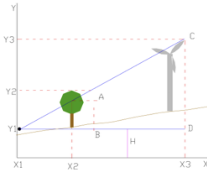
Figura 4-24: Schermatura di una turbina eolica
