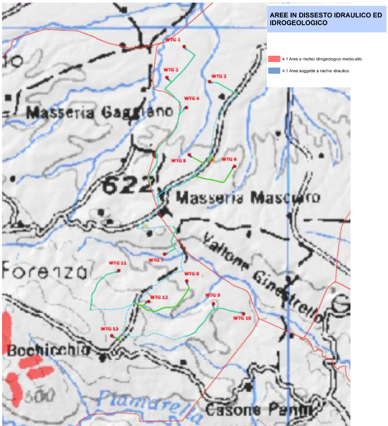
Figura 2-39: Stralcio carta delle aree in dissesto idraulico ed idrogeologico
