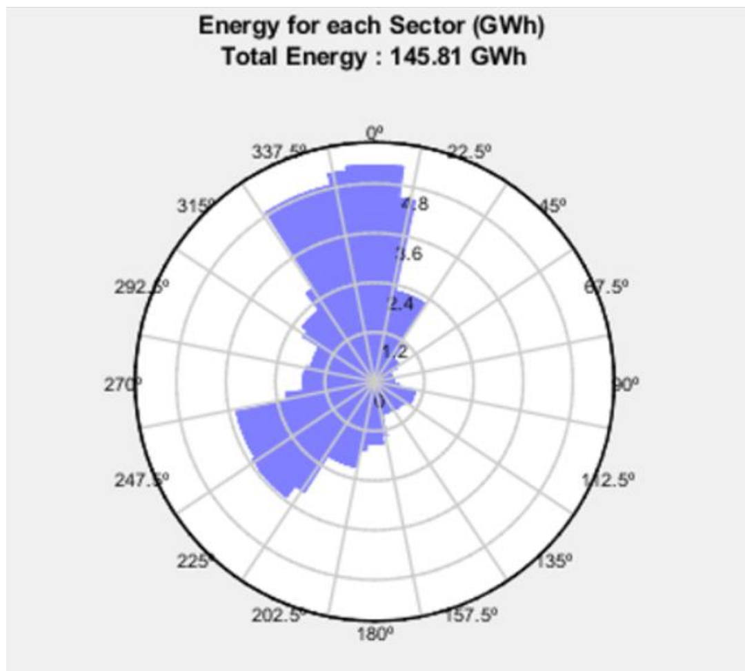
Figura 3-2: Rosa dei venti di produzione eolica del progetto CE PALAZZO.
