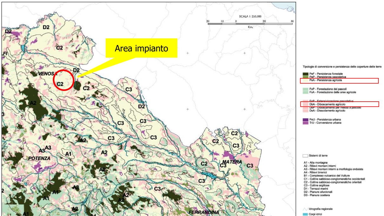
Figura 2-15: Stralcio Tavola B1: Carta delle dinamiche delle coperture delle terre
