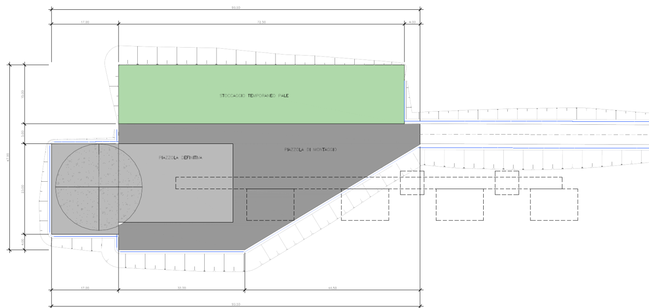
Figura 3-9: Piazzola tipo e viabilità di accesso
