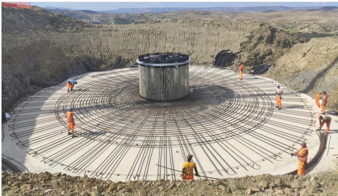
Figura 3-5: immagine tipo posa anchor cages
