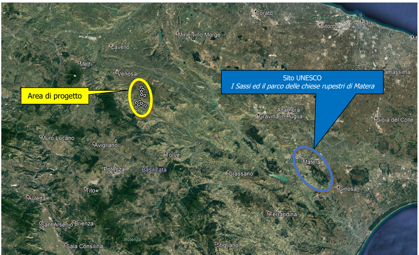
Figura 2-29: Perimetrazione sito UNESCO I Sassi ed il parco delle chiese rupestri di Matera e layout di progetto
