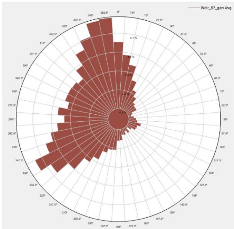
Figura 3-1: Rosa dei venti del progetto CE PALAZZO.
