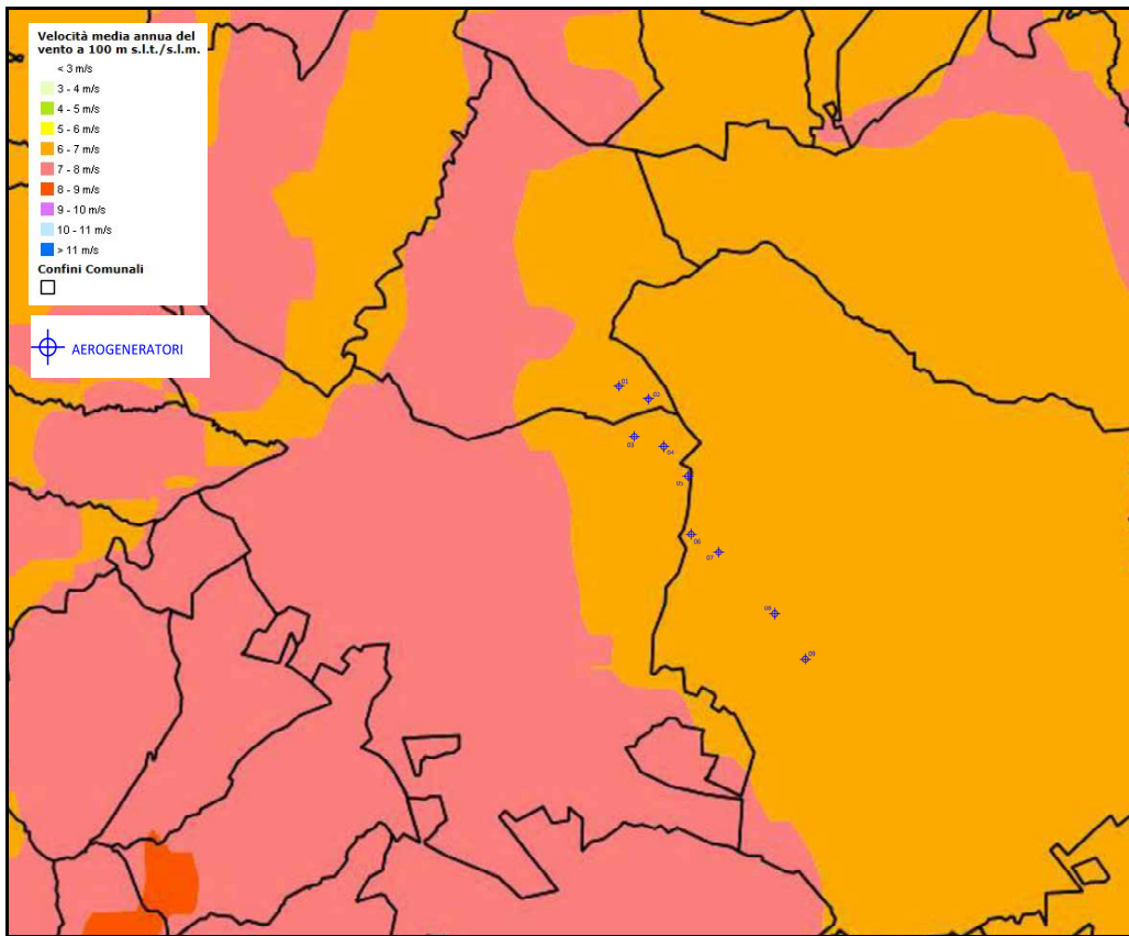
Impianto su Atlante eolico interattivo con velocità media annua del vento a 100 m s.l.m.
