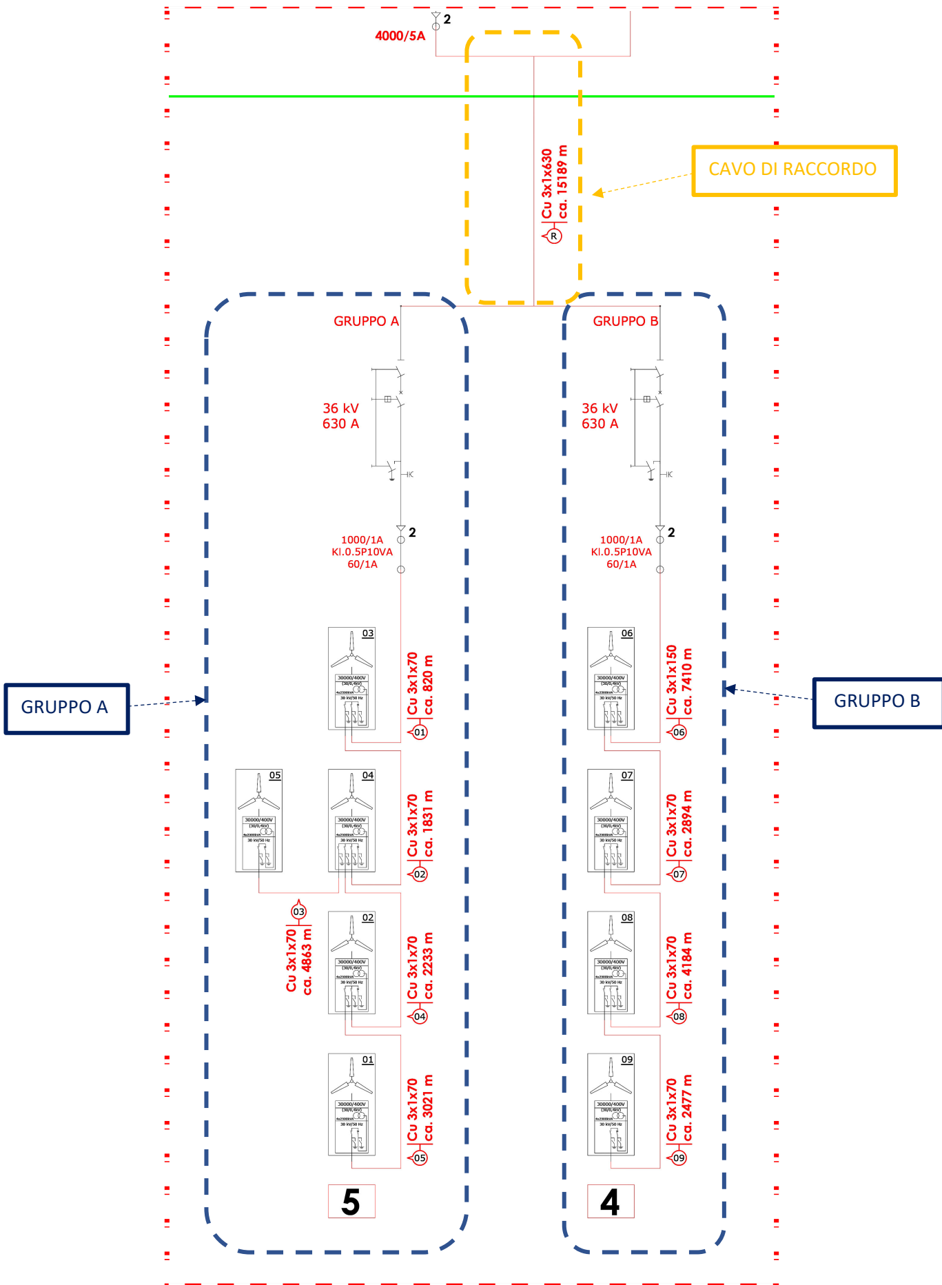
Dettaglio Gruppi schema elettrico unifilare
