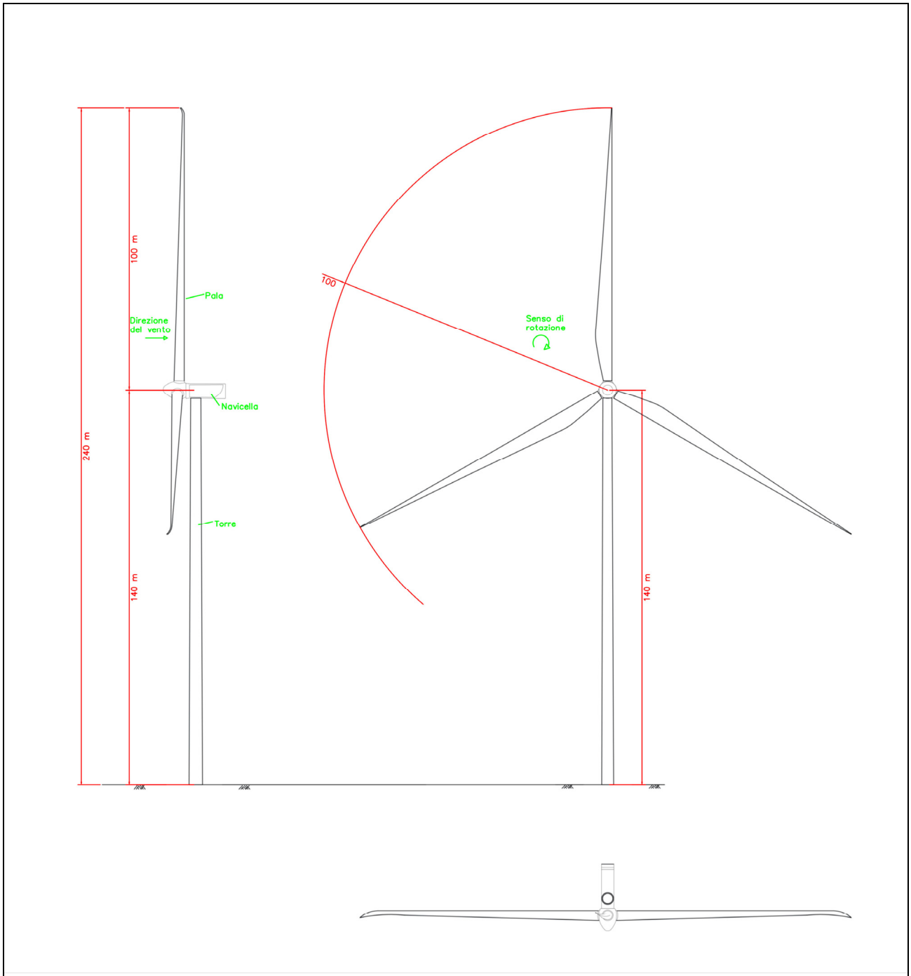
Aerogeneratore tipo: pianta, prospetto frontale e prospetto laterale
