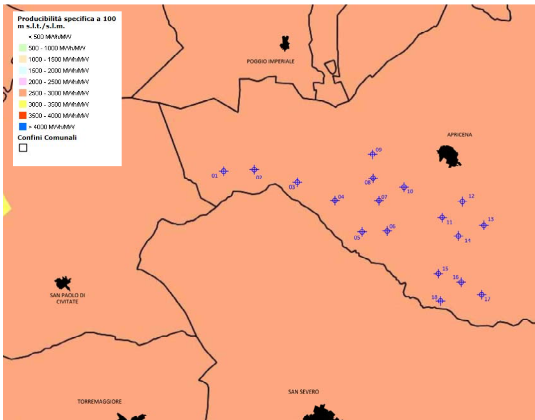
Impianto su Atlante eolico interattivo con produttività specifica a 100 m s.l.m.
