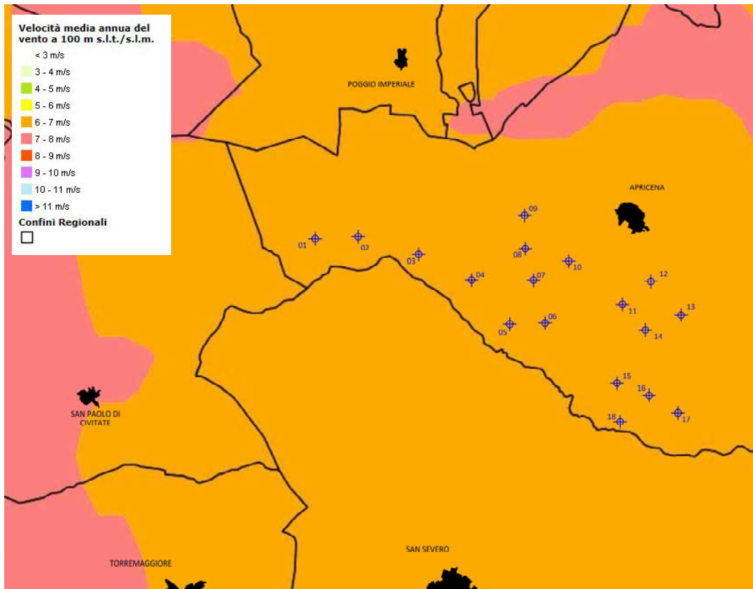
Impianto su Atlante eolico interattivo con velocità media annua del vento a 100 m s.l.m.
