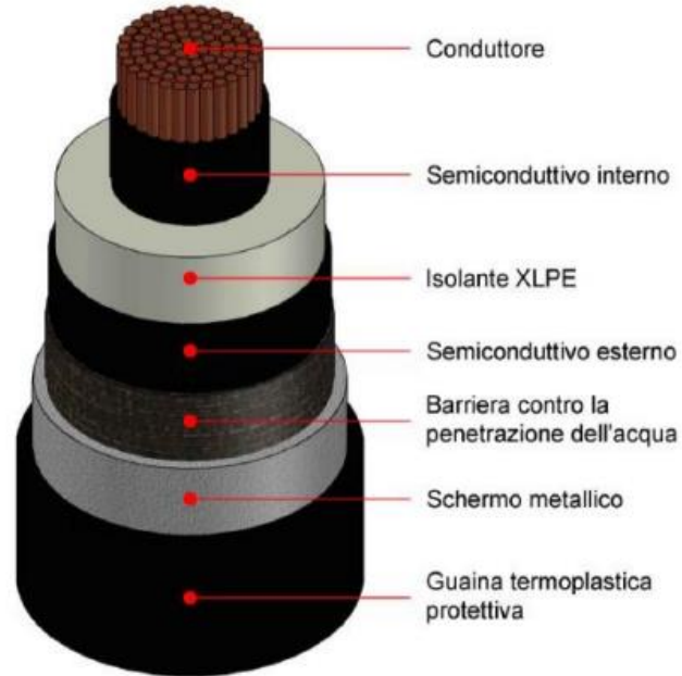
Schema costitutivo (a titolo indicativo)
