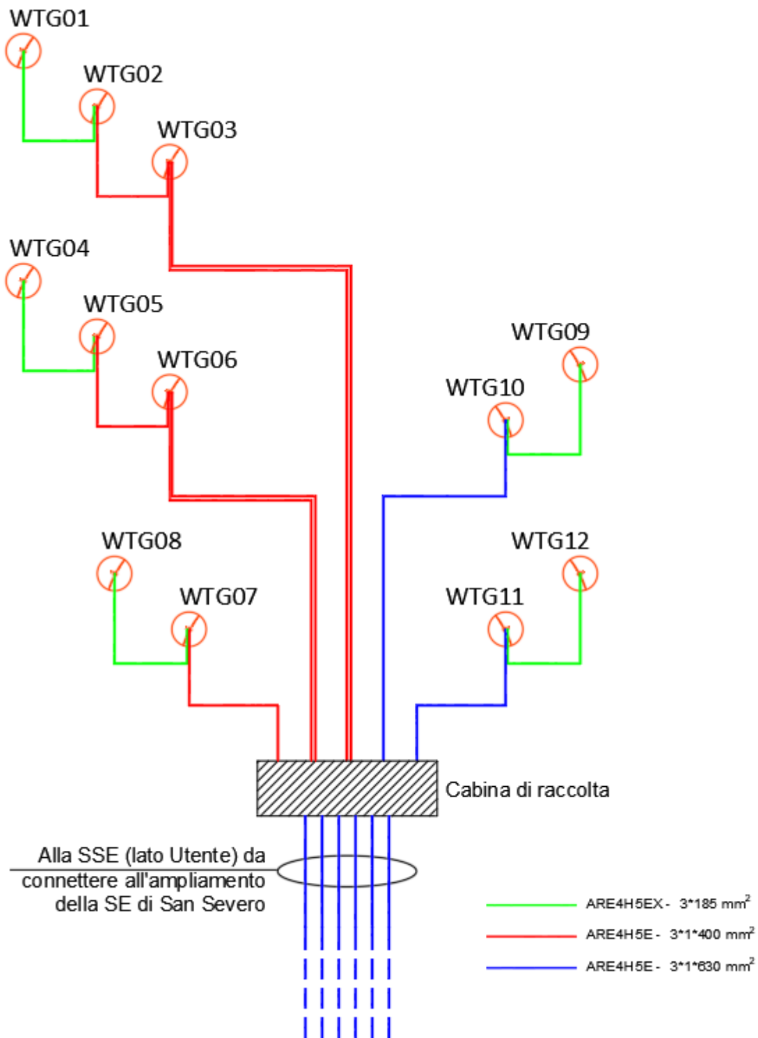
Figura 3 - Schema di connessione elettrica dell'impianto eolico in progetto
