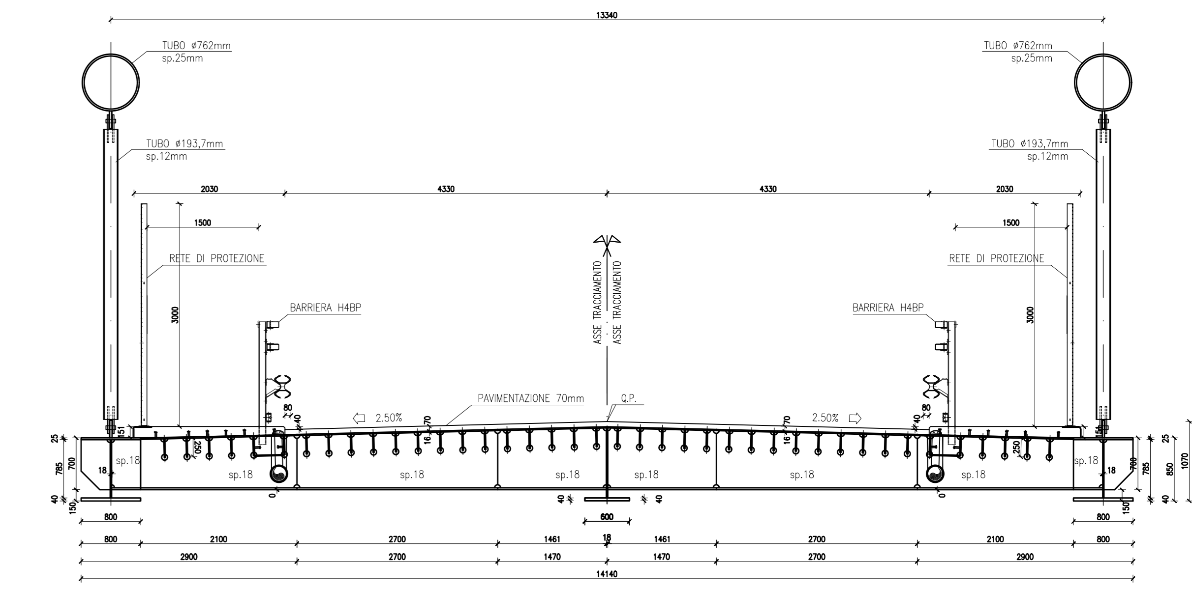
SEZIONE TRASVERSALE TIPO IN MEZZERIA SCALA 1:50
