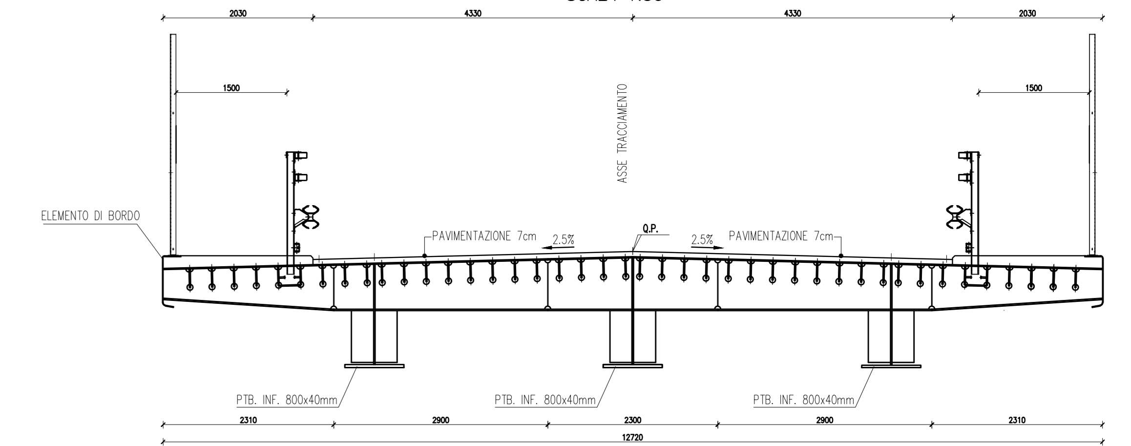
SEZIONE TRASVERSALE TIPO IN MEZZERIA SCALA 1:50
