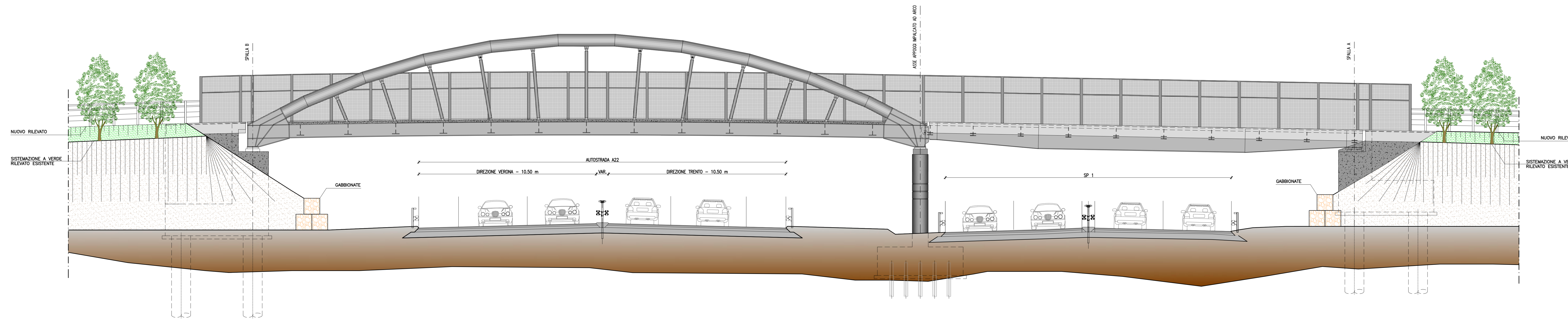
PROSPETTO LONGITUDINALE SCALA 1:100
