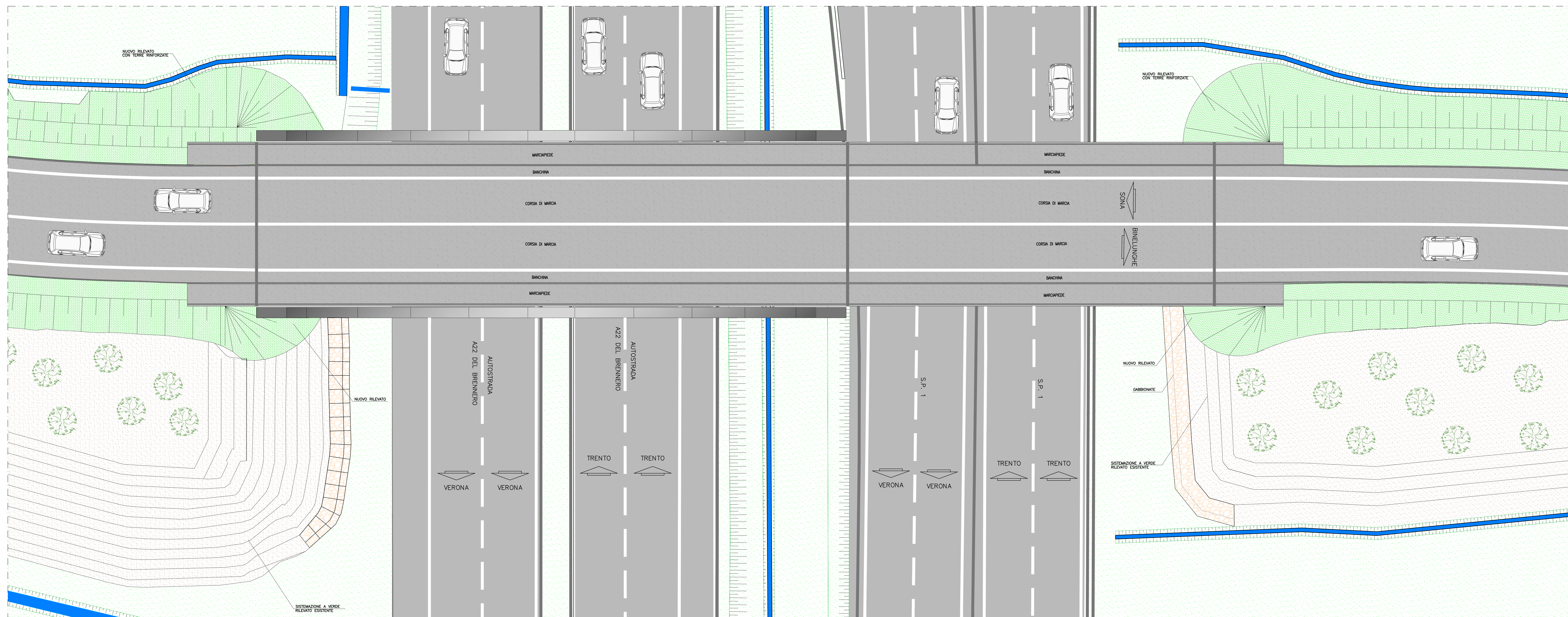
PIANTA SCALA 1:100
