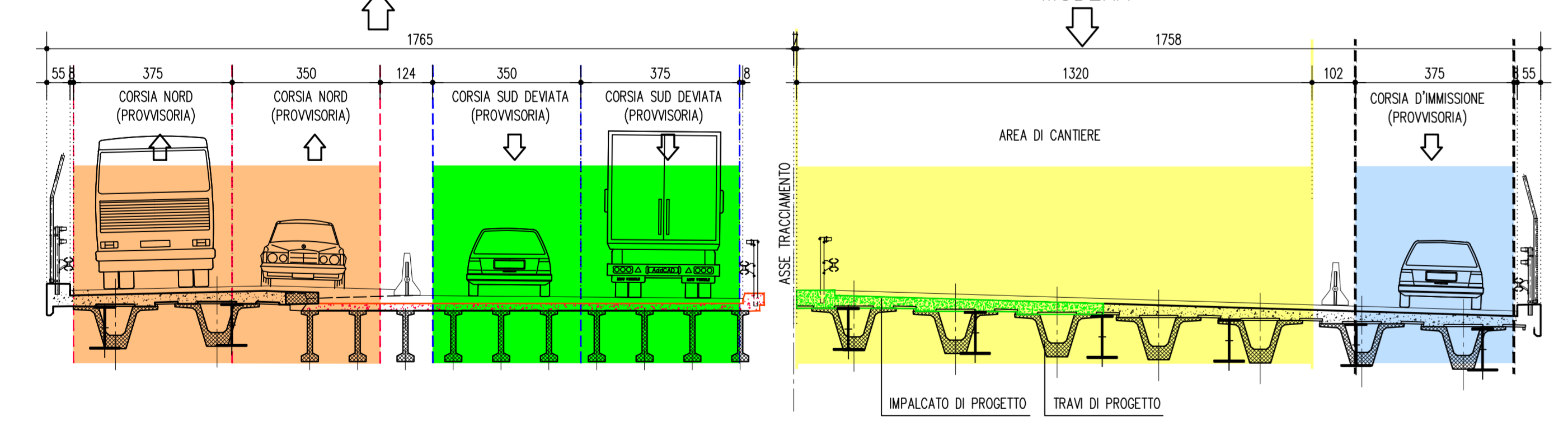
SEZIONE A-A – FASE 4 1:100
