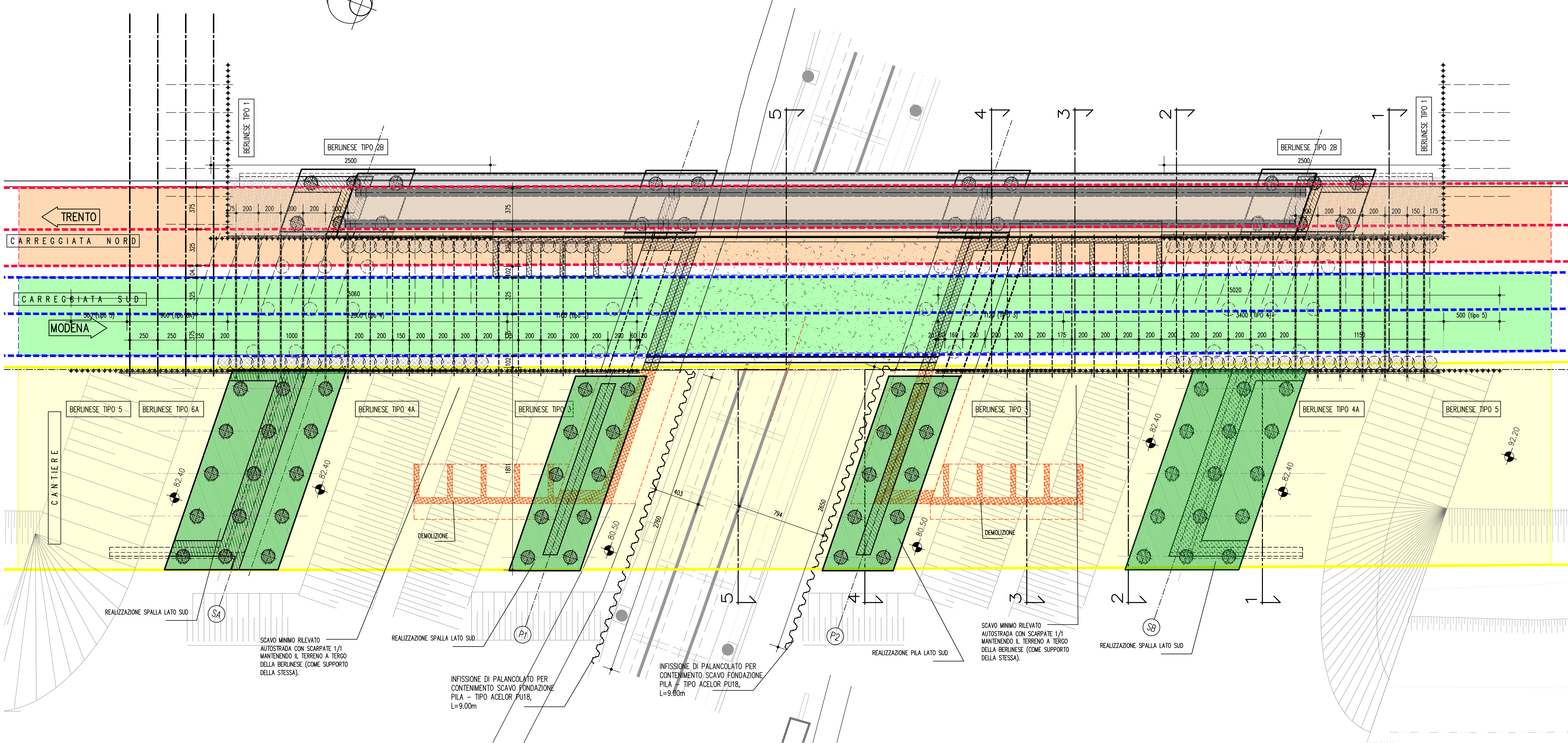
FASE 2 - PLANIMETRIA 1:200
