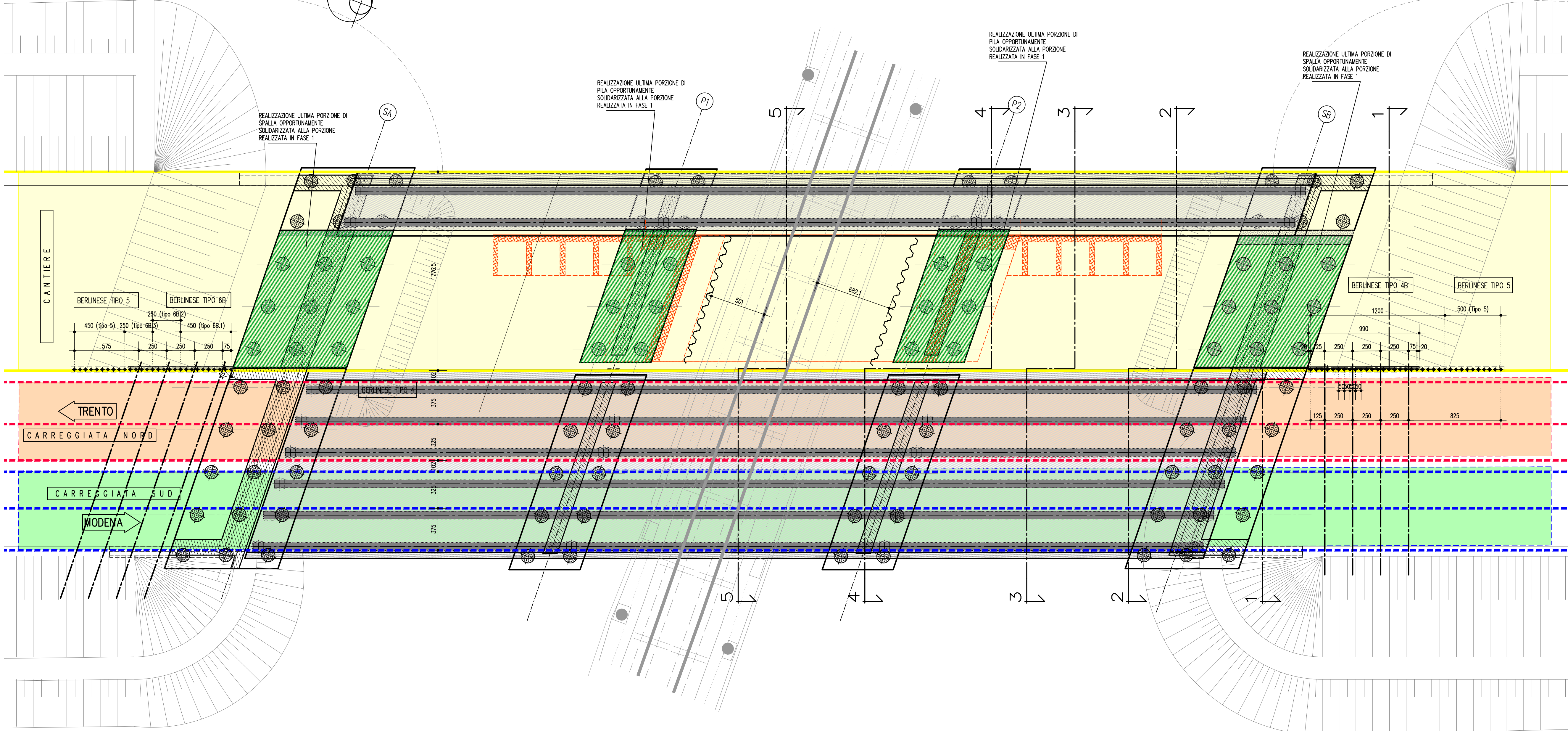
FASE 3 - PLANIMETRIA 1:200
