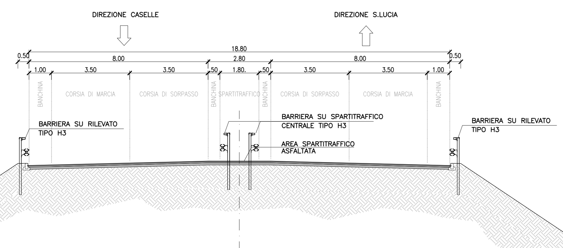
PROGETTO SEZIONE TIPOLOGICA A-A Scala 1:100
