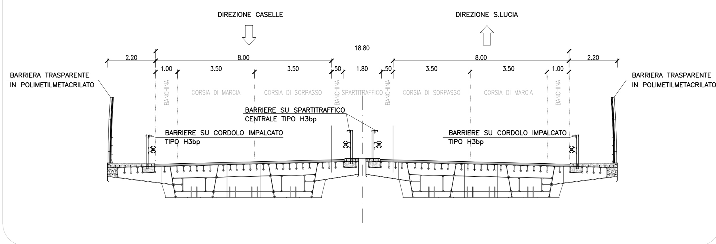
PROGETTO SEZIONE TIPOLOGICA B-B Scala 1:100
