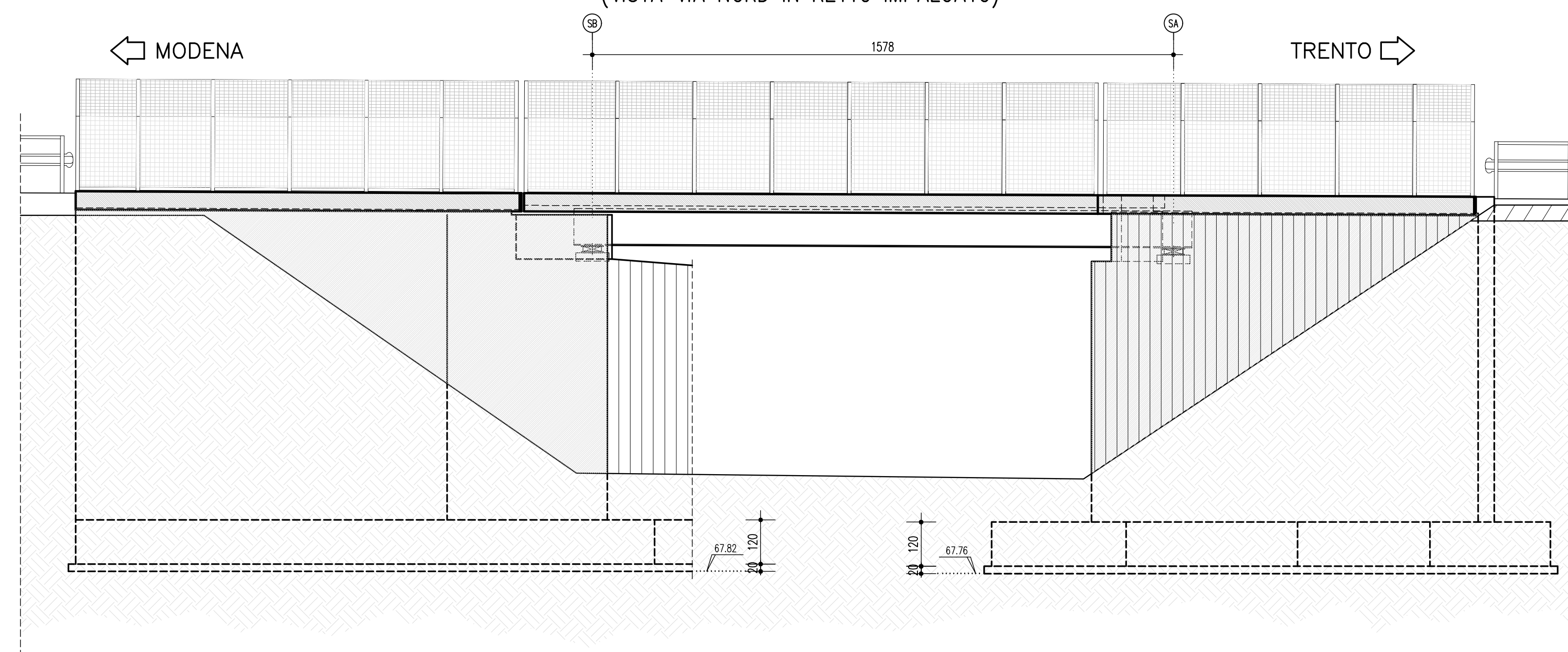
PROSPETTO LONGITUDINALE SCALA 1:100 (VISTA VIA NORD IN RETTO IMPALCATO)
