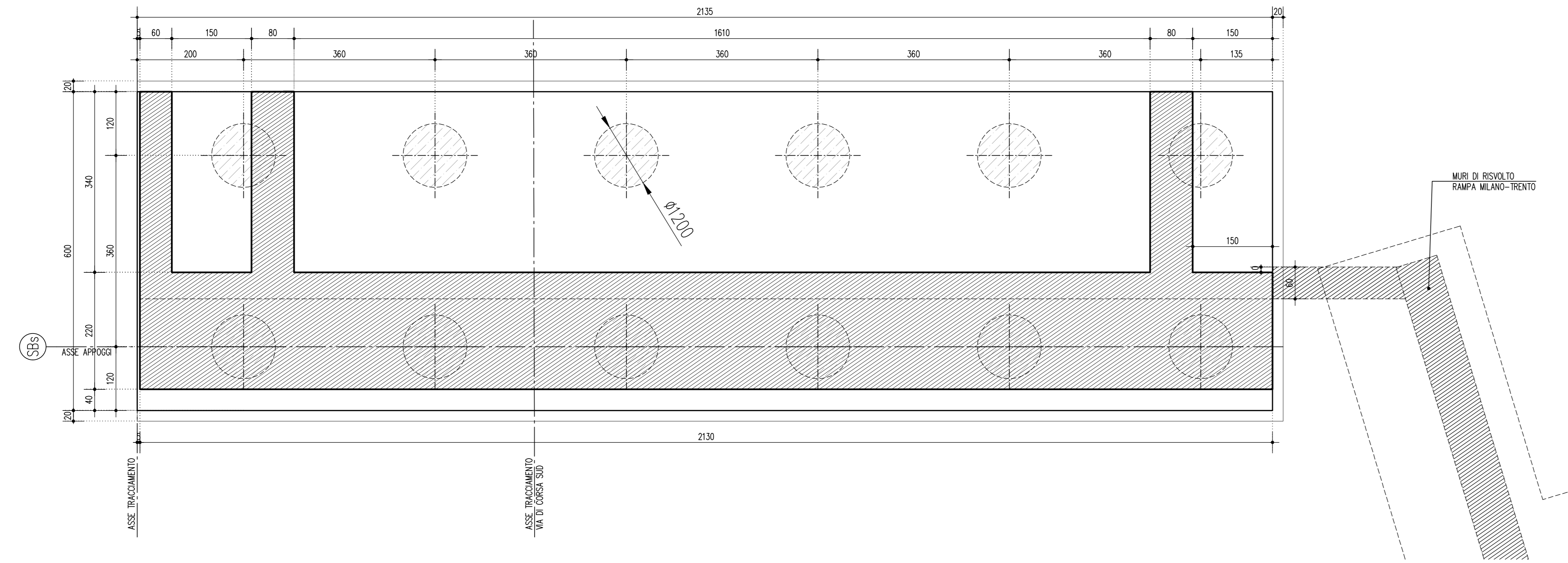
PIANTA QUOTA APPOGGI SPALLA (SBs) 1:50
