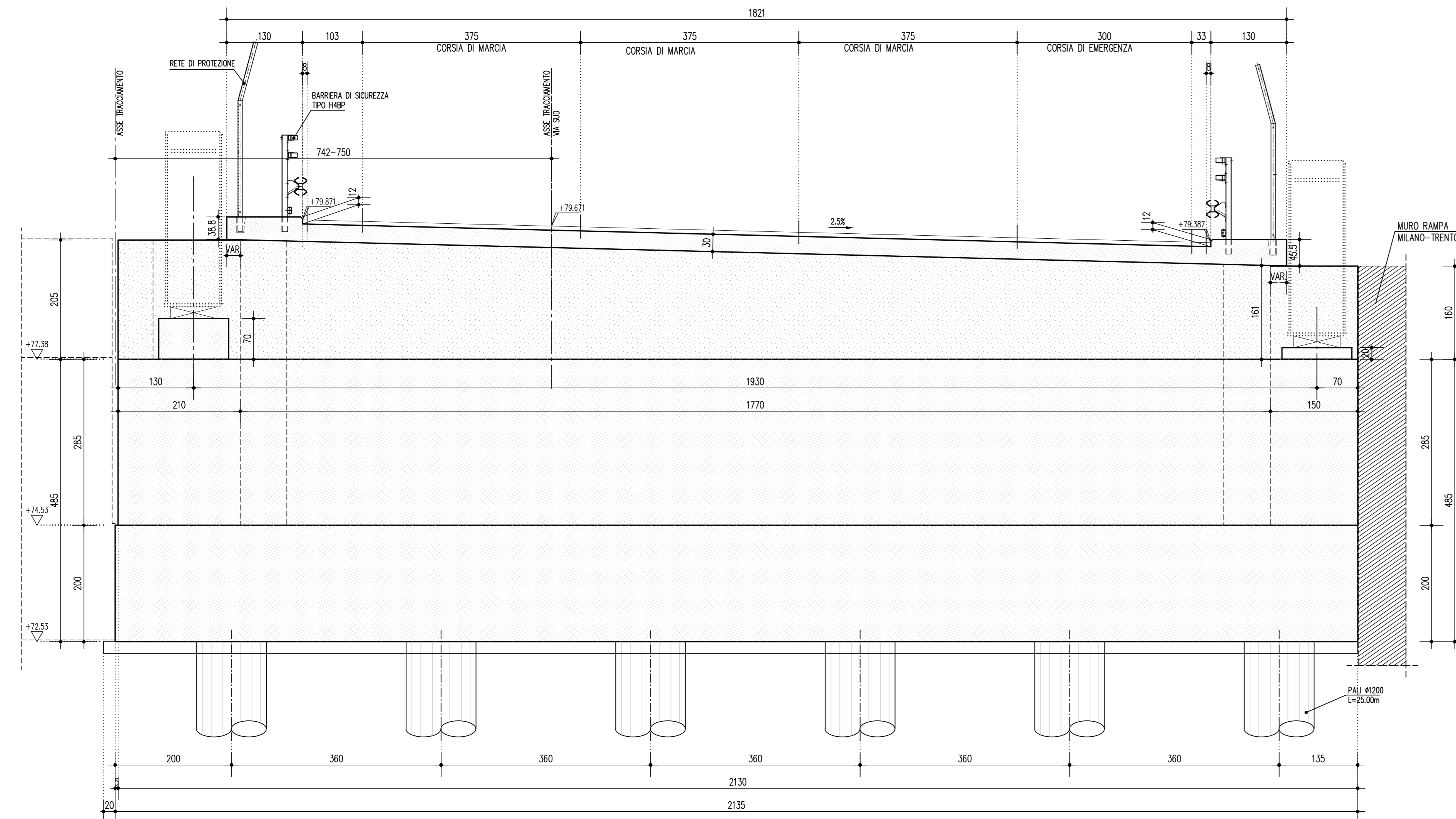
PROSPETTO SPALLA (SBs) 1:50
