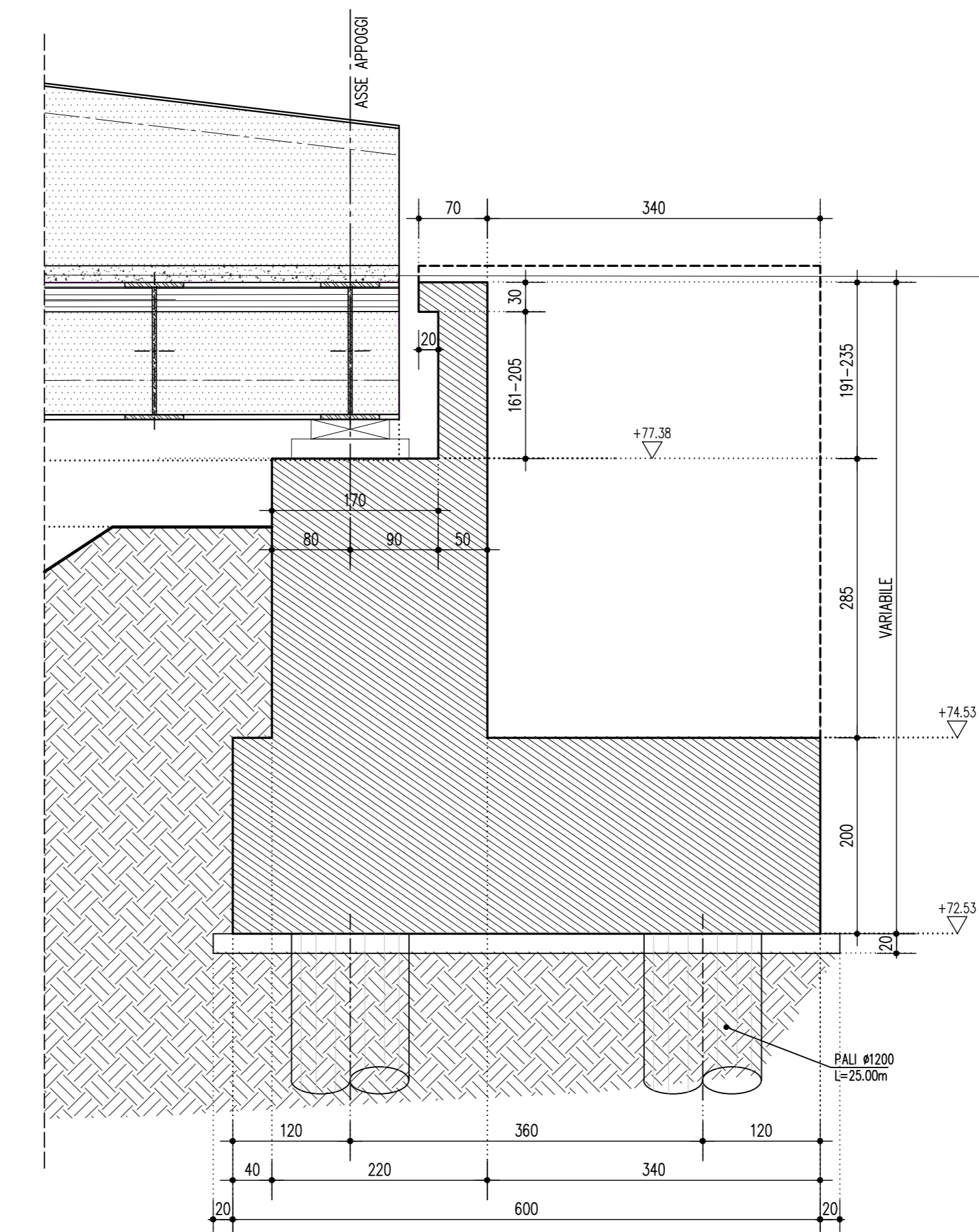
SEZIONE SPALLA (SBs) 1:50 (in asse tracciamento)
