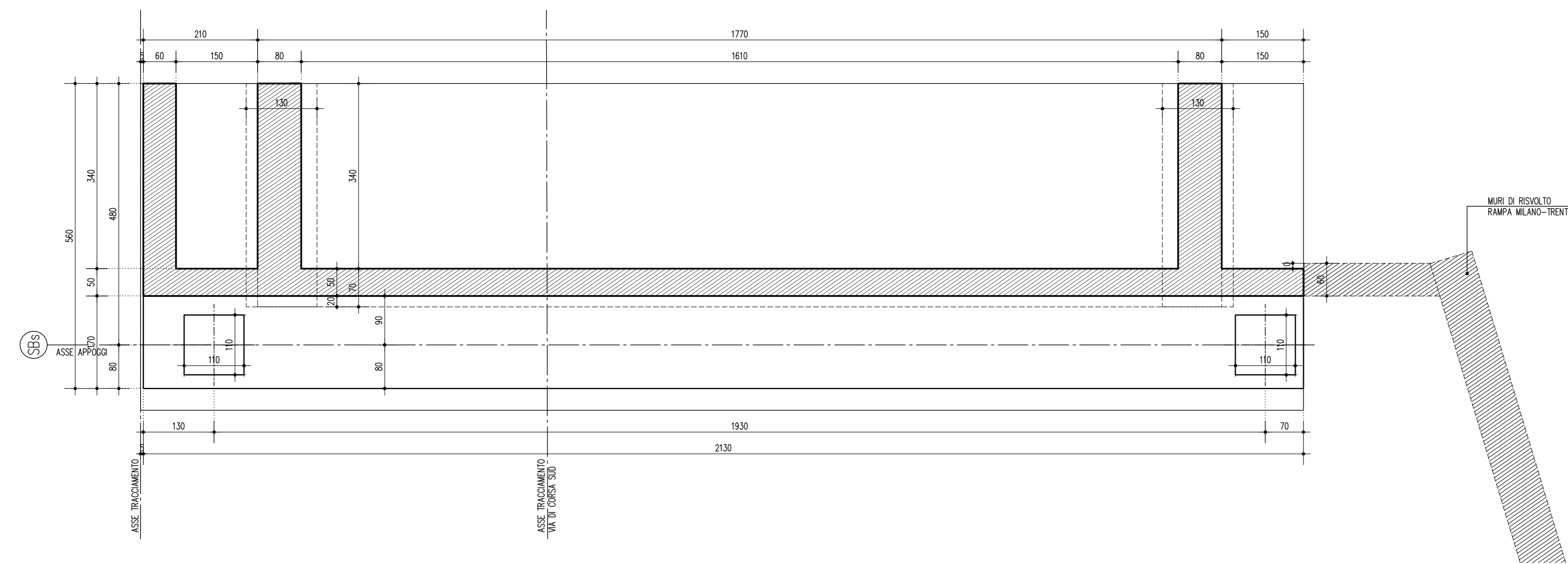
PROSPETTO SPALLA (SBs) 1:50
