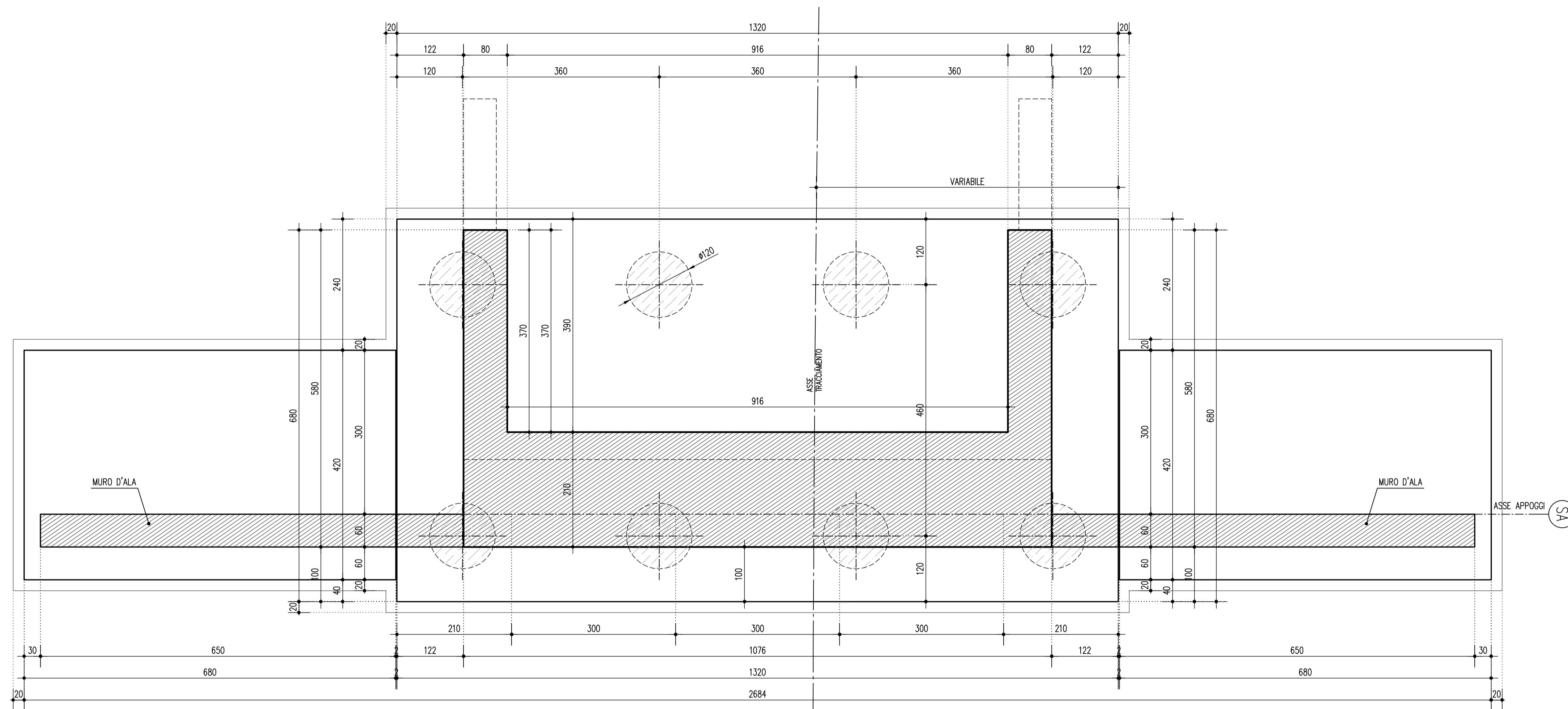
PIANTA FONDAZIONE E SPICCATO ELEVAZIONE SPALLA A 1:50
