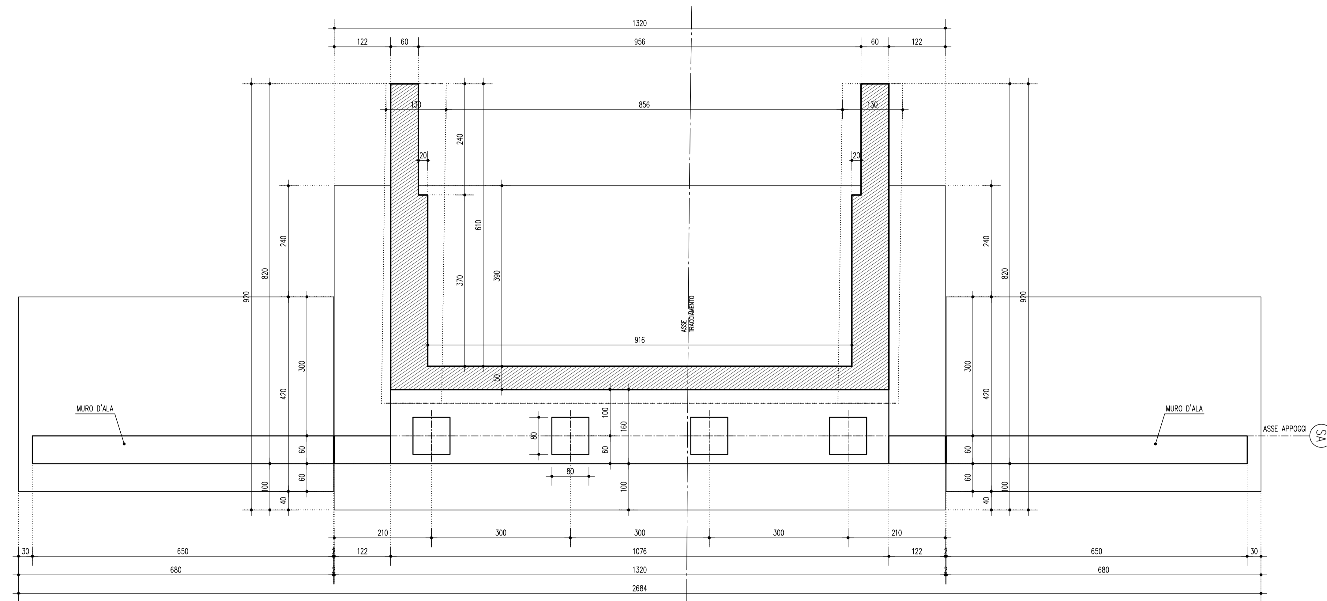
PIANTA QUOTA APPOGGI SPALLA A 1:50
