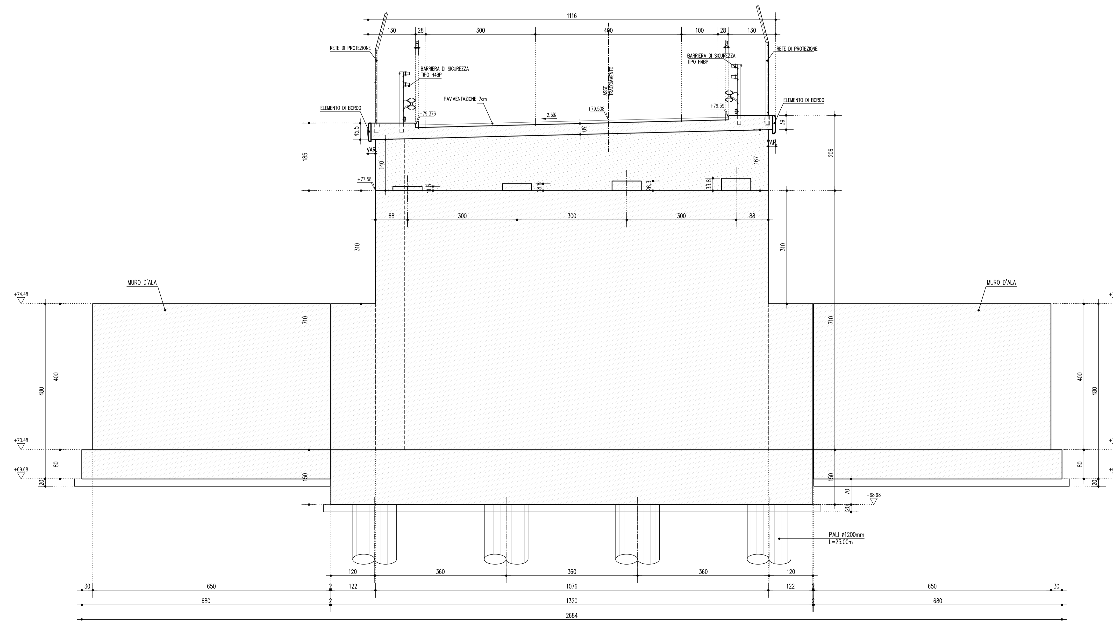
PROSPETTO SPALLA A 1:50
