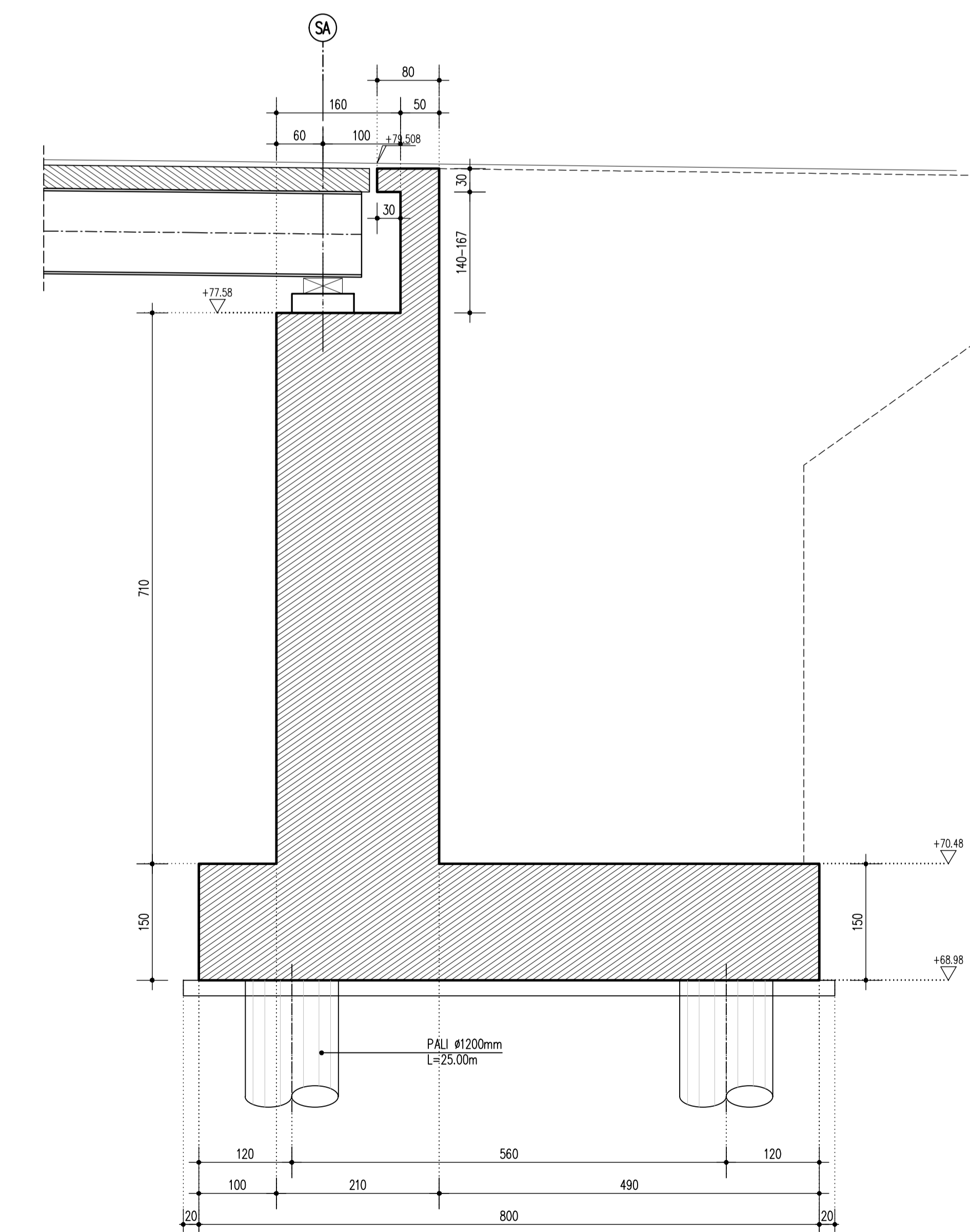
SEZIONE SPALLA A 1:50
