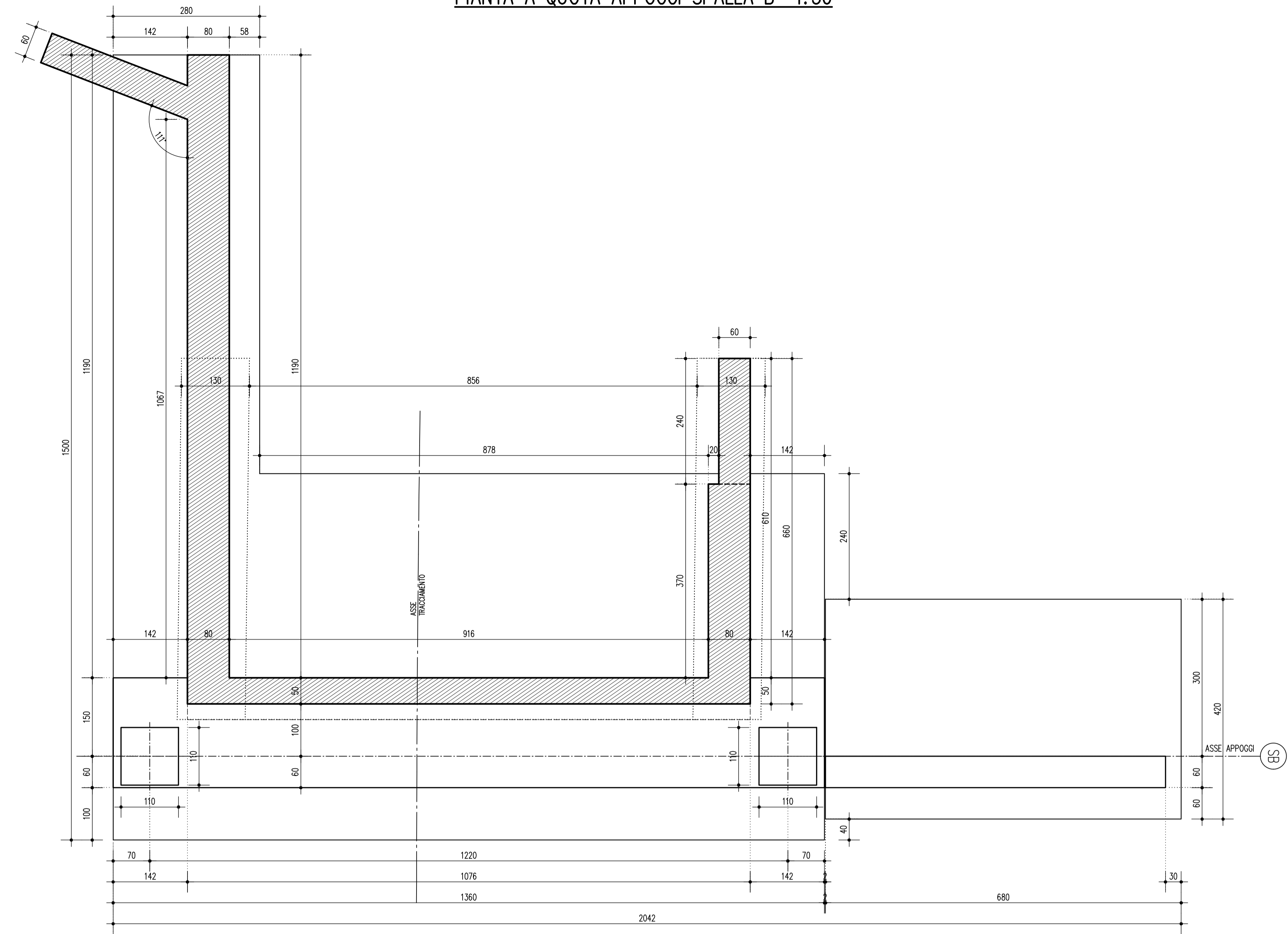
PIANTA A QUOTA APPOGGI SPALLA B 1:50
