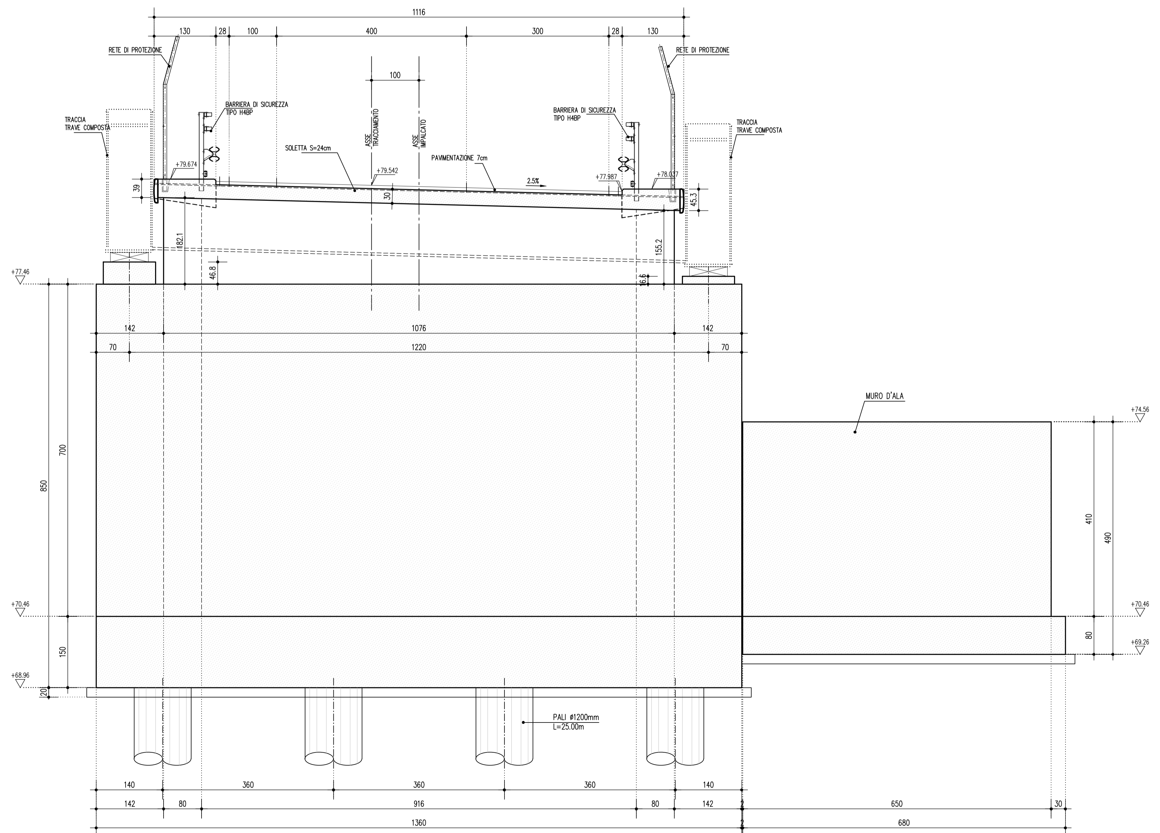
PROSPETTO SPALLA B 1:50
