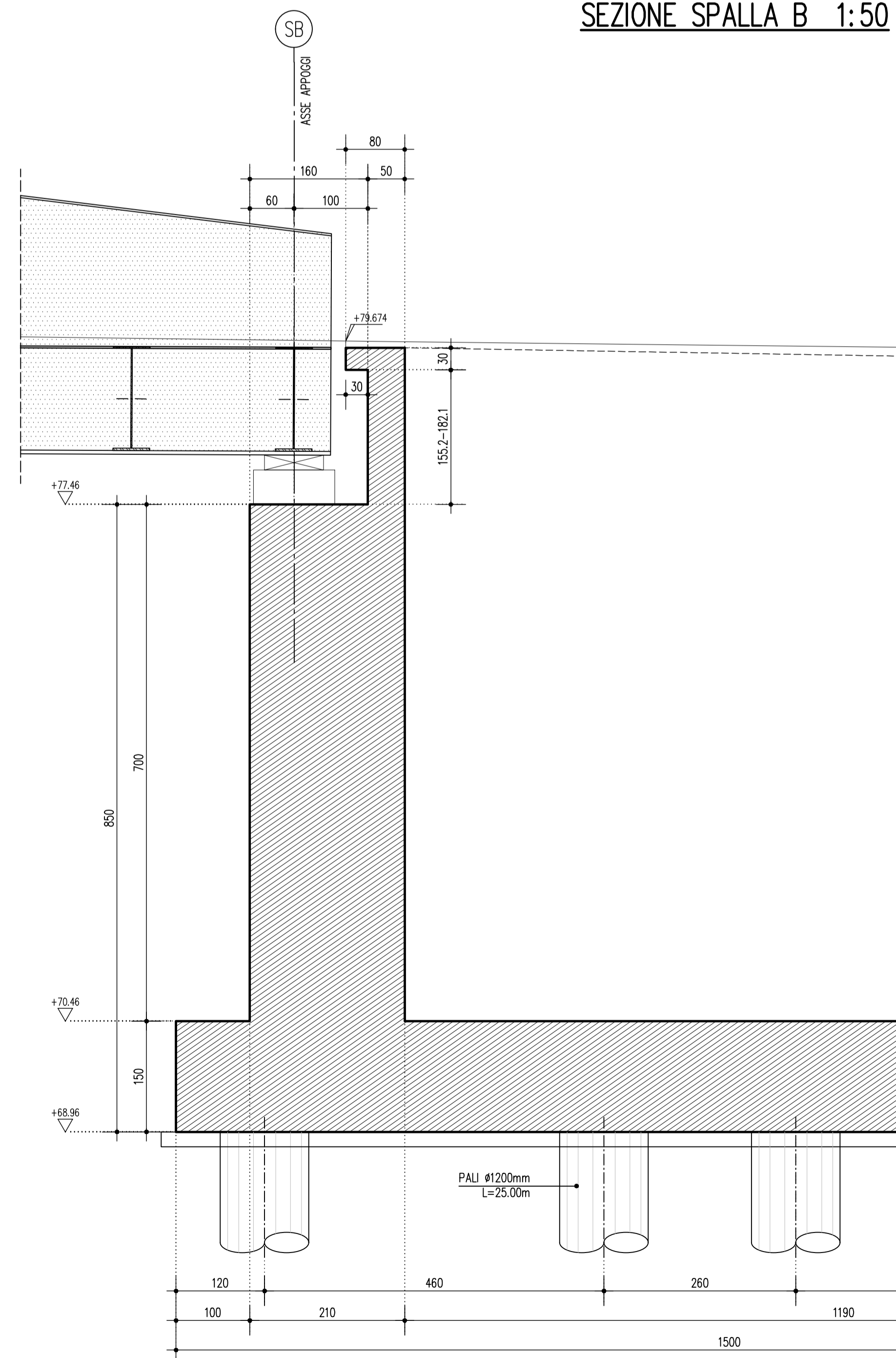
SEZIONE SPALLA B 1:50
