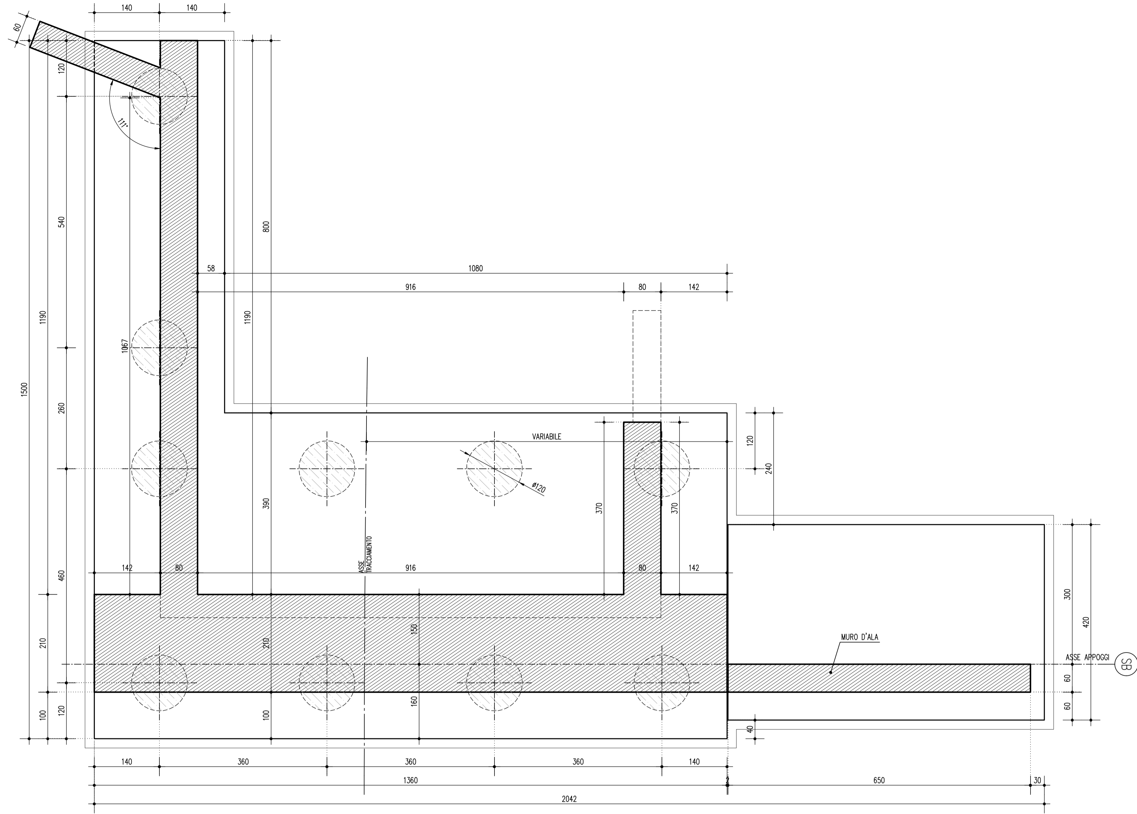
PIANTA FONDAZIONE E SPICCATO ELEVAZIONE SPALLA B 1:50
