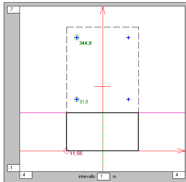
M < 0 ( M_{Sd}=-165 kNm)
