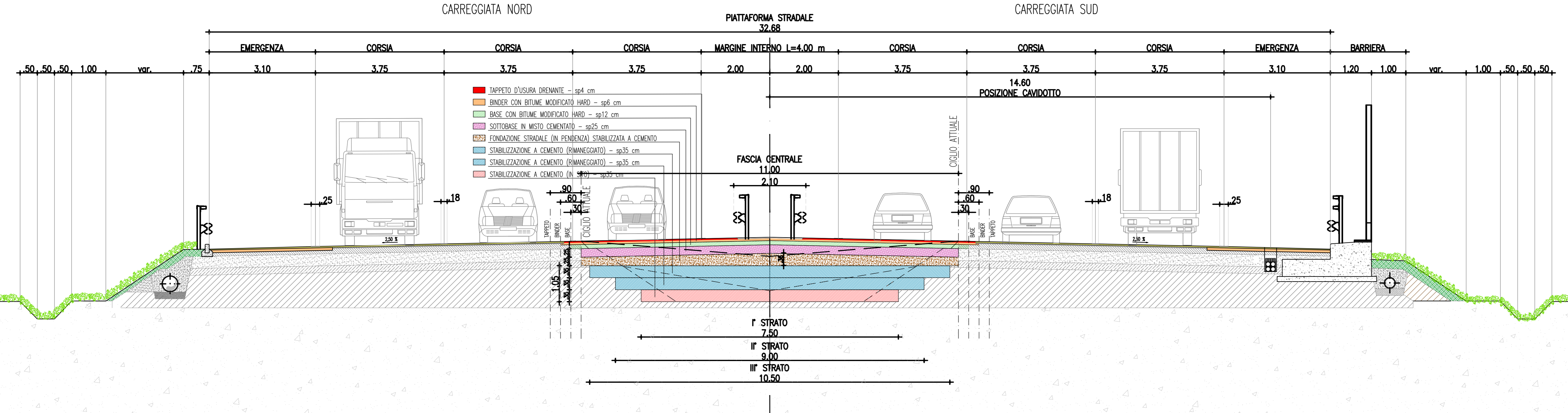
SEZIONE TIPO - STATO DI PROGETTO scala 1:50
