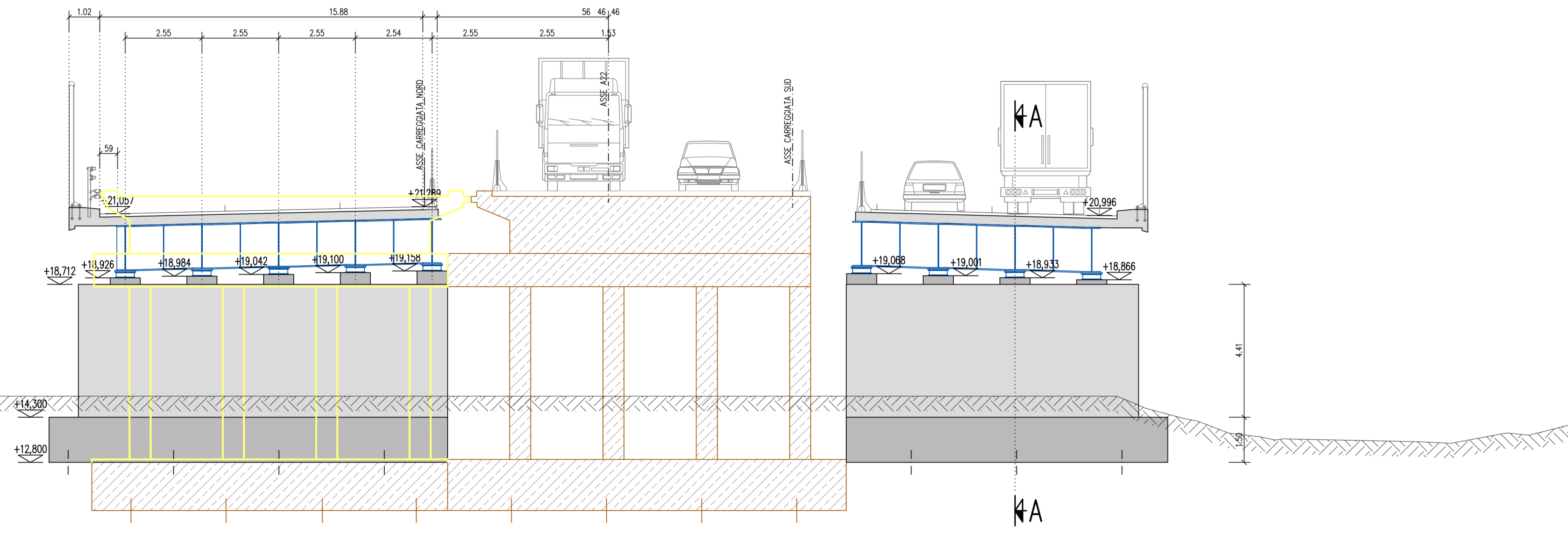
SEZIONE SPALLA NORD - FASE 2 1:100
