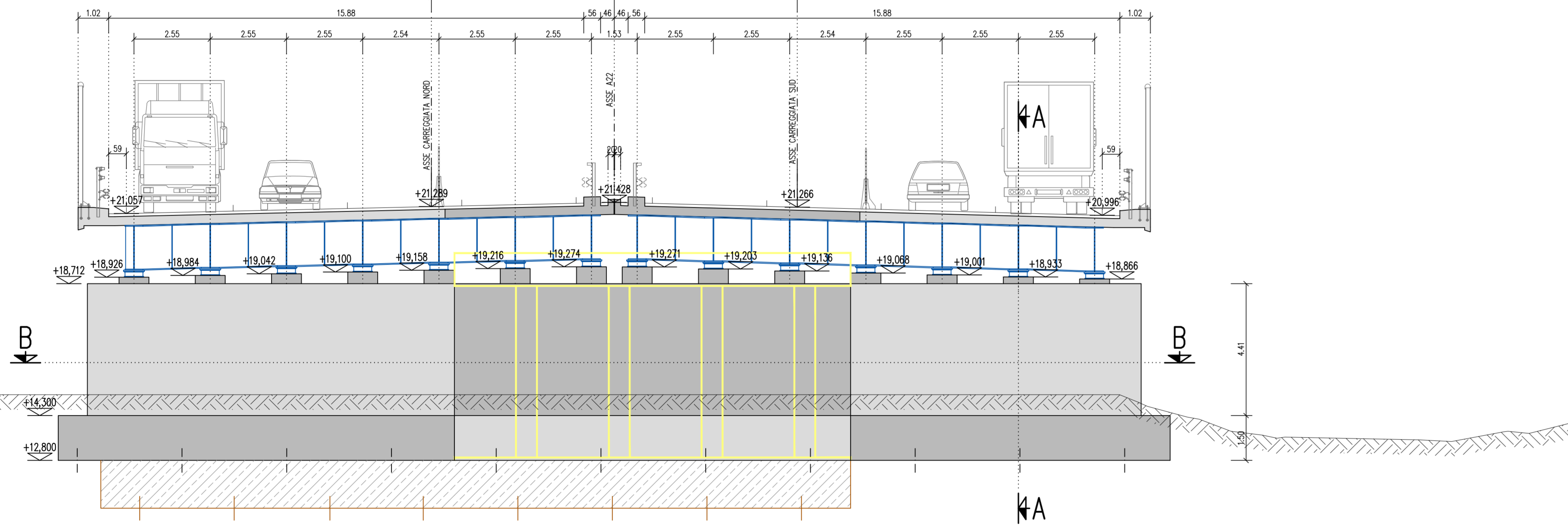
SEZIONE SPALLA NORD - FASE 3 1:100
