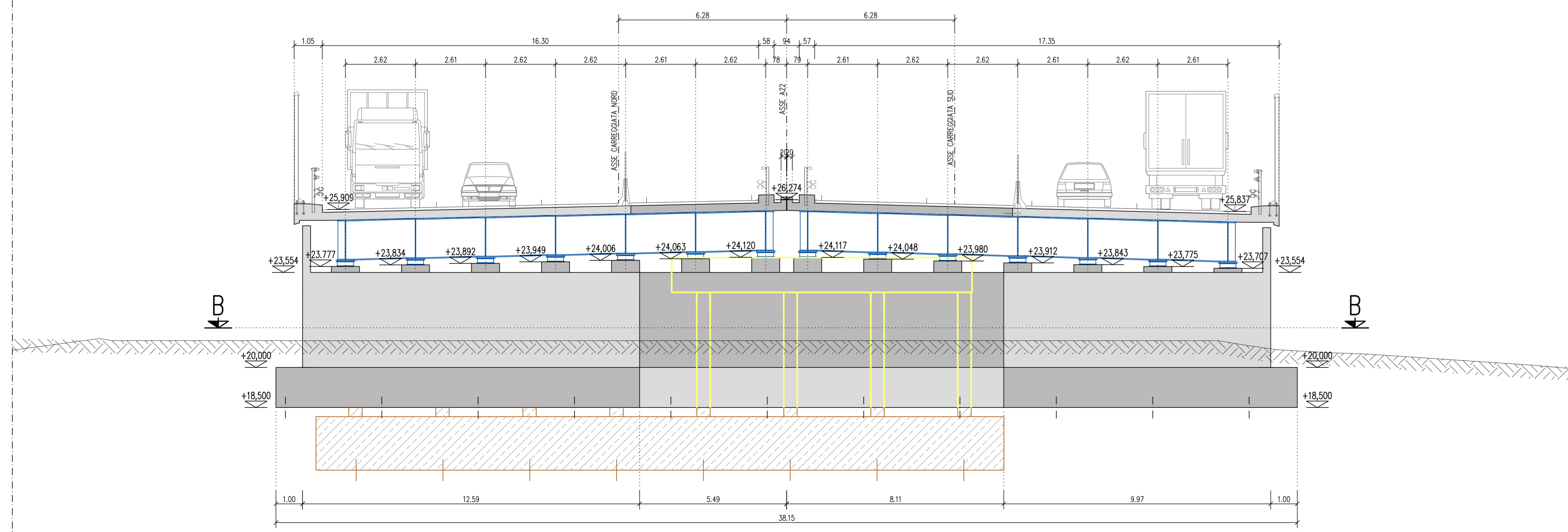
SEZIONE SPALLA NORD - FASE 3 1:100
