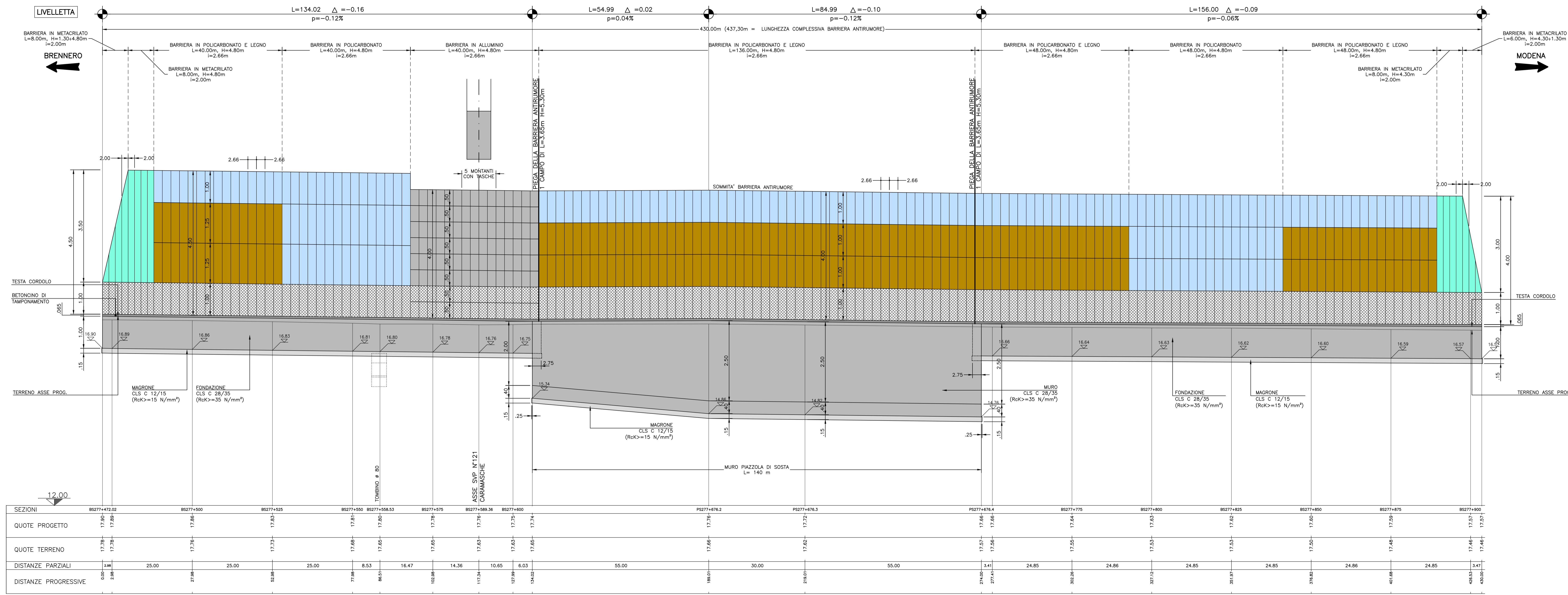
PROFILO LONGITUDINALE SCALA LUNGHEZZE 1:500 SCALA ALTEZZE 1:50
