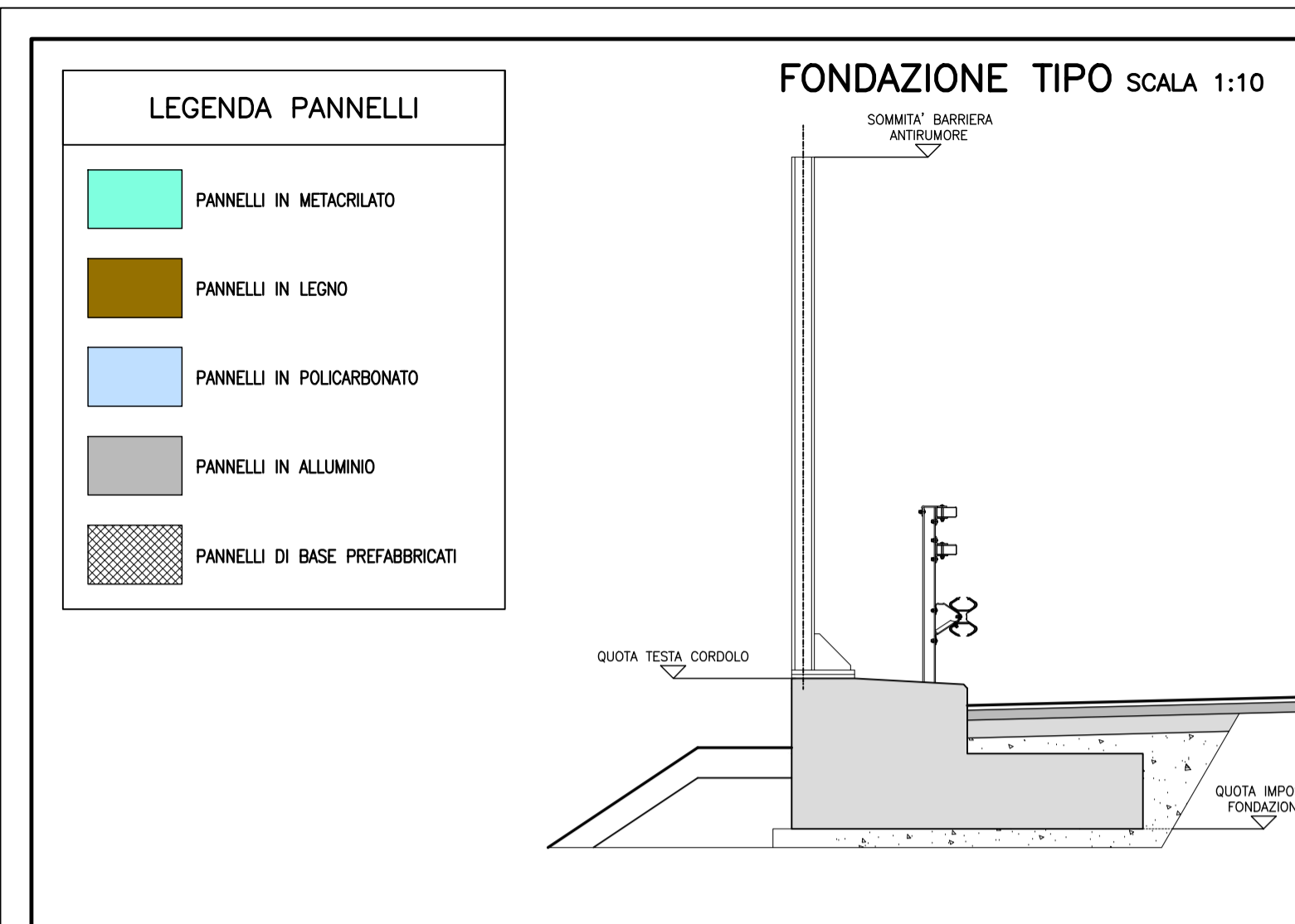
FONDAZIONE TIPO SCALA 1:10
