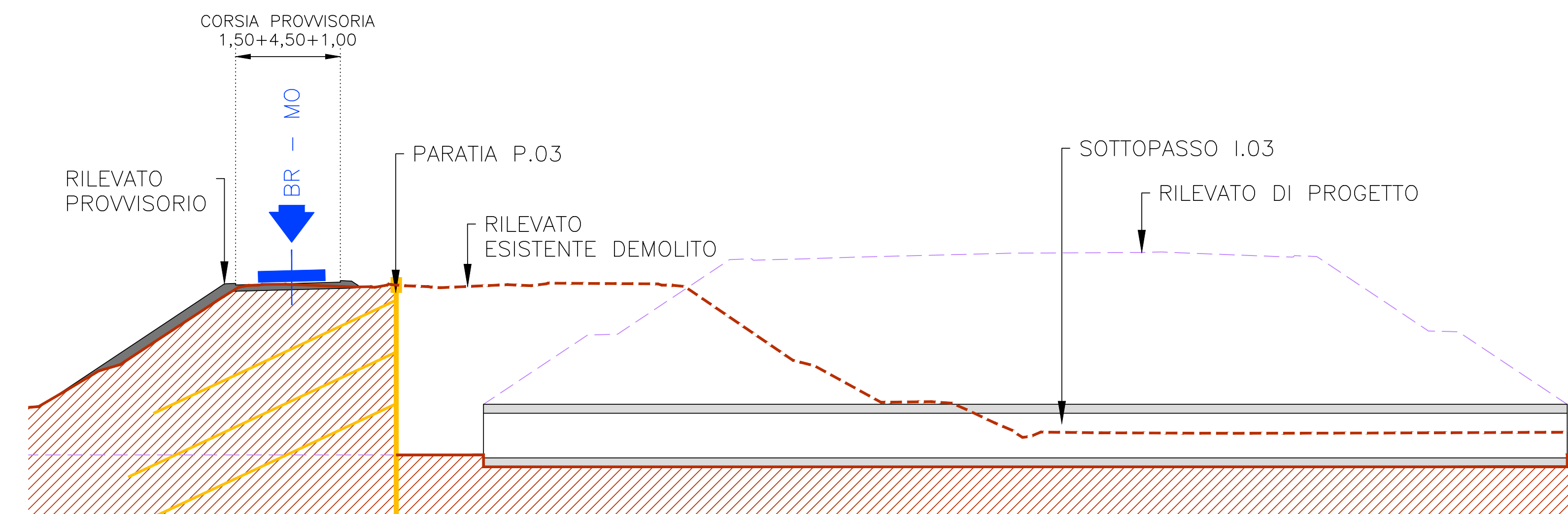
SEZIONE 3 scala 1:250
