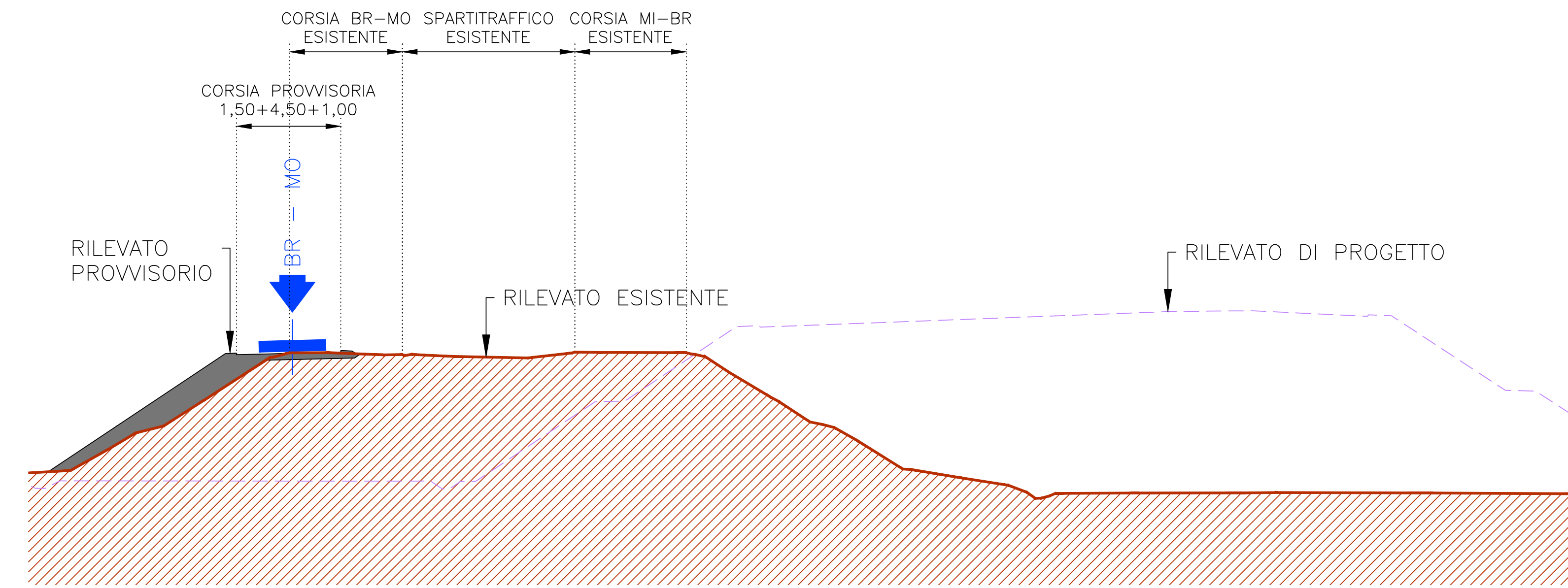
SEZIONE 2 scala 1:250
