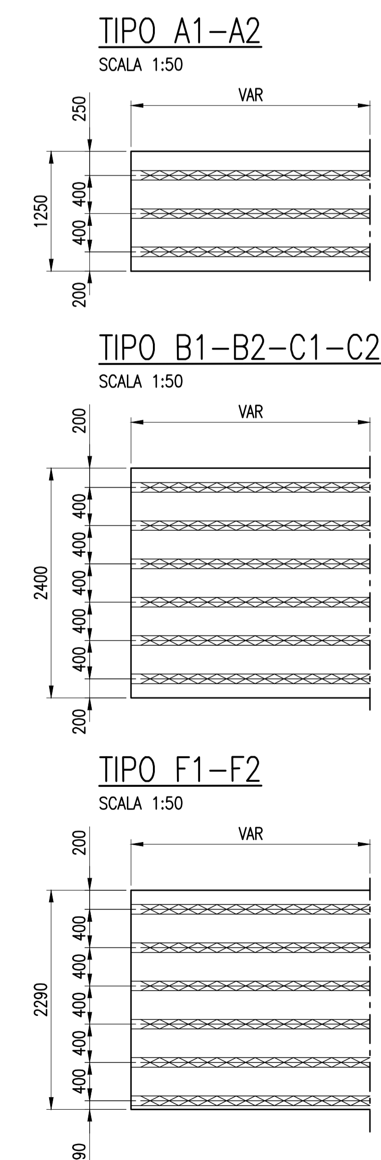
DETTAGLIO PREDALLES
