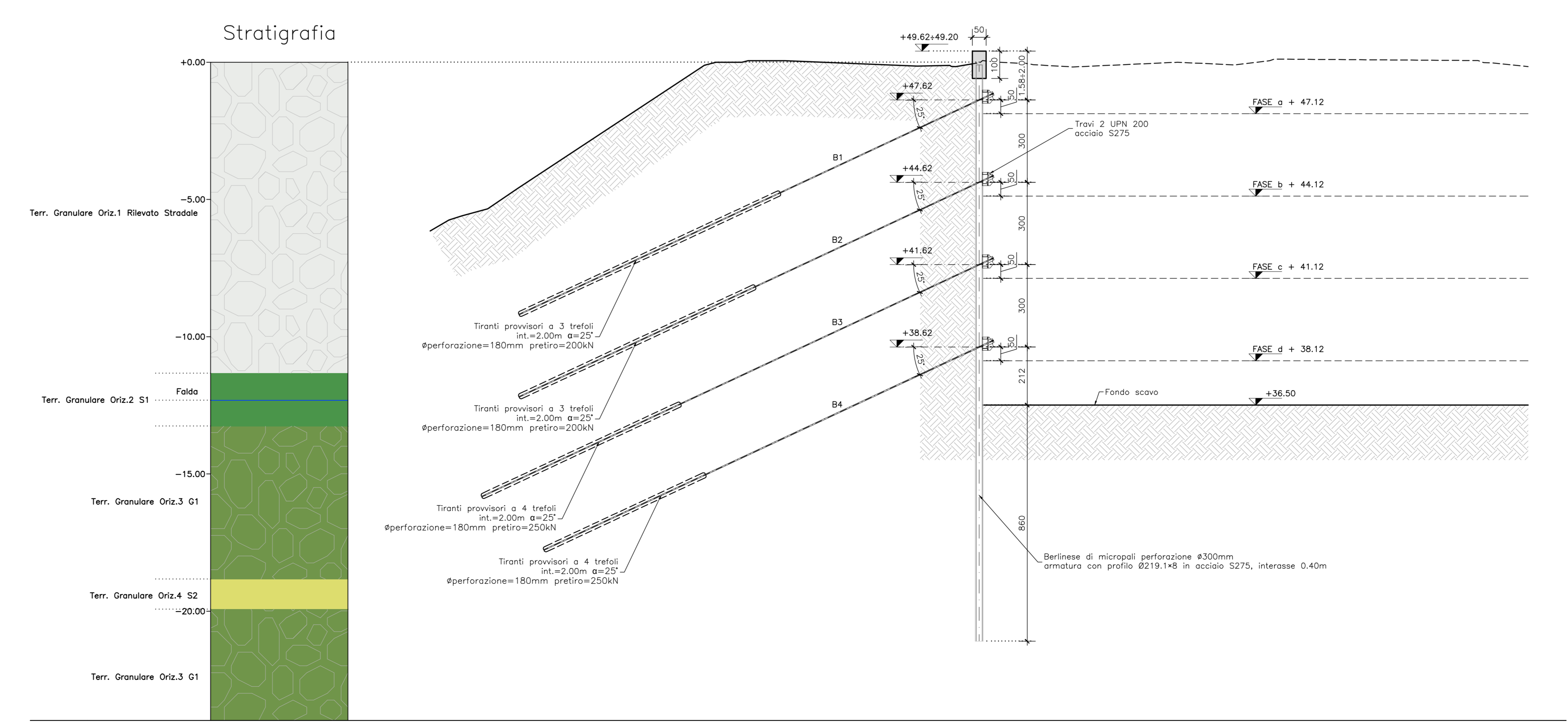
SEZIONE B-B scala 1:100
