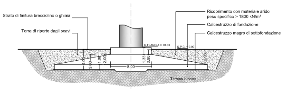
Figura 1 – Pianta e vista della fondazione tipo dell'aerogeneratore
