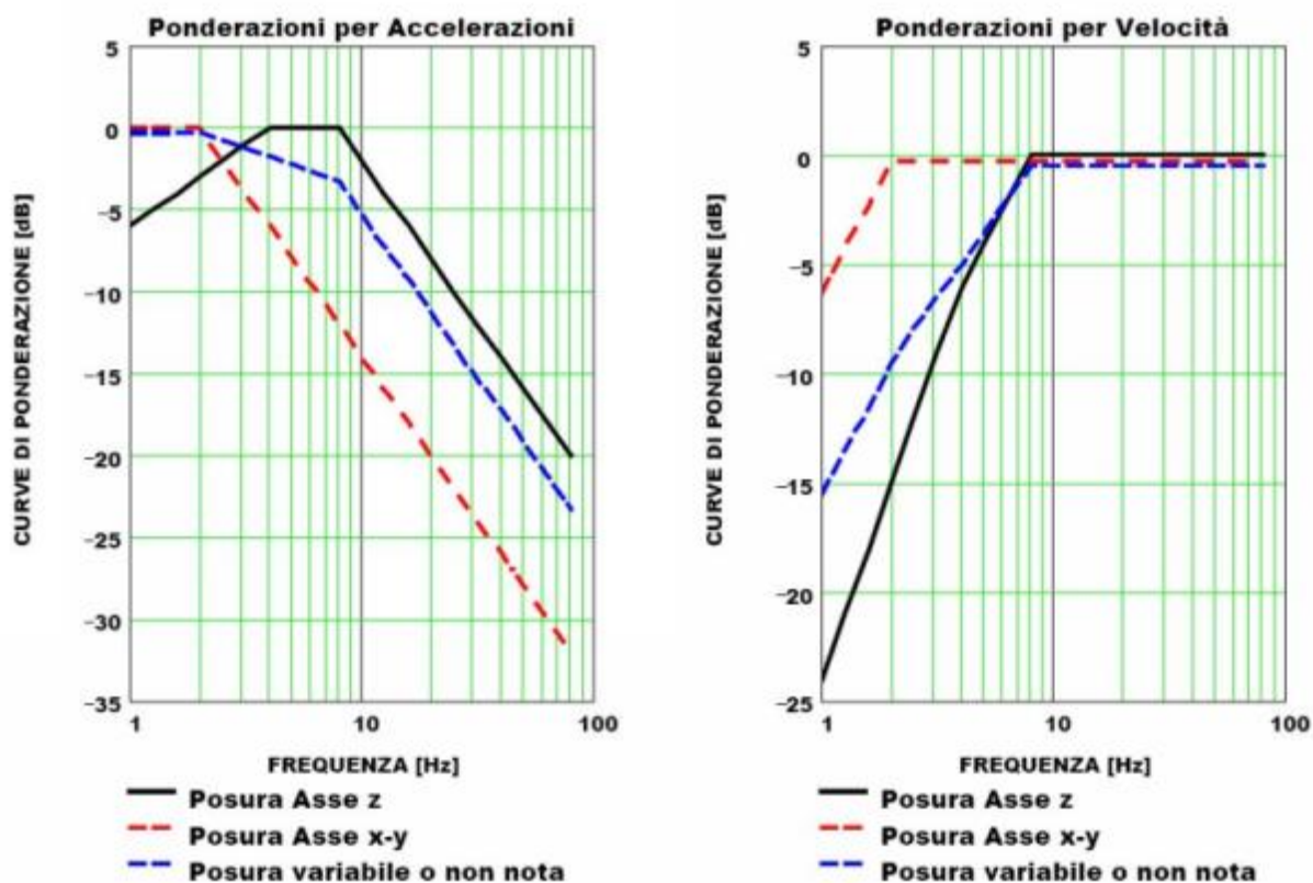
Figura 2 – Curve di ponderazione (ISO) per vibrazioni lungo gli assi verticali, orizzontali e per postura non nota nell'intervallo di frequenze 1÷80 Hz
