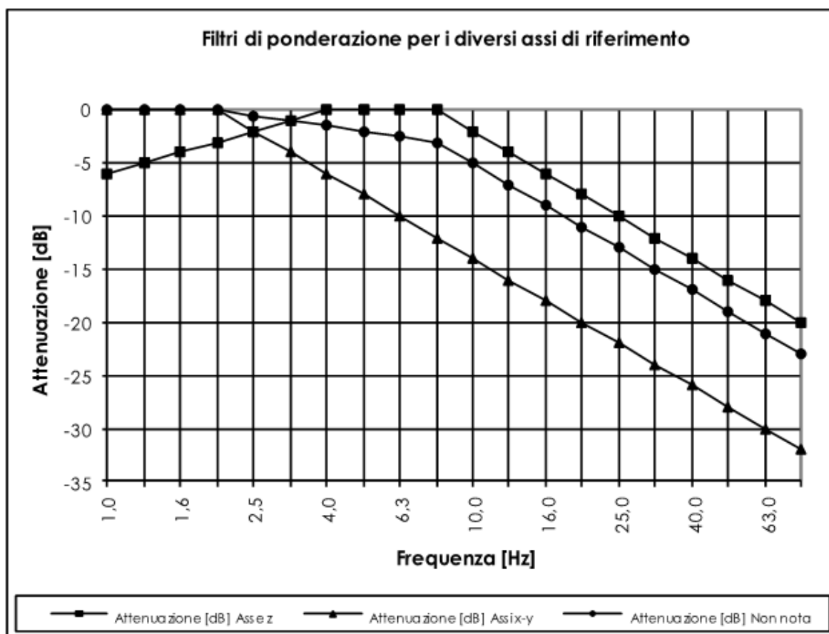
Figura 17– Curve di ponderazione delle vibrazioni indicate dalla UNI 9614:2017 per i diversi assi di riferimento
