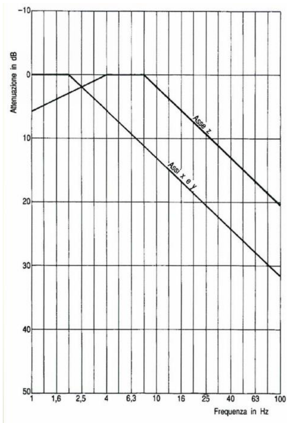
Figura 3 – Curve di ponderazione norma UNI 9614:2017
