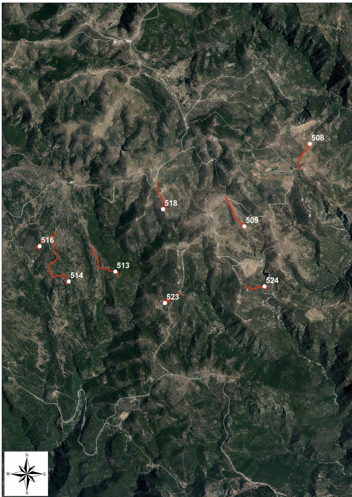
Figura 10 - Aerogeneratori di progetto su base aerofotogrammetrica.
