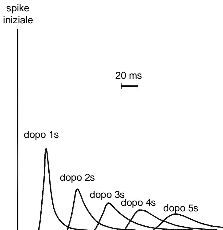
Figura 6 - Progressiva variazione della forma d'onda durante la propagazione a causa dell'effetto di attenuazione (Anstey, 1977)
