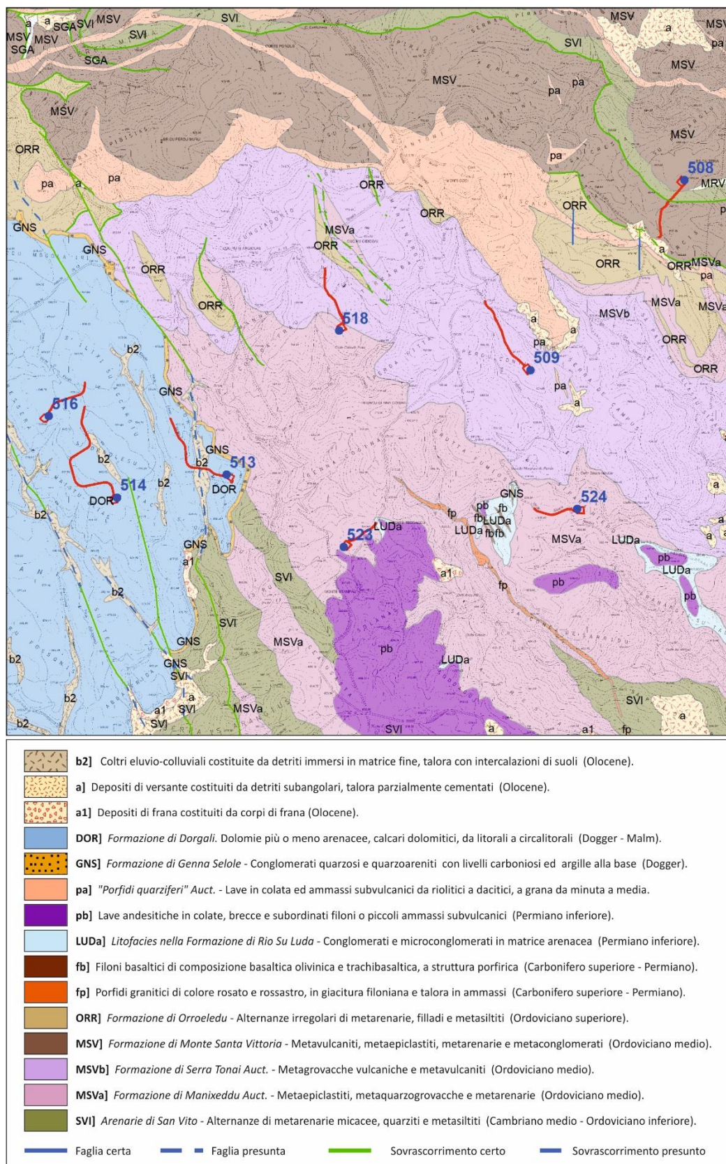
Figura 12– Stralcio della “CARTA GEOLOGICA D’ITALIA a cura di APAT, modificata, fuori scala
