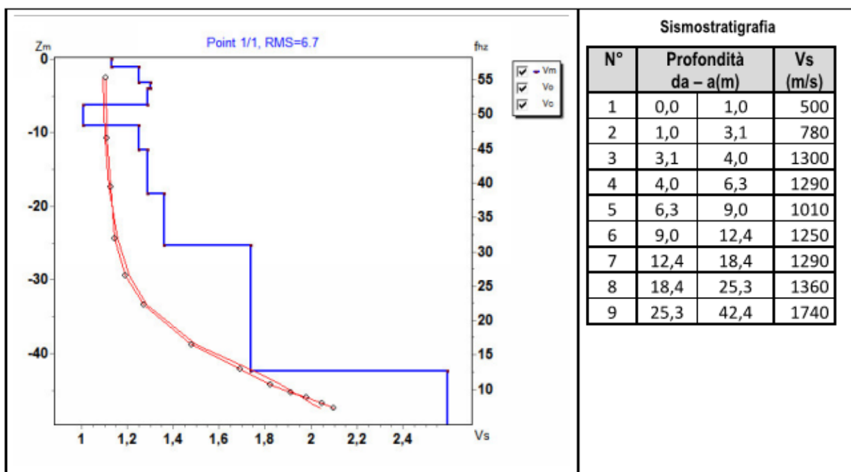
MASW M1 – PROFILO Vs (Vs eq= 1020 m/s)
