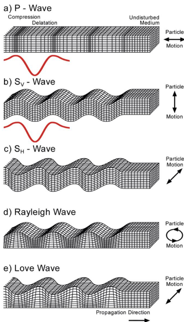
Figura 4 – Caratteristiche delle onde sismiche
