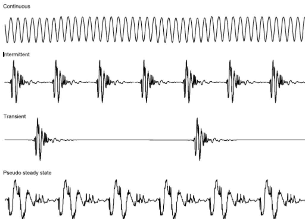
Figura 5 – Variazioni temporali delle vibrazioni
