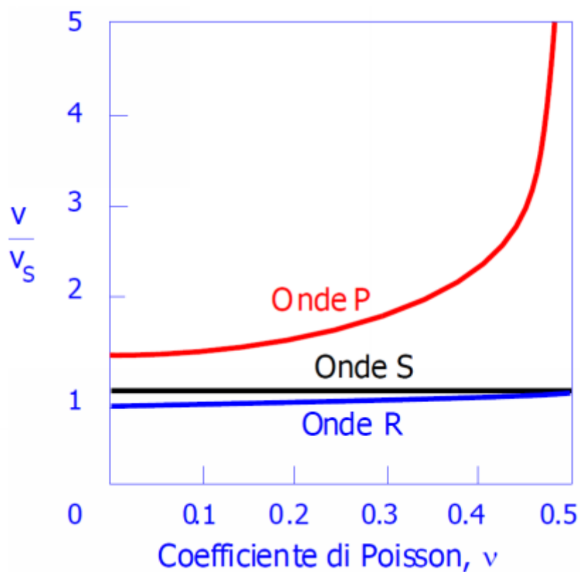
Figura 16– Relazione tra la velocità delle onde P, R ed S in funzione dei valori assunti dal coefficiente di Poisson (Richard at. al. mod., 1970)
