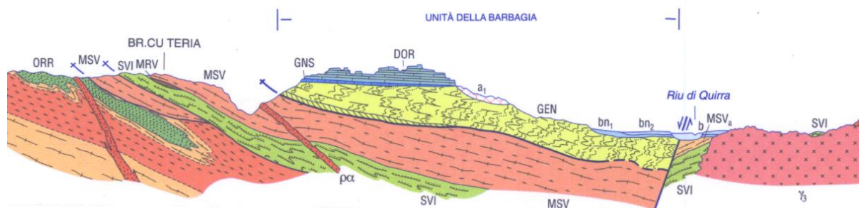
Figura 11- Schema tettonico strutturale del settore di intervento rappresentato su sezione geologica (Carta geologica d'Italia - Foglio 541 Jerzu in scala 1:50.000, modificata).
