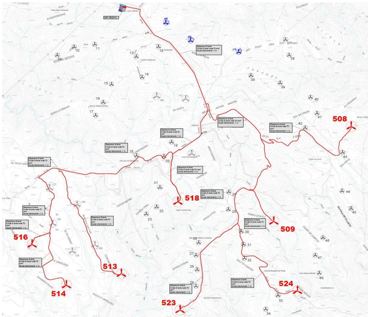
Figura 3 – Nuovi aerogeneratori in progetto ed elettrodotti MT (in rosso)
