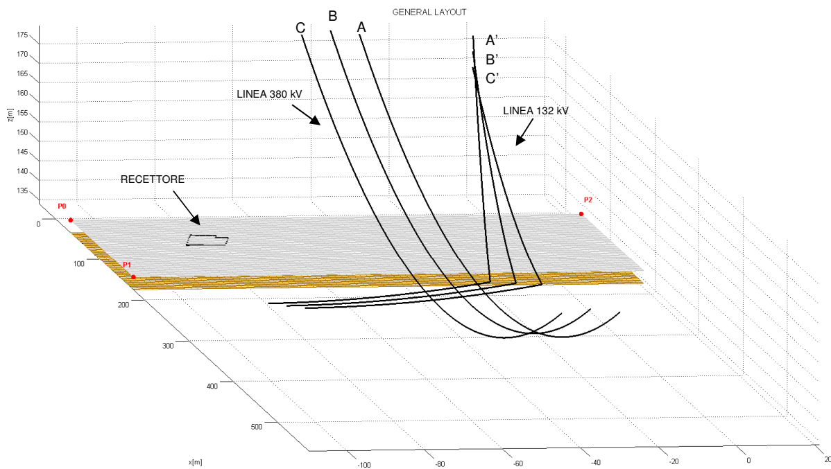
Sezione di calcolo orizzontale – Modello
