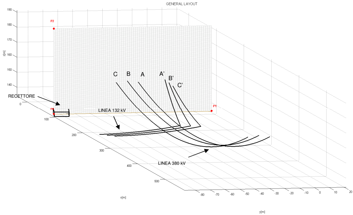
Sezione di calcolo verticale - Modello
