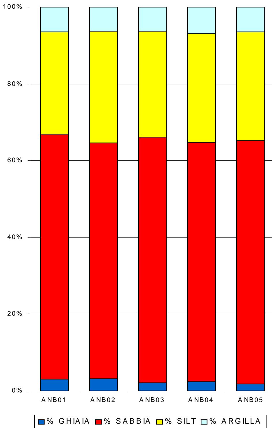
Fig. 5.2.6a – Intervalli granulometrici
