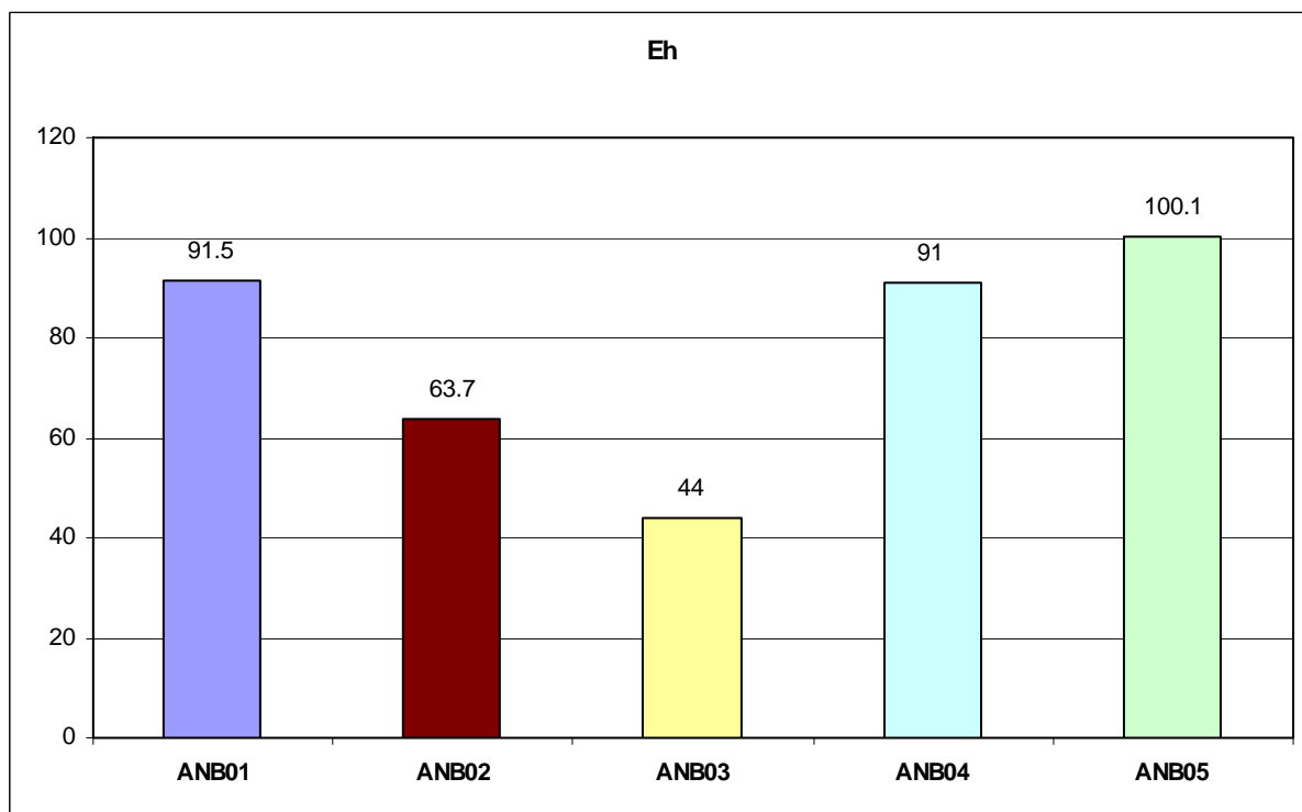
Fig. 5.2.5a – Valori di pH ed Eh nelle diverse postazioni
