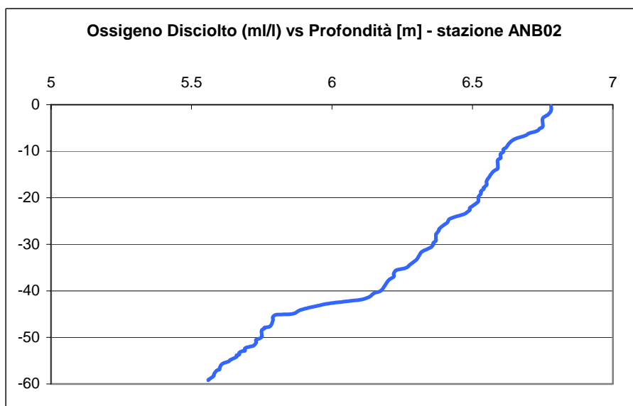
Fig. 5.2.3d – Stazione ANB02: ossigeno disciolto in rapporto con la profondità.
