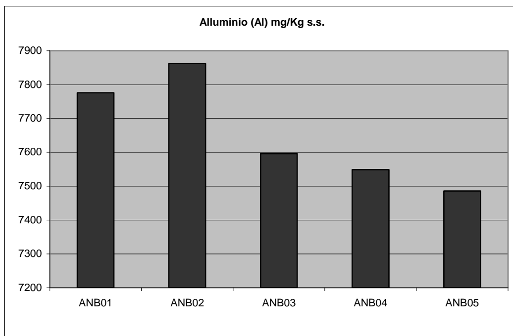
Fig 5.2.5d – Concentrazioni di Alluminio nelle varie stazioni
