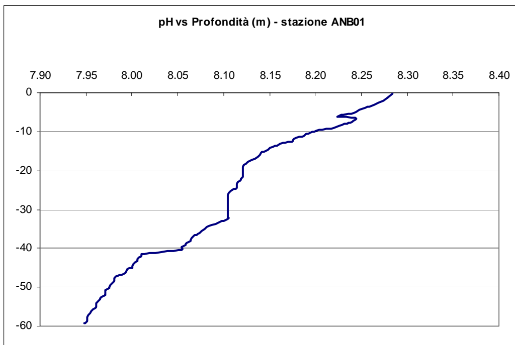
Fig. 5.2.3e – Stazione ANB01: pH in rapporto con la profondità.
