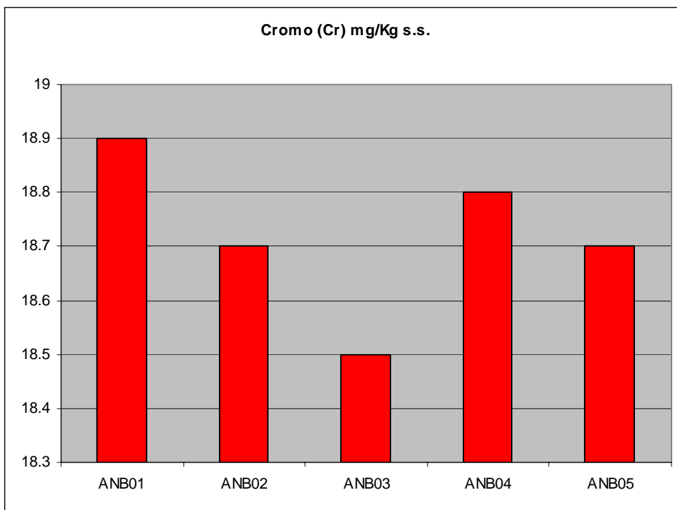
Fig 5.2.5e – Concentrazioni di Cromo nelle varie stazioni
