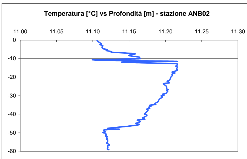
Fig. 5.2.1b – Temperatura in rapporto con la profondità (campione ANB02).
