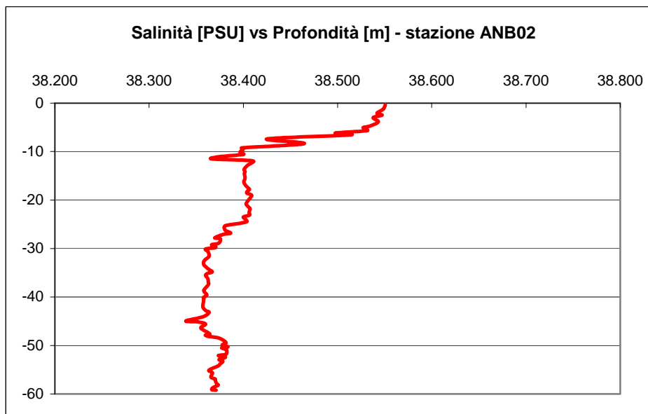
Fig. 5.2.3b – Stazione ANB02: salinità in rapporto con la profondità.
