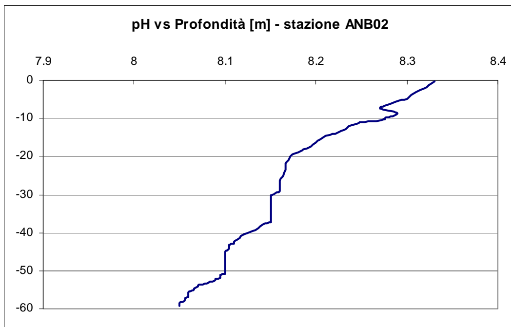
Fig. 5.2.3f – Stazione ANB02: pH in rapporto con la profondità.
