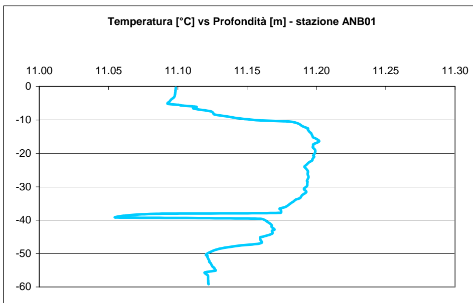
Fig. 5.2.1a – Temperatura in rapporto con la profondità (campione ANB01).
