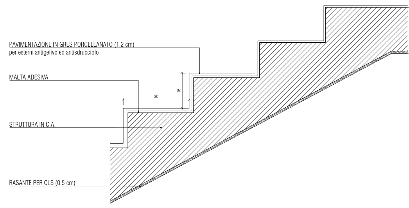
S11 SCALE E PIANEROTTOLI
