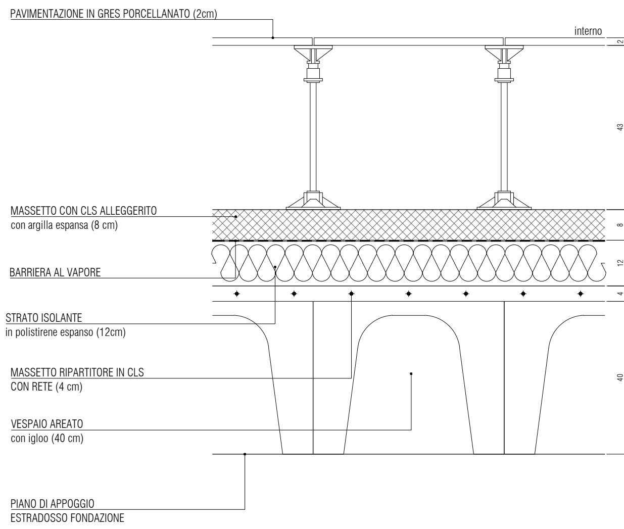
S1 SOLAIO CONTROTERRA EDIFICIO ESAZIONE (vespaio aerato + pavimento galleggiante)
