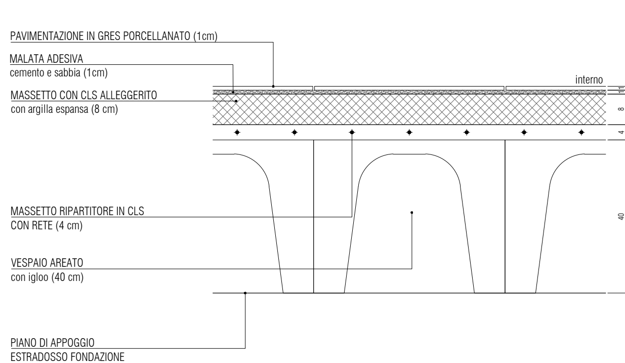
S5 SOLAIO CONTROTERRA EDIFICIO IMPIANTI
