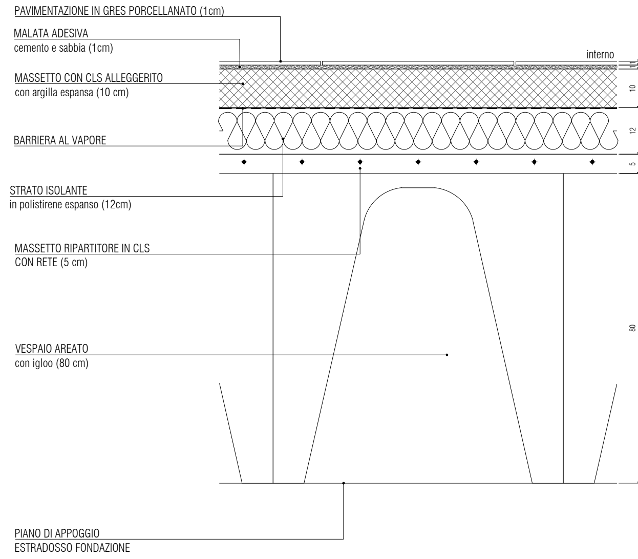
S2 SOLAIO CONTROTERRA EDIFICIO ESAZIONE (vespaio aerato)
