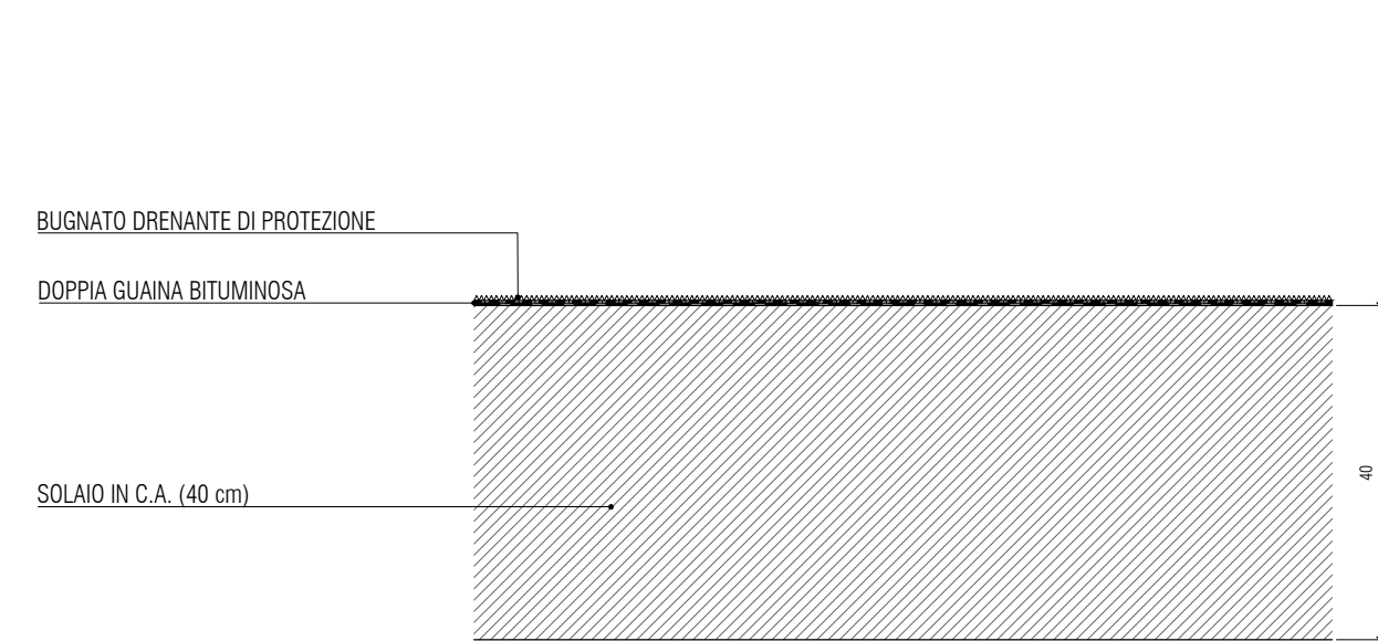
S8 SOLAIO COPERTURA CUNICOLO
