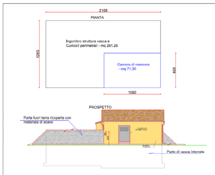
Schema dell'ingombro in pianta della vasca costituente il serbatoio di accumulo, ricoperta in terra, e relativo prospetto
