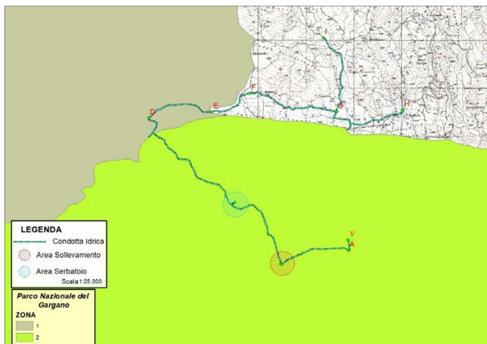
Parco Nazionale del Gargano – Ubicazione dell'intervento
