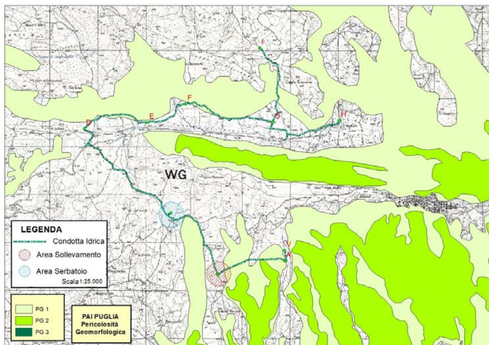
Pericolosità Geomorfologica
