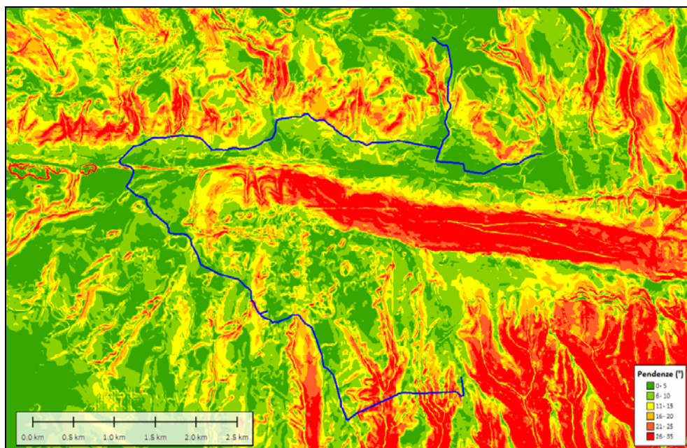
Carta delle pendenze dell’area
