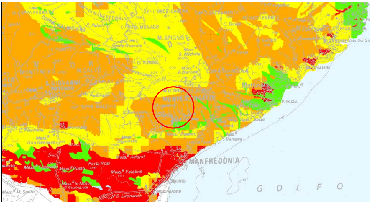
Carta di vulnerabilità intrinseca o naturale dell'acquifero
