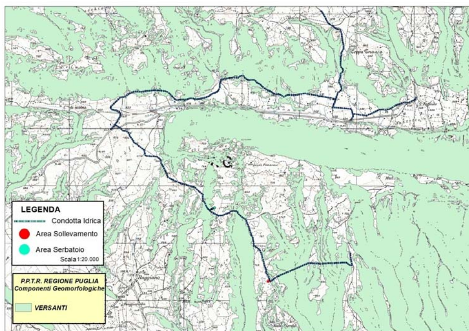
Componenti geomorfologiche interessate: Versanti
