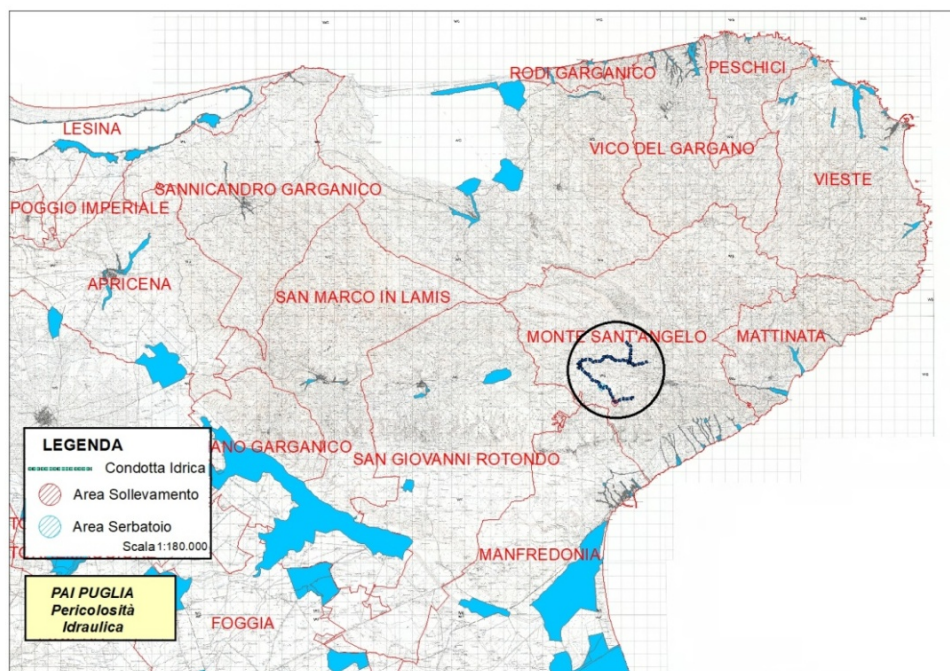
Pericolosità Idraulica
