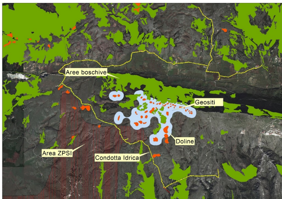
Stralcio planimetrico su base ortofoto con individuazione della condotta idrica interferente con l'area ZPSI, in adiacenza a Geositi, Doline ed aree boschive.
