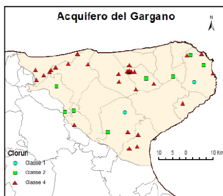
Distribuzione dei Cloruri
