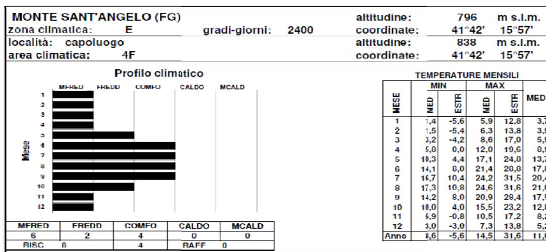
Profilo Climatico di Monte Sant'Angelo
