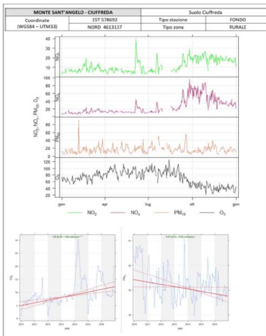
Emissioni complessive rilevate dalla centralina di monitoraggio in Monte Sant'Angelo (2010-2017)
