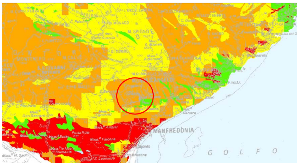
Carta di vulnerabilità intrinseca o naturale dell'acquifero
