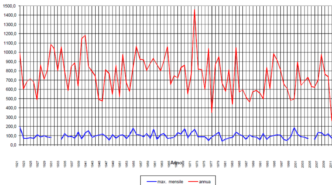
Dati pluviometrici stazione di Monte Sant'Angelo (FG)
