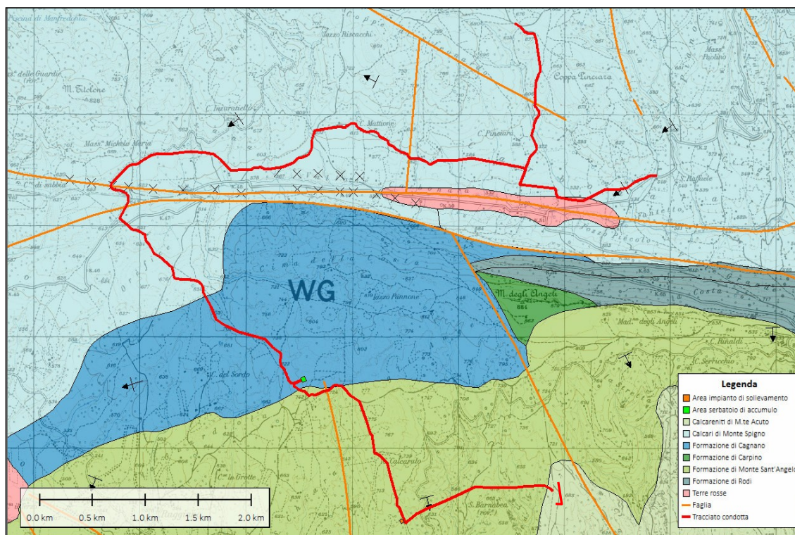
Stralcio della carta geologica con indicazione del tracciato della condotta idrica
