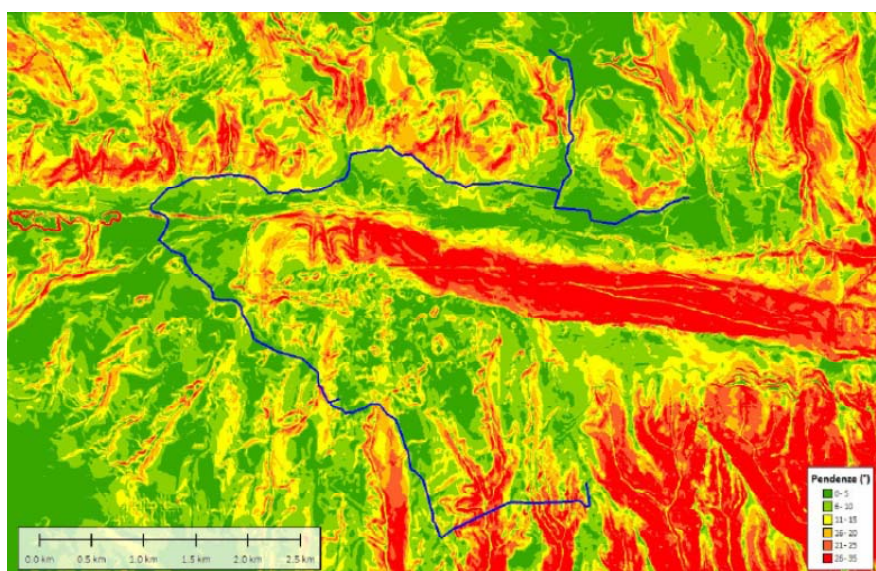
Carta delle pendenze dell'area
