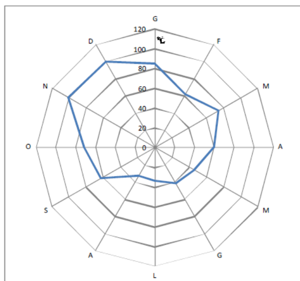
Precipitazioni medie mensili in mm
