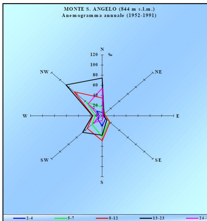
Anemogramma annuale della stazione di Monte Sant'Angelo (1952-91)
