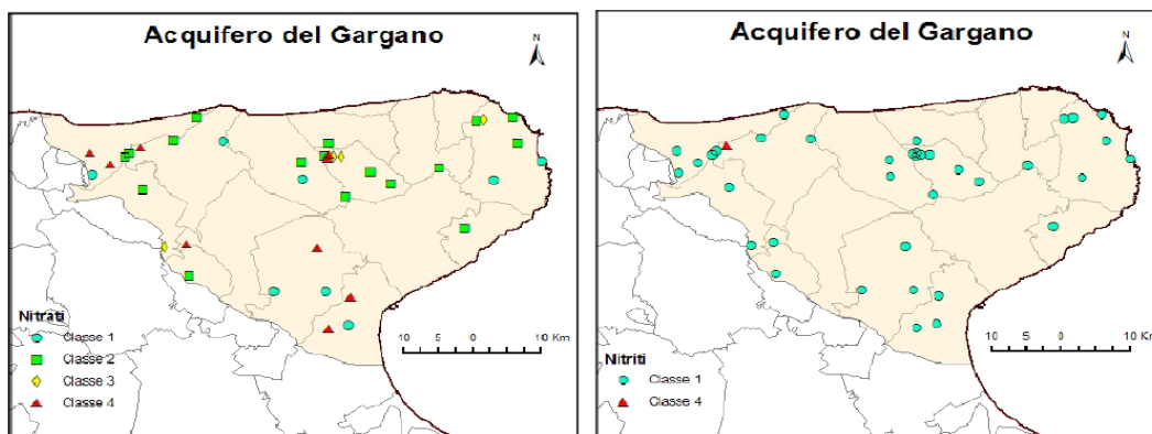
Distribuzione dei Nitrati e dei Nitriti
