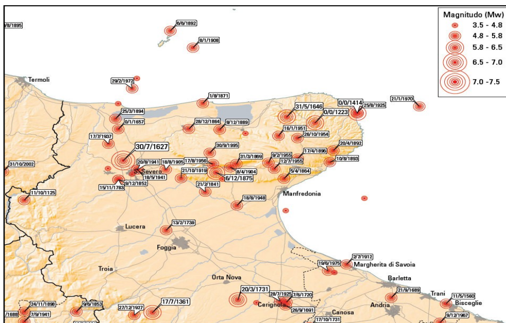
Carta della distribuzione epicentrale dei terremoti storici della provincia di Foggia.
