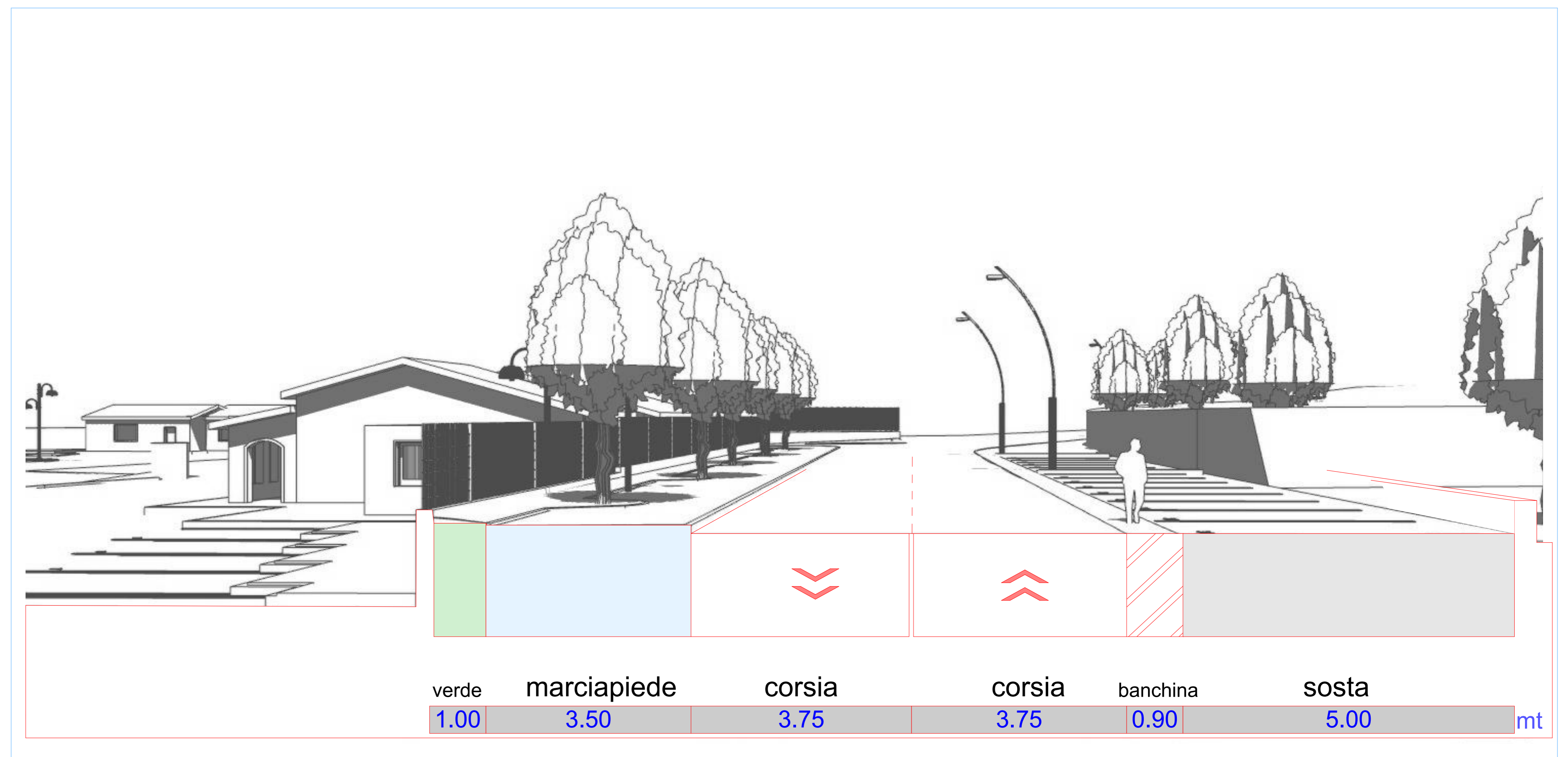
B - B Sezione prospettica
