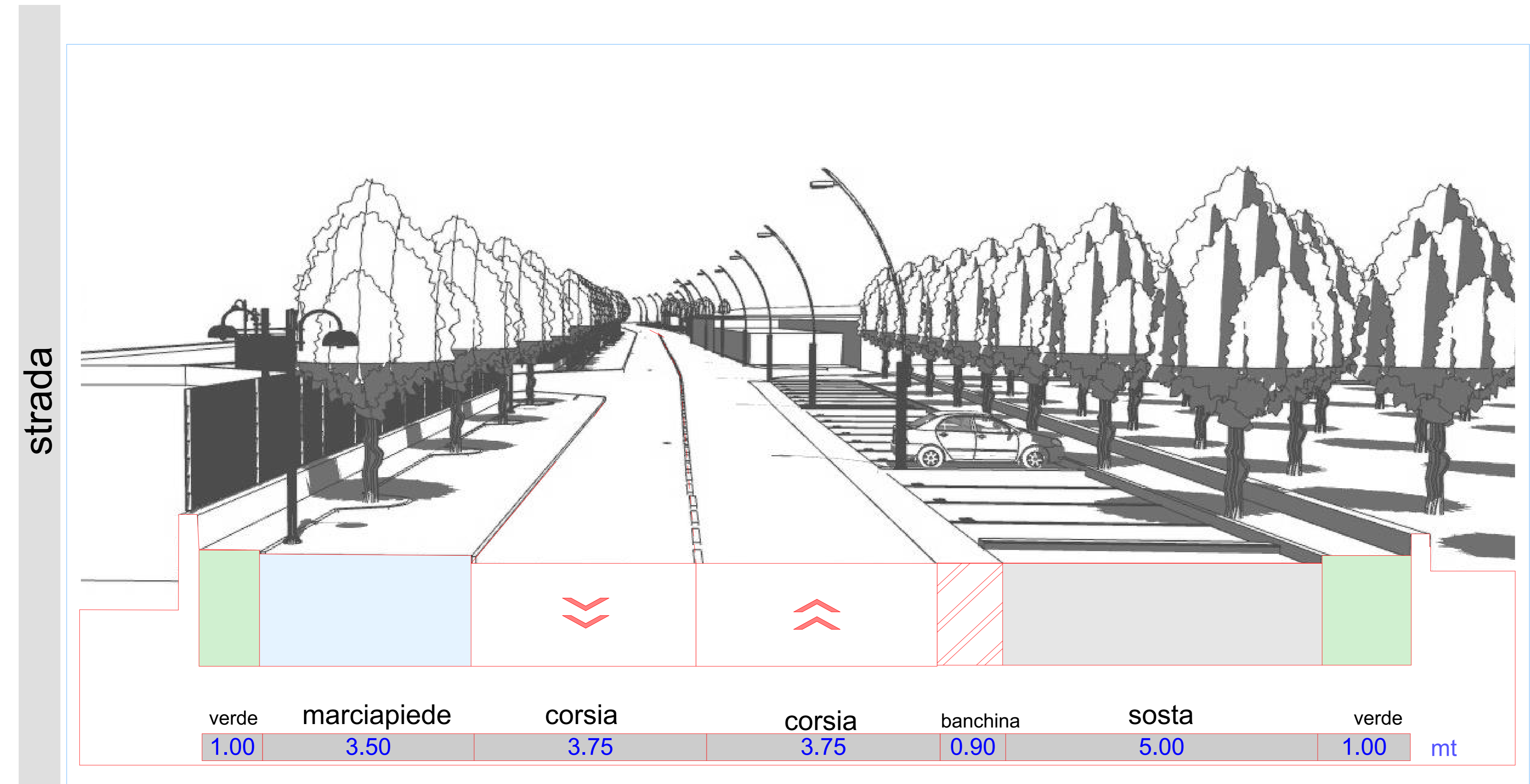
A-A Sezione prospettica
