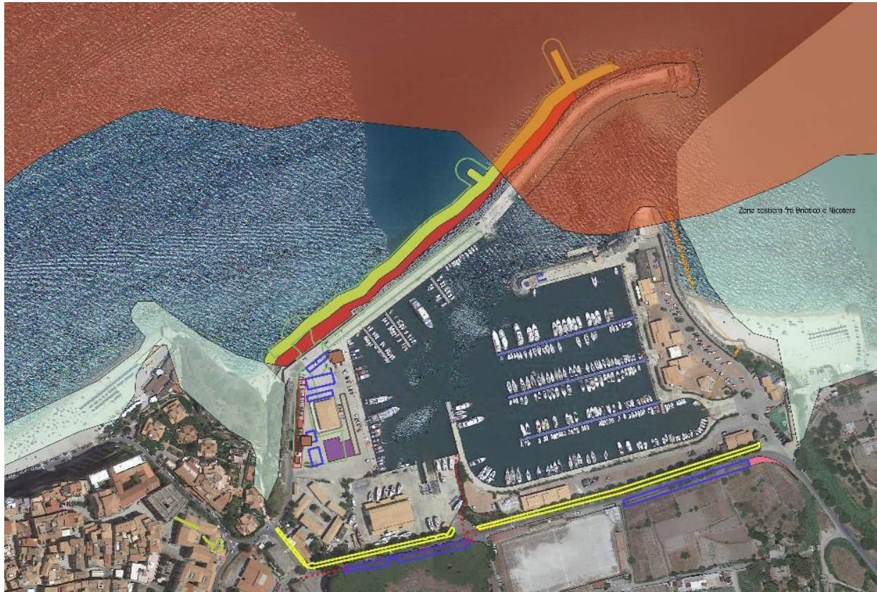
Figura 33: Planimetria delle opere rispetto alle aree protette
