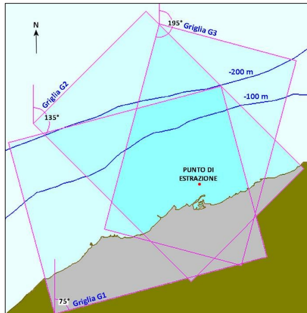
Figura 13: Griglie di calcolo del modello NSW.
