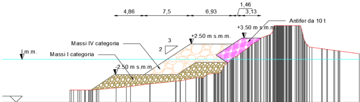
Figura 23: sezione composta per il tratto compreso fra la sezione 10 e la sezione 20
