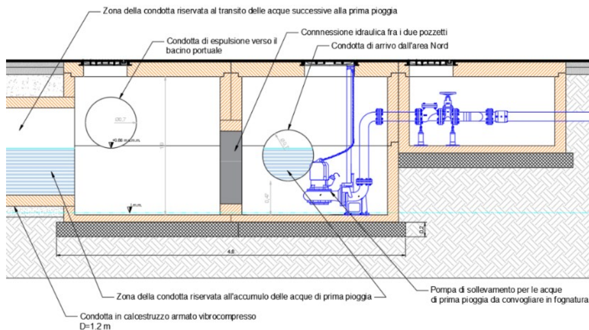
Figura 32 – Sezione trasversale del pozzetto di smistamento.
