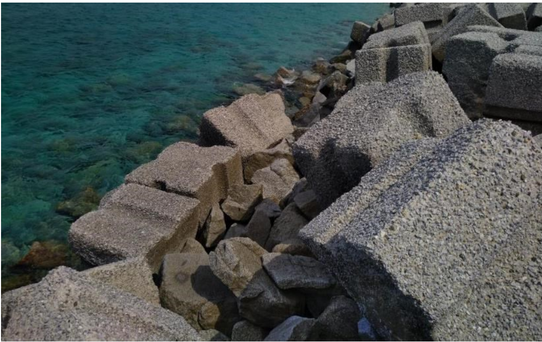
Figura 5: Vista dei dissesti al piede della mantellata.
