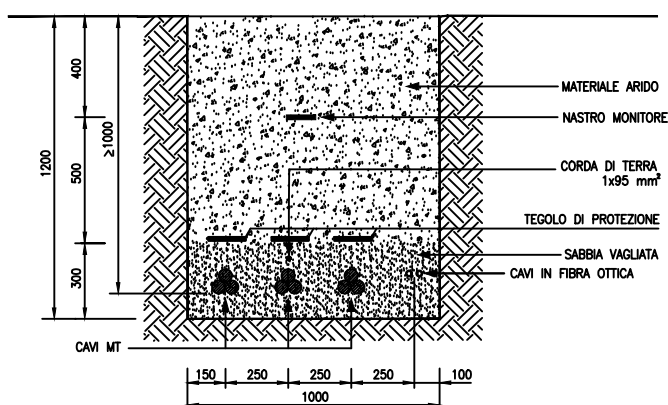
SEZIONE DI POSA "3" POSA SU STRADA STERRATA O TERRENO VEGETALE
