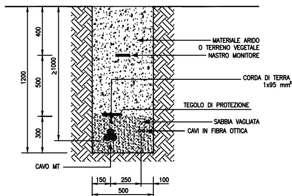
SEZIONE DI POSA "3" POSA SU STRADA STERRATA O TERRENO VEGETALE
