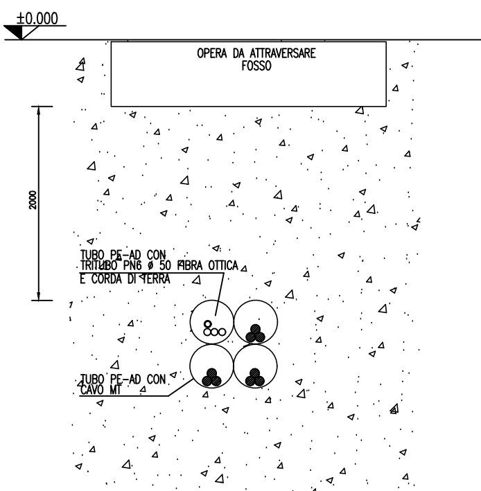
SEZIONE DI POSA "4" POSA IN TUBO CON SPINGITUBO
