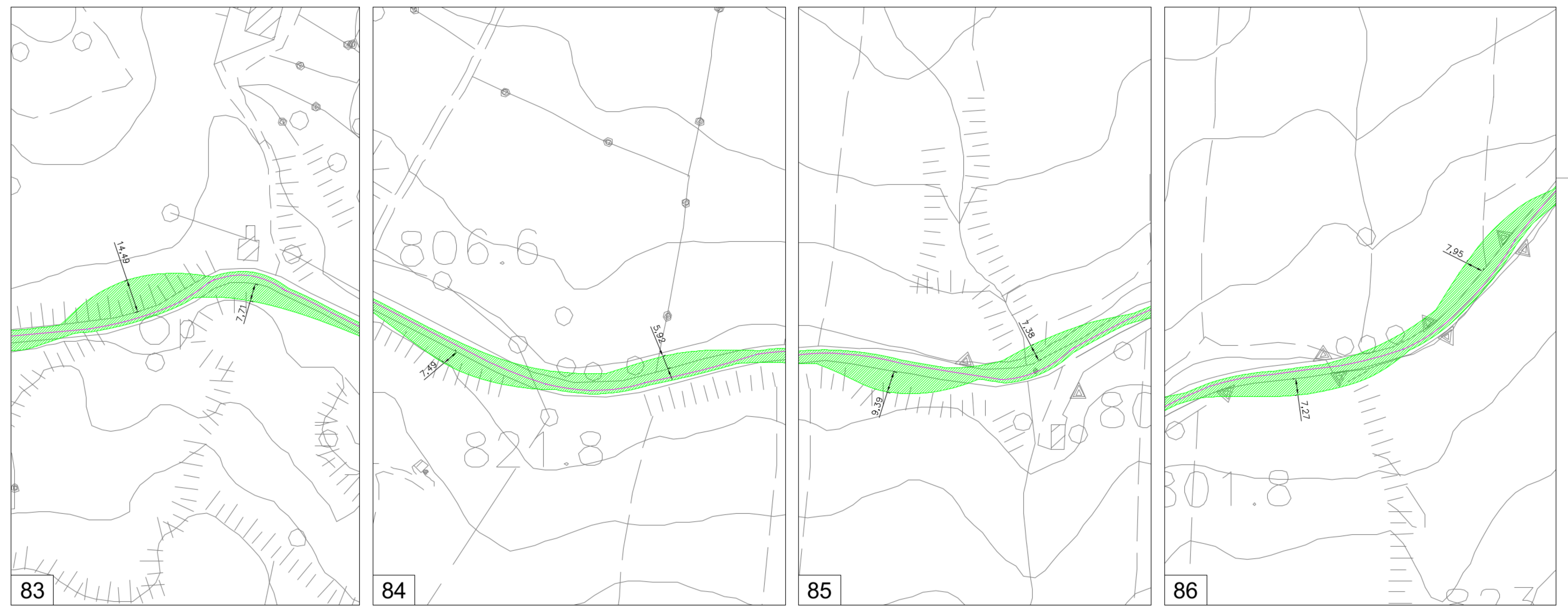
PERCORSO SCLAFANI - INGRANDIMENTI scala 1: 100
