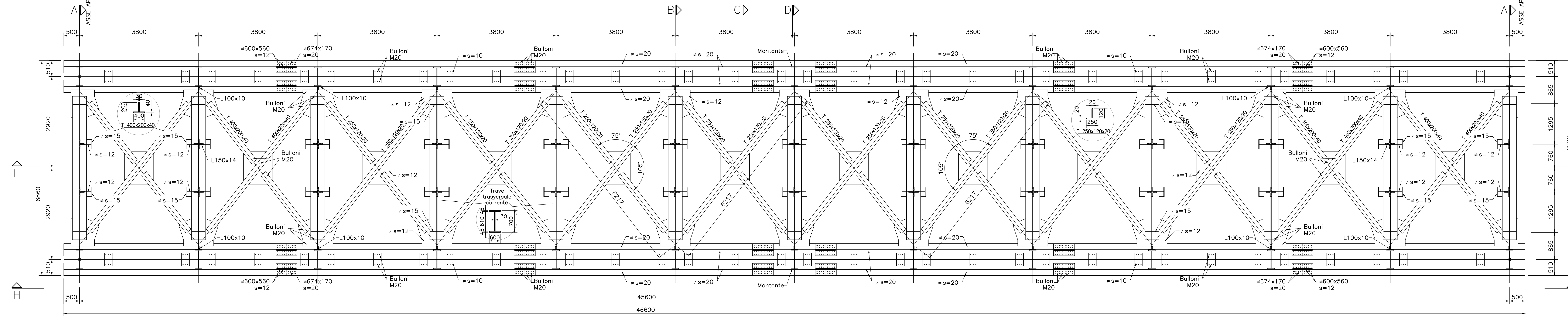
PIANTA "G" SCALA 1:50
