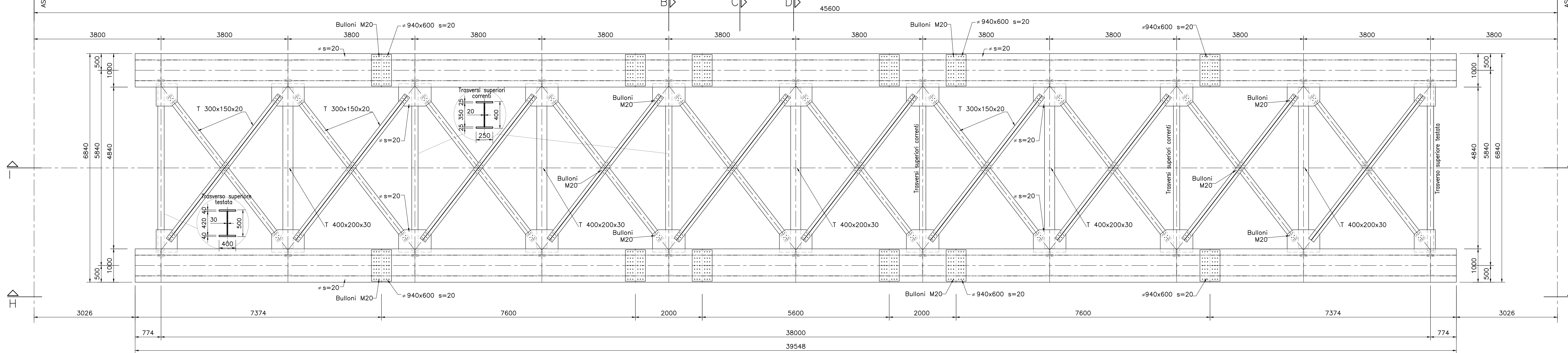
PIANTA "E" SCALA 1:50
