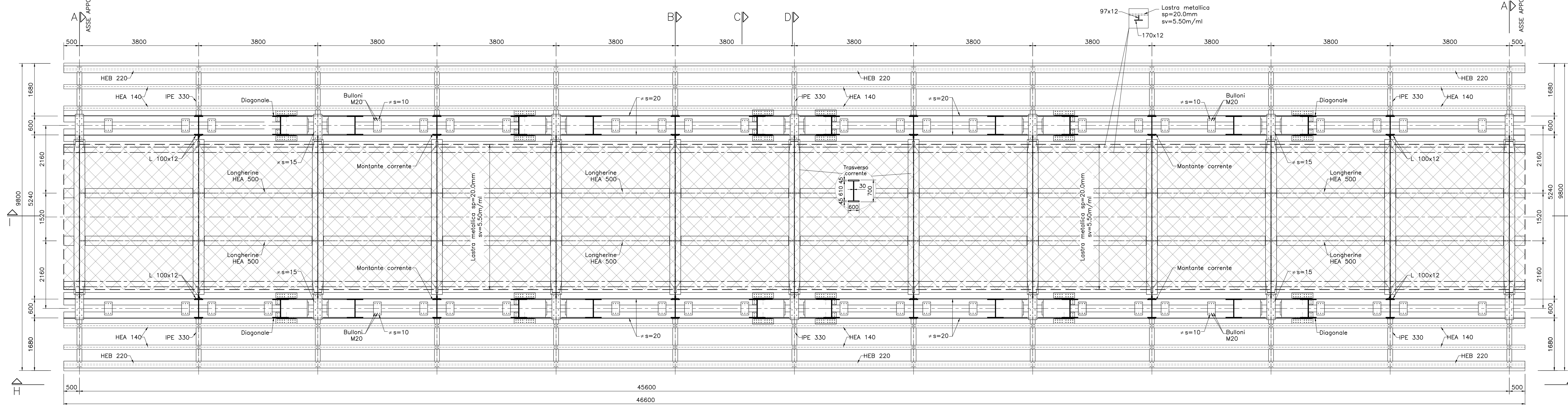
PIANTA "F" SCALA 1:50
