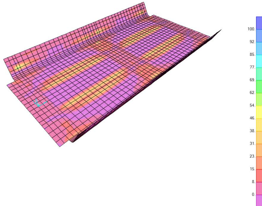
Figura 8_ Sollecitazioni SLU su vasca portaballast tensioni trasversali
