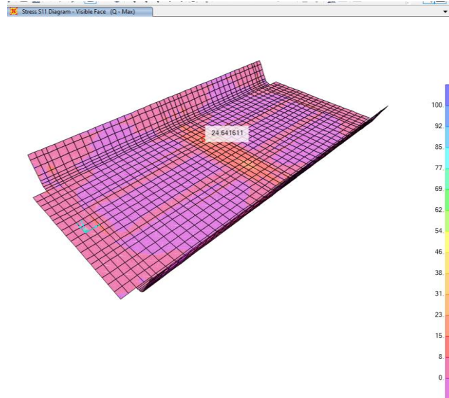
Figura 10: Sollecitazione a fatica su vasca porta ballast tensioni longitudinali
