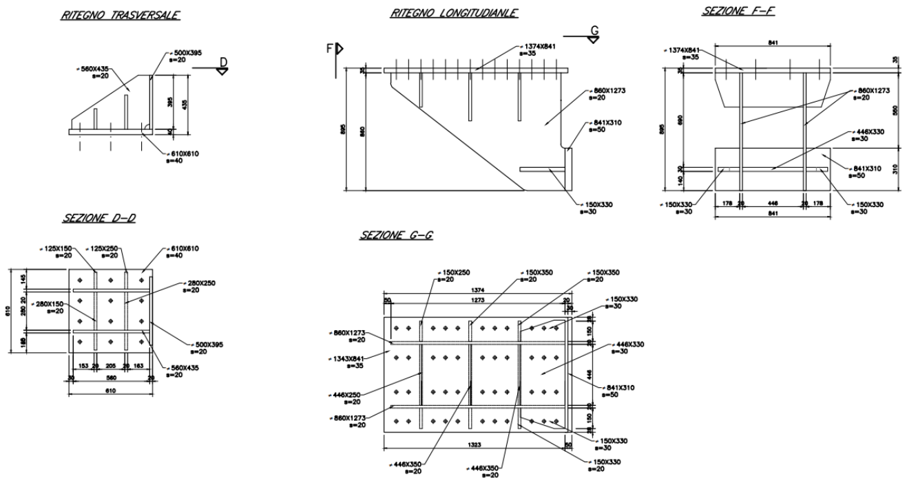
Figura 19: Dettaglio Ritegno sismico
