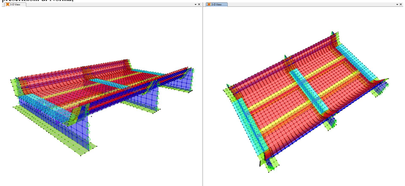
Figura 5: Verifica locale della vasca porta ballast
