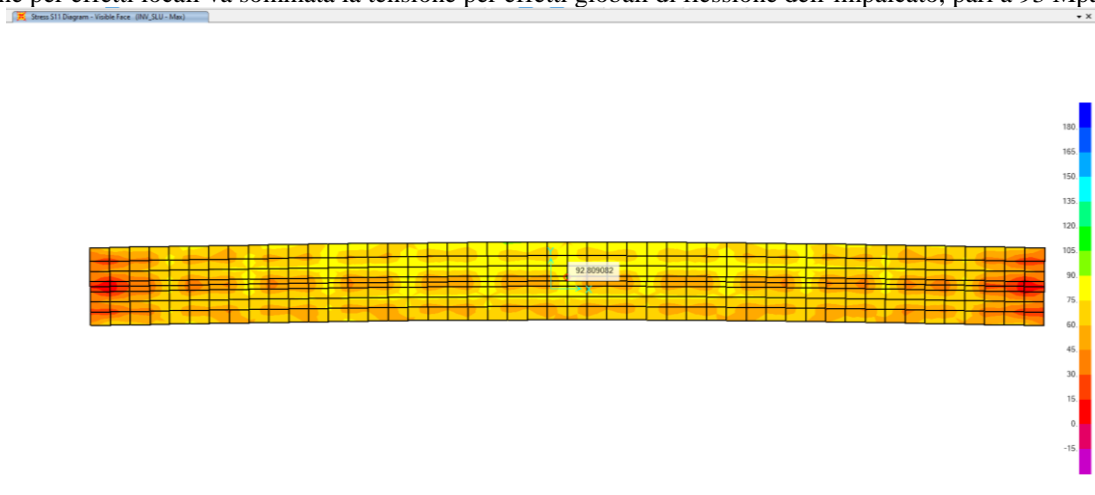
Figura 9: Sollecitazioni SLU su vasca portaballast modello globale
