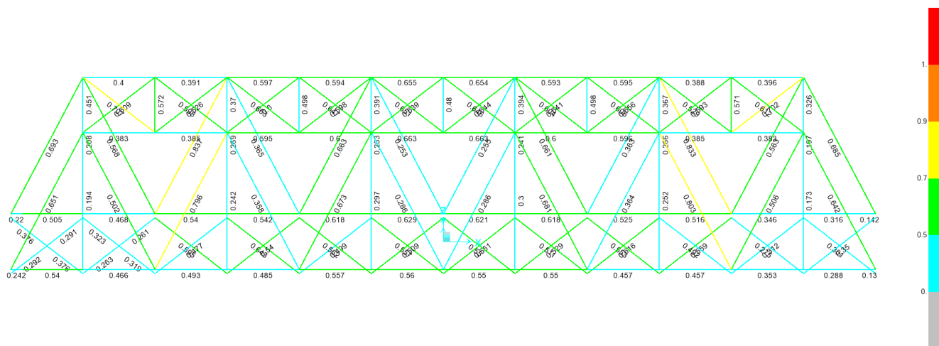
Figura 15_ Verifica di resistenza valida per elementi di parete e controventi (modello globale)
