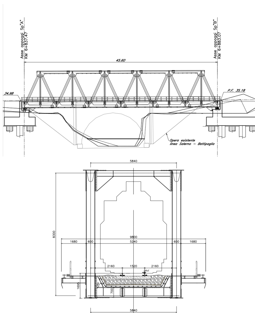
Figura 1_Prospetto e sezione trasv.
