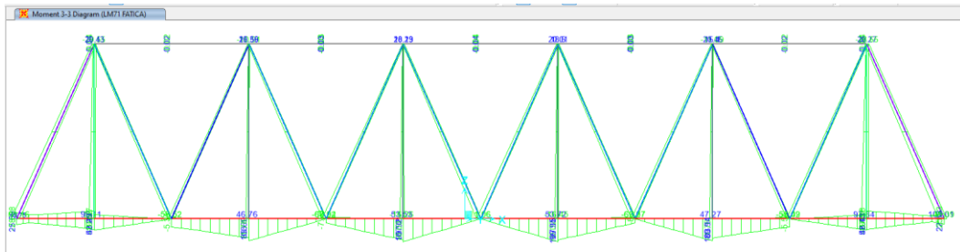
Figura 16_Sollecitazioni flettenti FATICA
