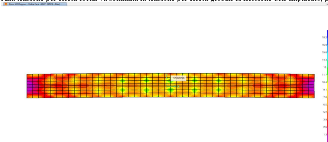
Figura 11: Sollecitazioni a fatica su vasca modello globale
