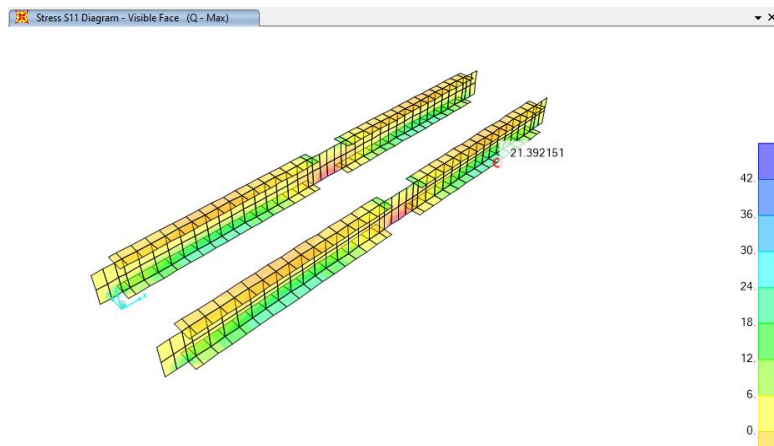
Figura 13: Sollecitazioni a fatica su longherina
