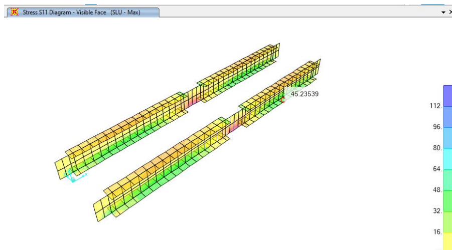
Figura 12: Sollecitazioni SLU su longherina
