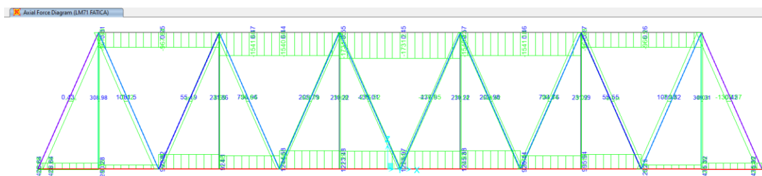
Figura 17_Sforzo assiale FATICA
