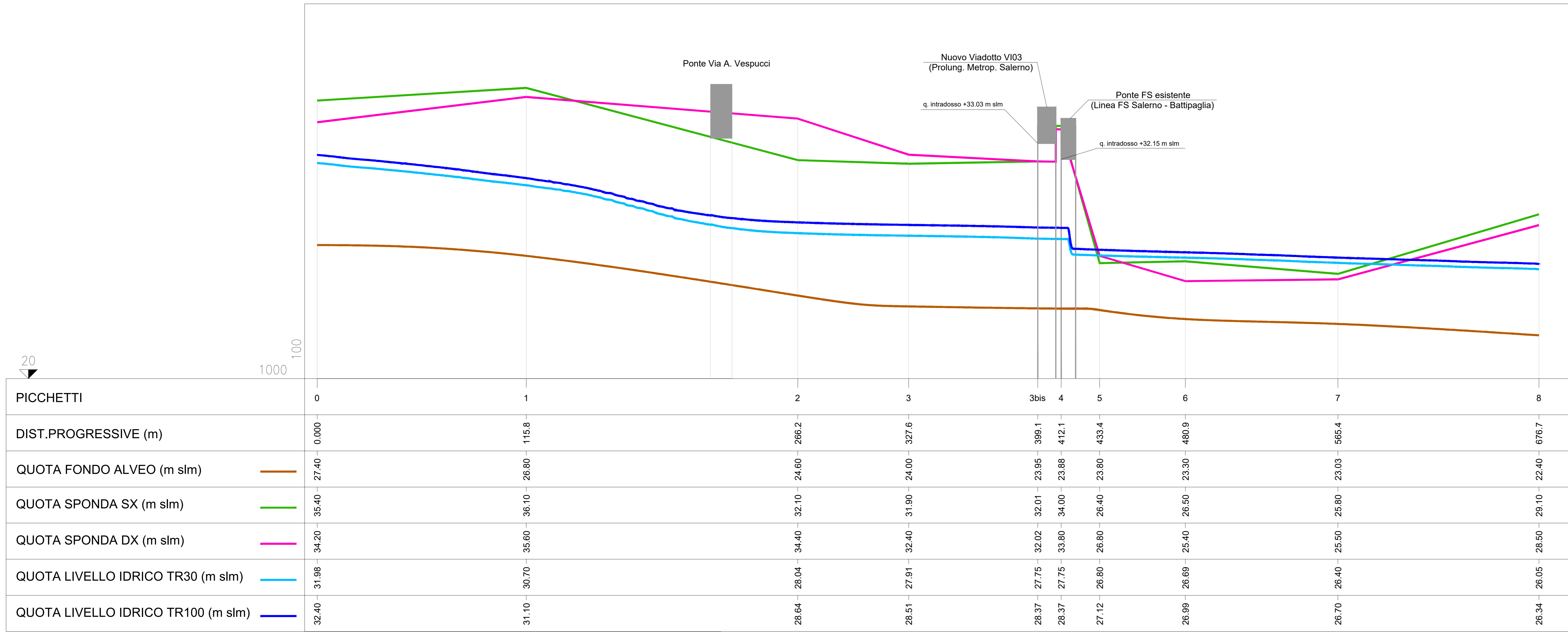
Profili di rigurgito Tr = 30 e 100 anni - post operam (scala 1:100/1:1000)
