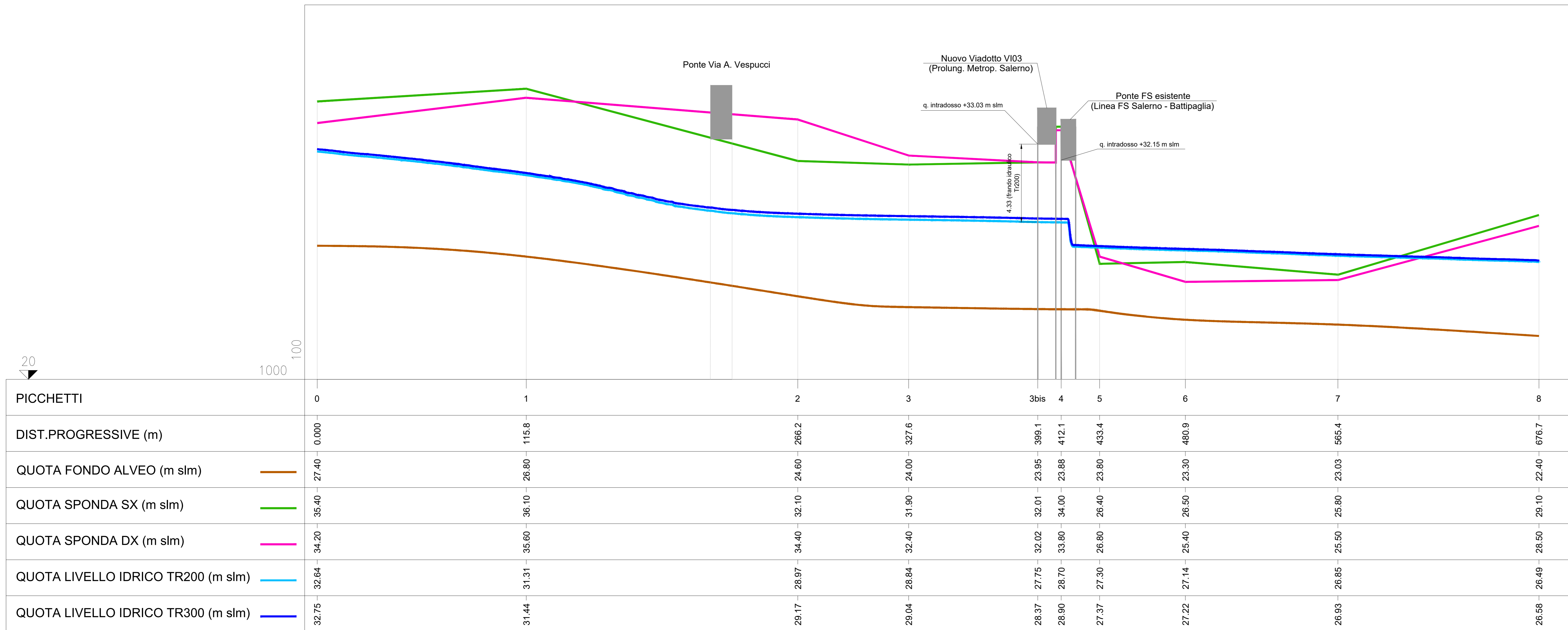
Profili di rigurgito Tr = 200 e 300 anni - post operam (scala 1:100/1:1000)
