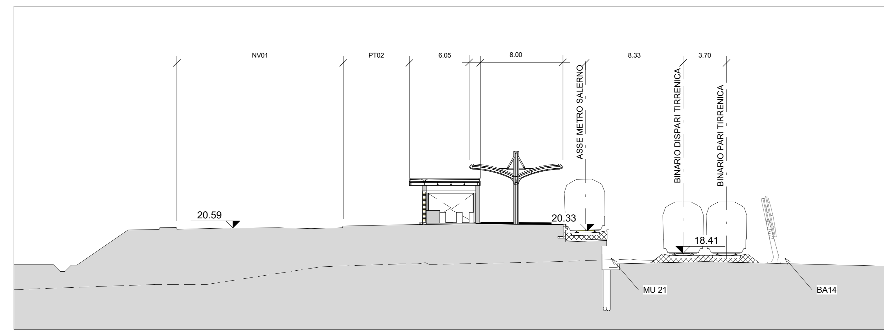
Sez. P1 Post Operam
