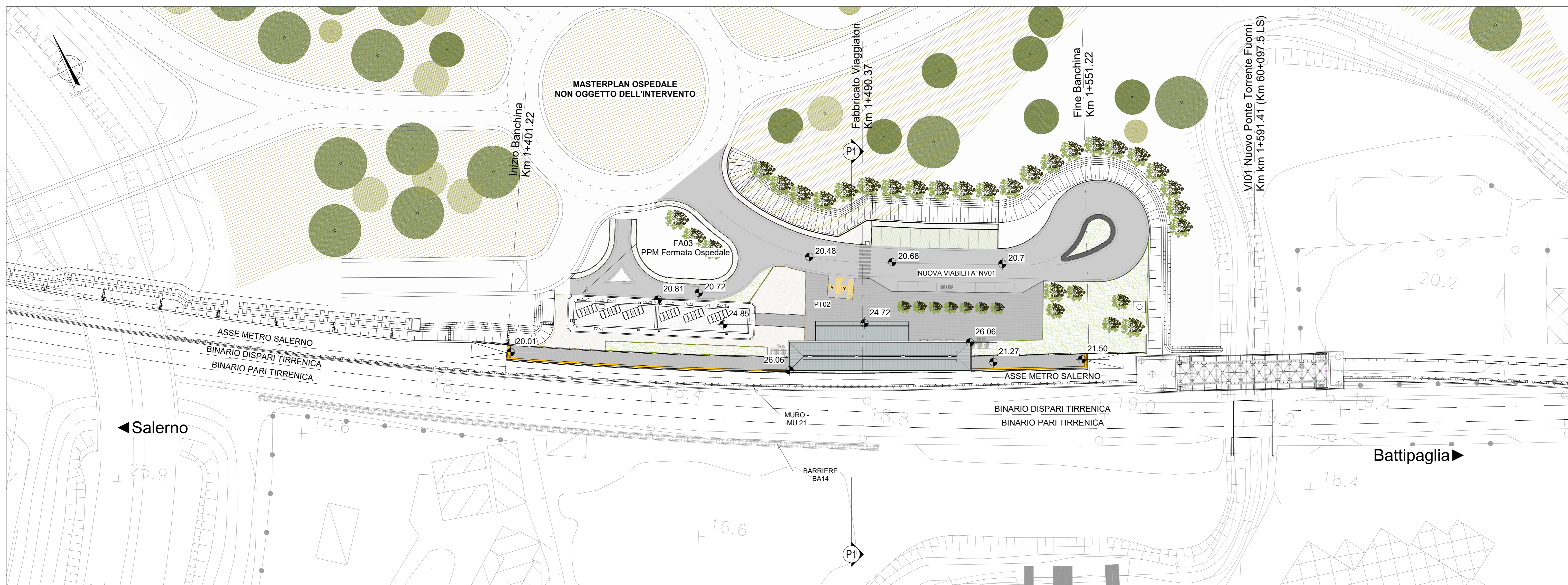
Planimetria Generale - Post Operam
