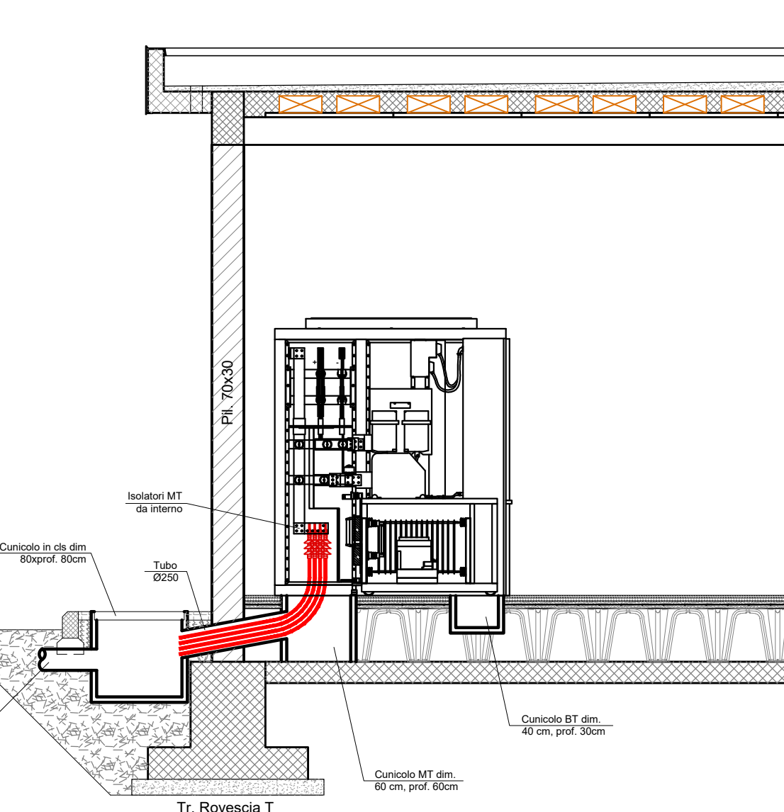
SEZIONE D. (Scala 1:50)
