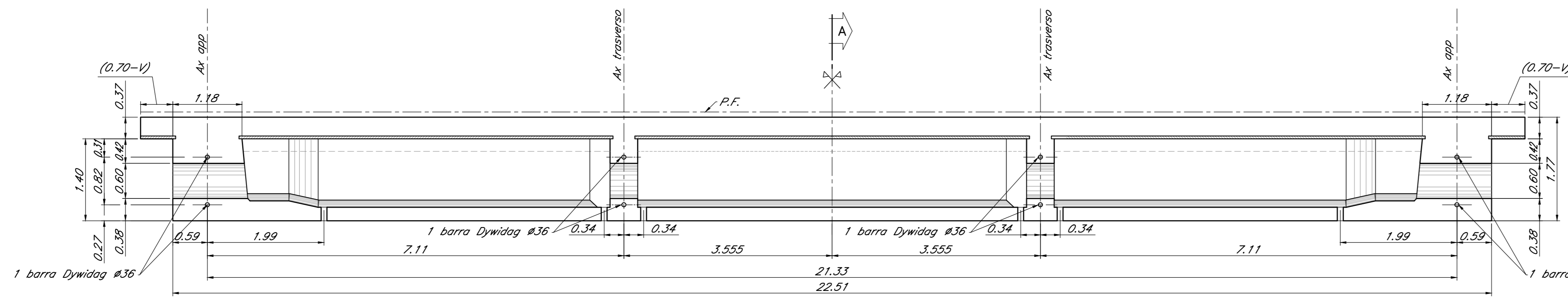
Sezione longitudinale "B" Scala 1:50
