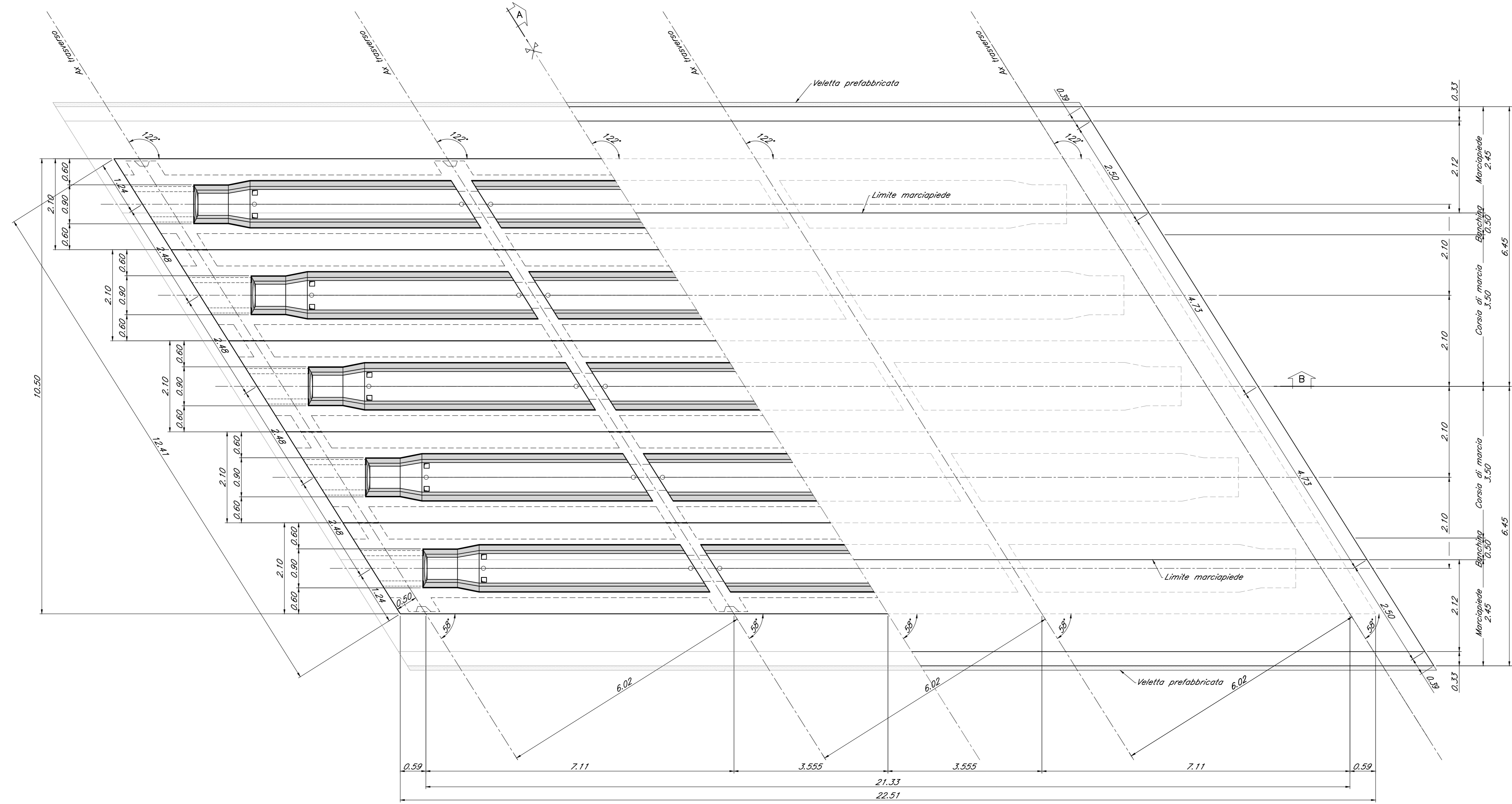
Sezione longitudinale "B" Scala 1:50
