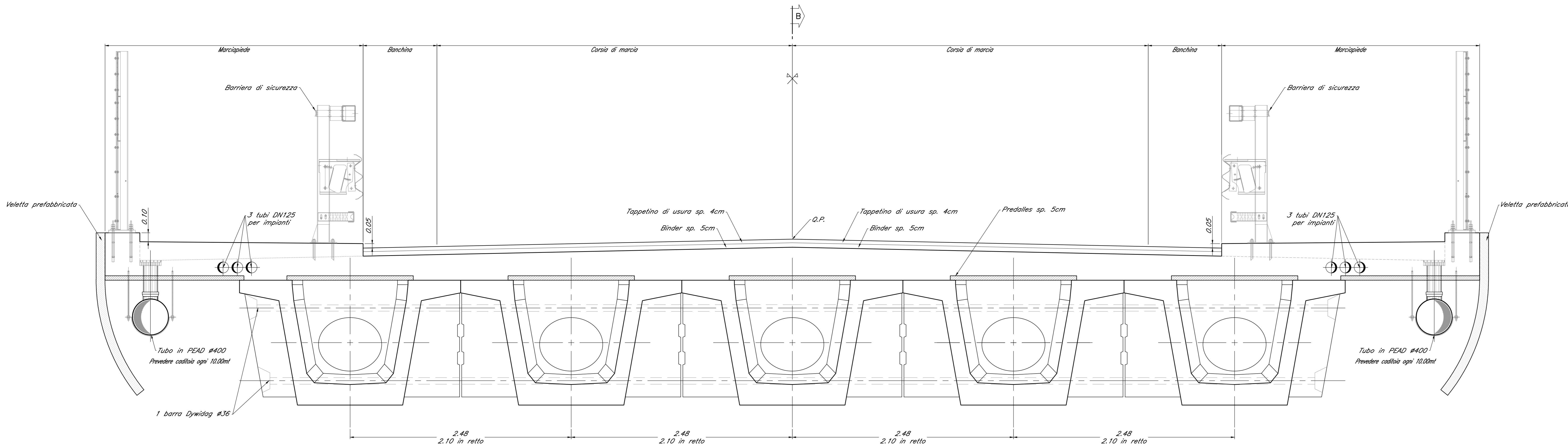
Sezione "A" Scala 1:20
